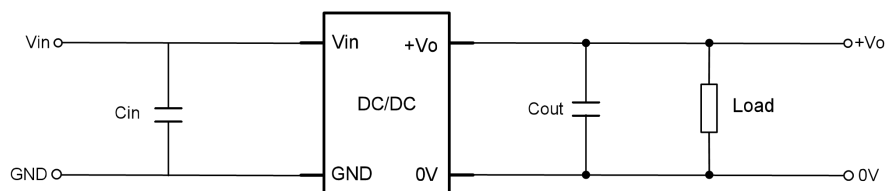
图 1 应用电路图
