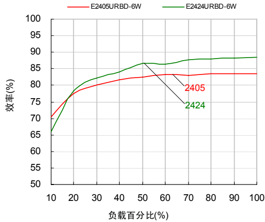
效率与负载关系曲线图
