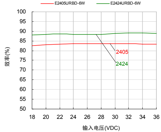
效率与输入电压关系曲线图
