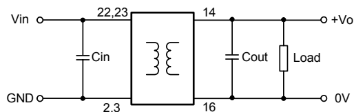
图 1 应用电路图
