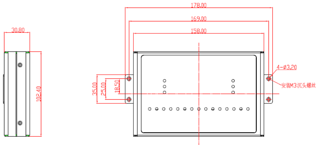
图 1.1 机械尺寸
