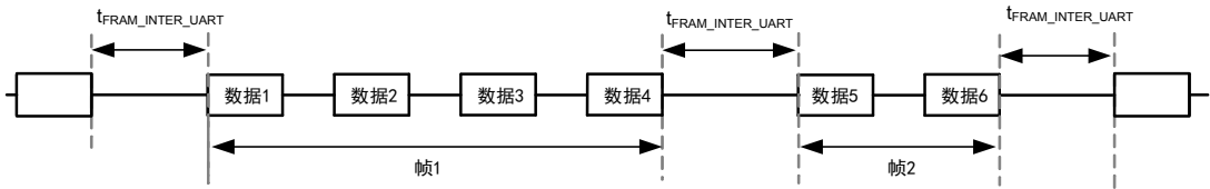
图 2 UART 帧间隔
