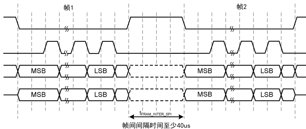
图 3 SPI 帧间隔
