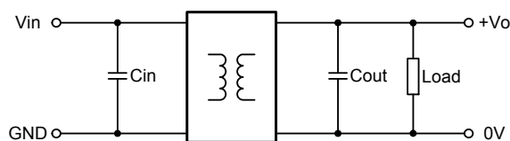
图 1 应用电路图
