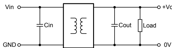
图 1 应用电路图
