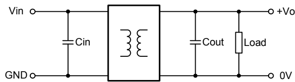
图 1 应用电路图
