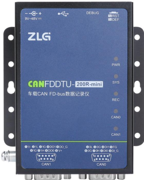
图 3.1 面板布局
