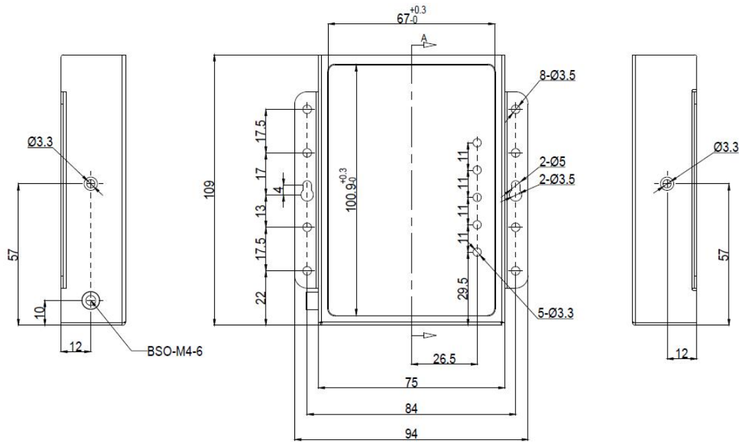
图 2.1 机械尺寸
