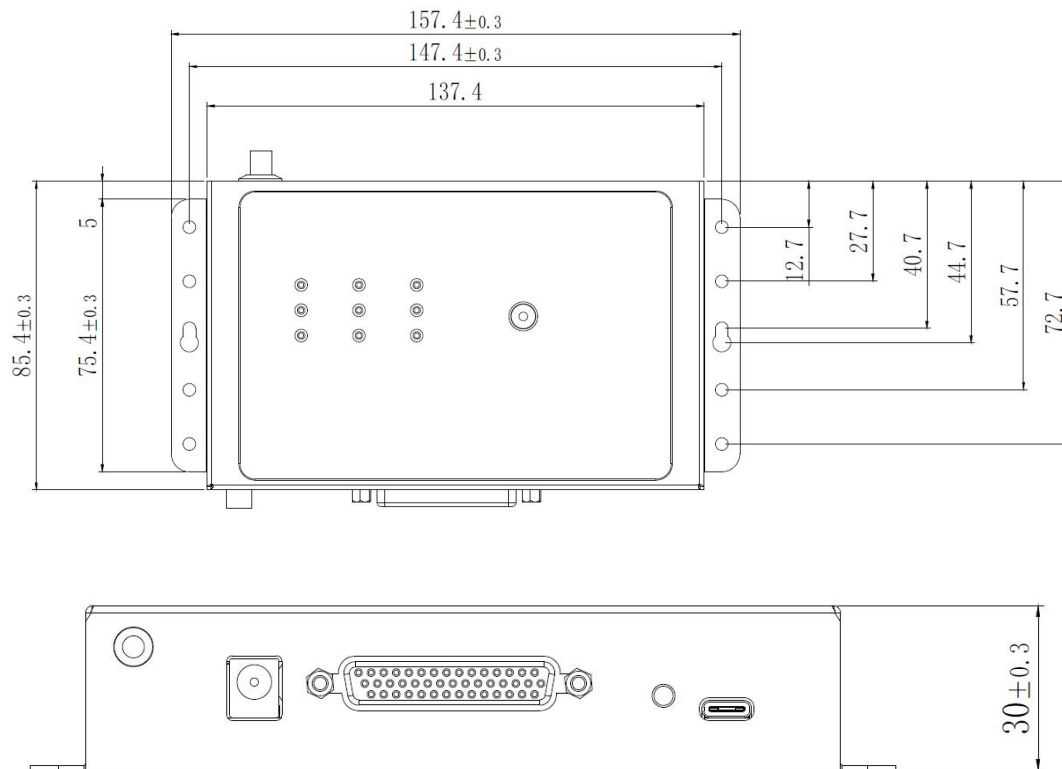
图 3.1 主机尺寸图
