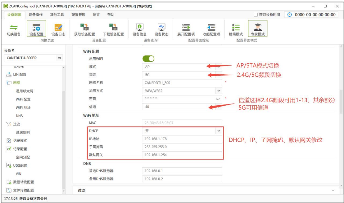
图 4.6 WiFi 配置
