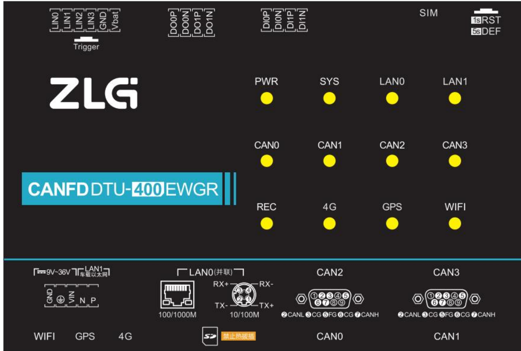
图 4.1 面板布局
