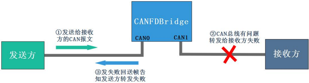
图 6.10 失败回送示意图
