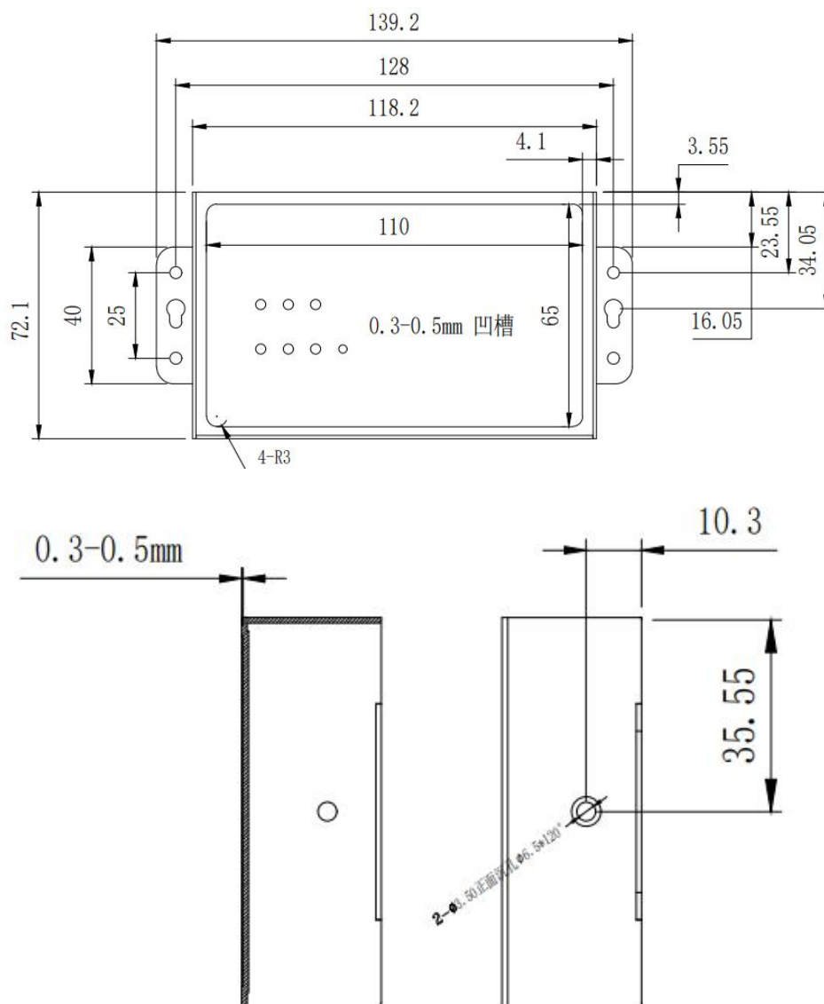
图 3.2 主机尺寸图二
