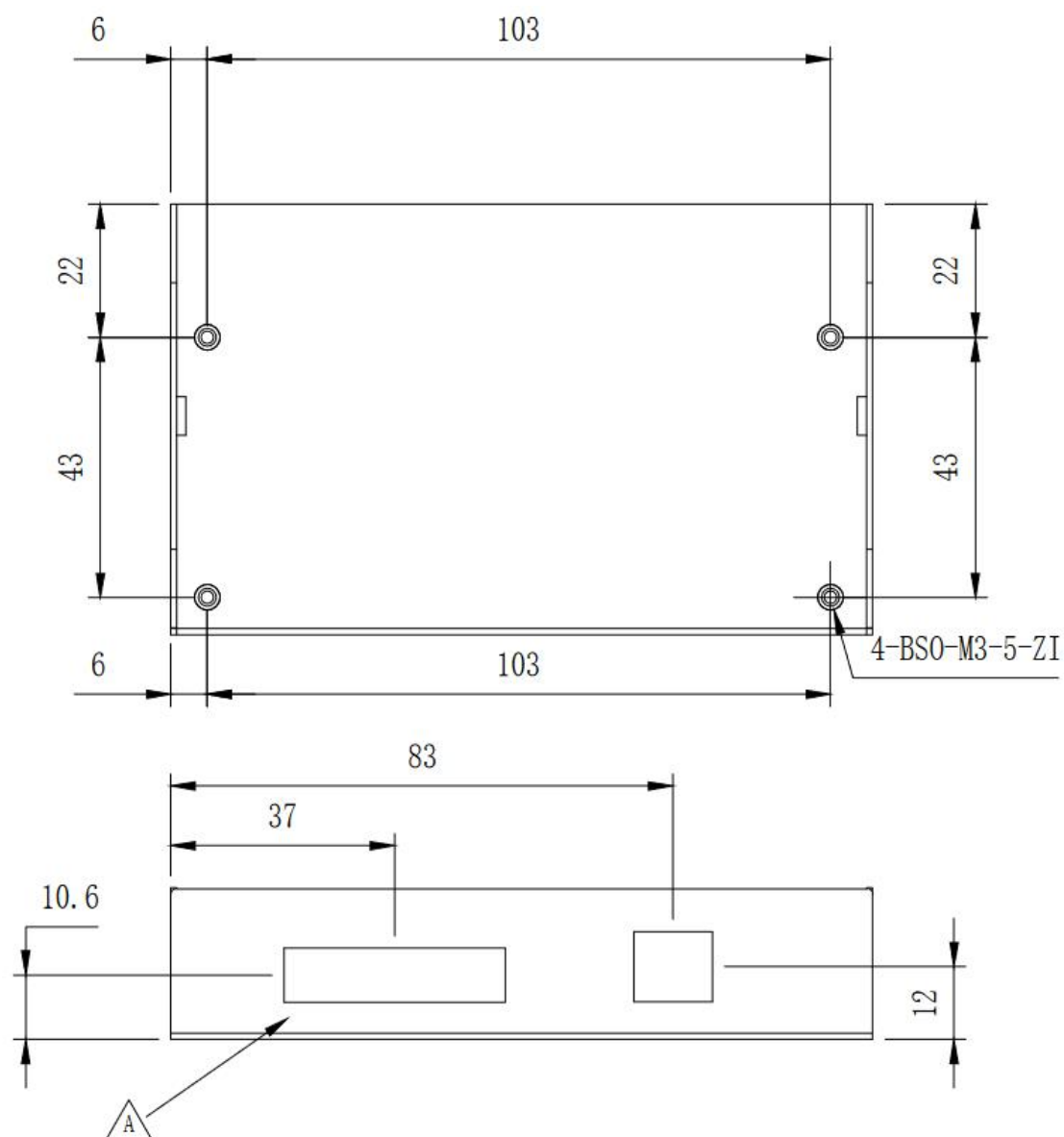
图 3.1 主机尺寸图一
