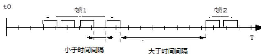
图 1.1 串行帧时间格式（透明带标识转换）
