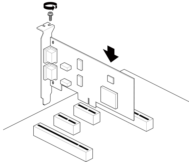
图 2.9 PCIeCANFD-800U 系列 CAN 接口卡拔插示意图
