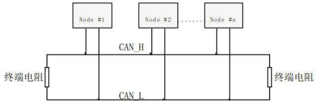
图 2.5 CAN-bus/CAN(FD)-bus 网络直线拓扑结构
