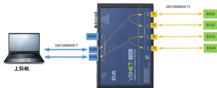
图 3.15 网络划分
