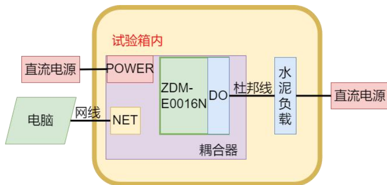
图 2 试验配置框图
