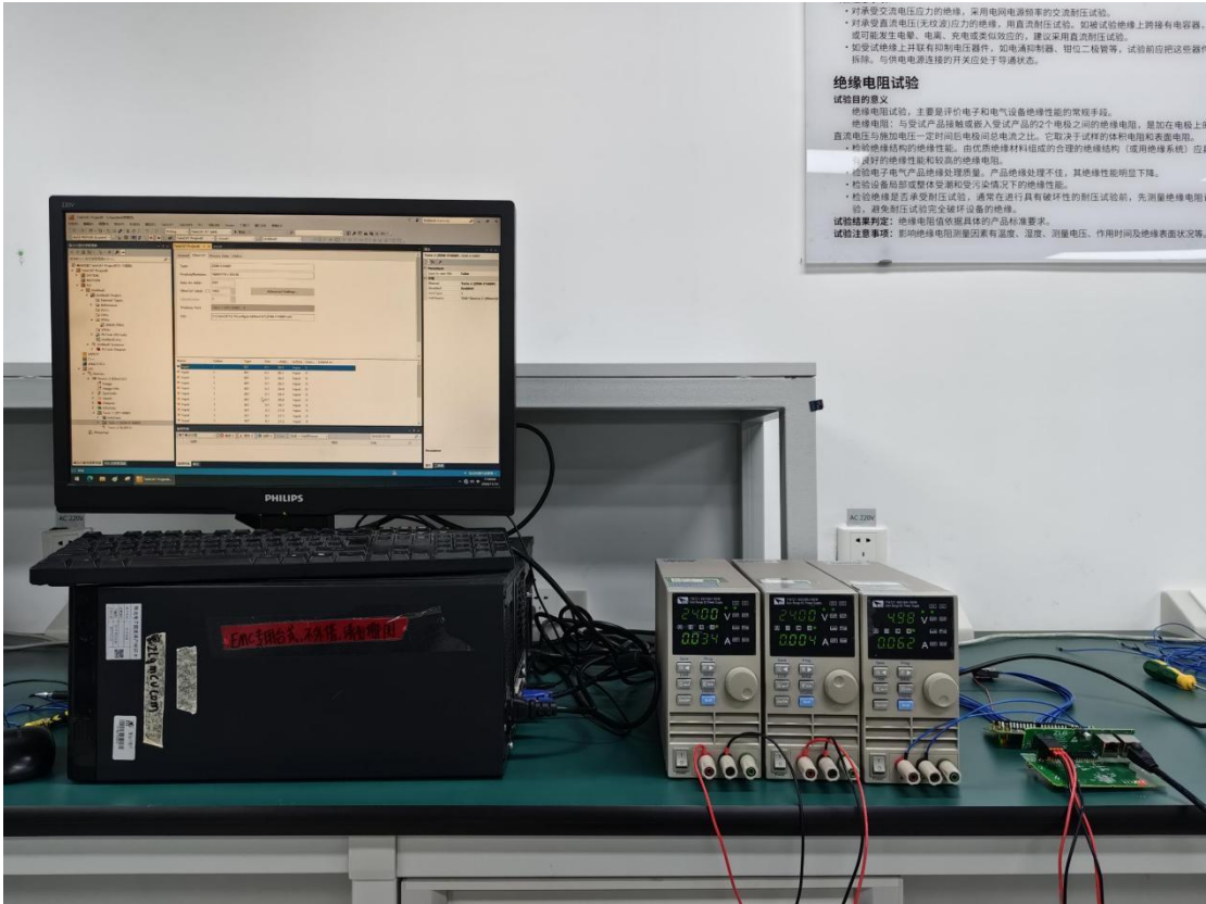
图 1 电源输入试验连接
