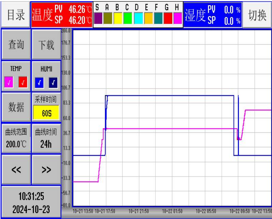
图 7 湿热处理曲线图
