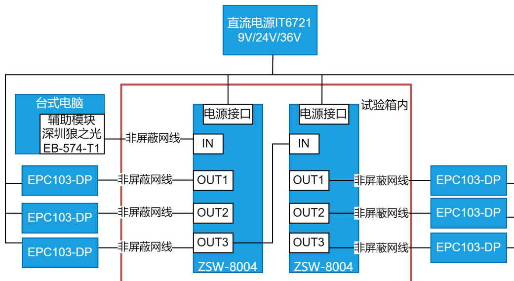
图 2 试验配置框图
