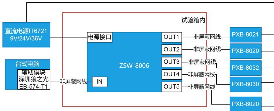
图 2 试验配置框图
