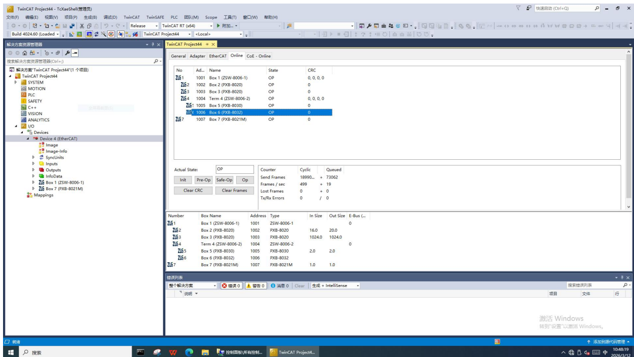
图 14 样机在恒定湿热试验时第三次启动运行检查功能正常(36V)
