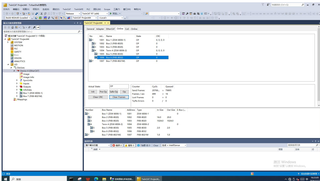
图 8 样机在低温试验时第三次启动运行检查功能正常(24V)
