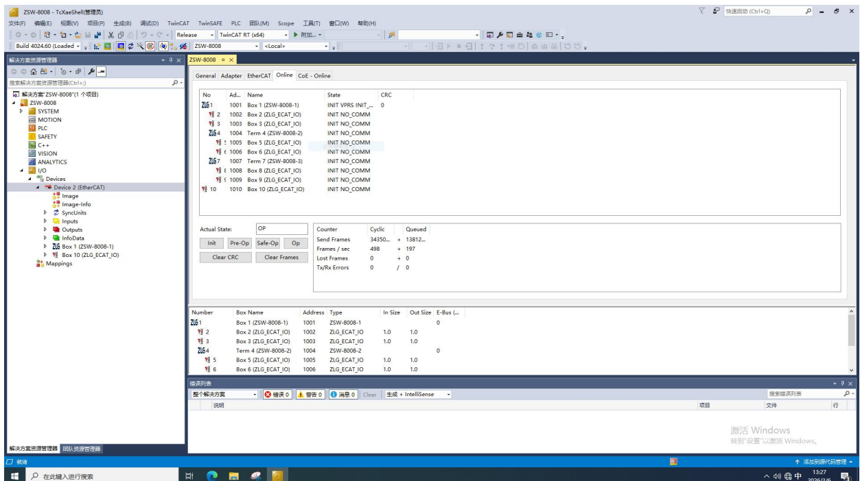
图 9 样机在低温试验第二次检查功能正常（供电 24VDC）
