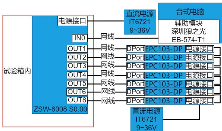
图 2 试验配置框图
