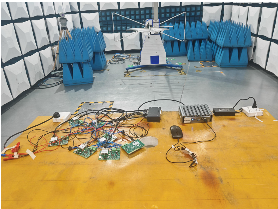
图 8 辐射骚扰试验现场配置图
