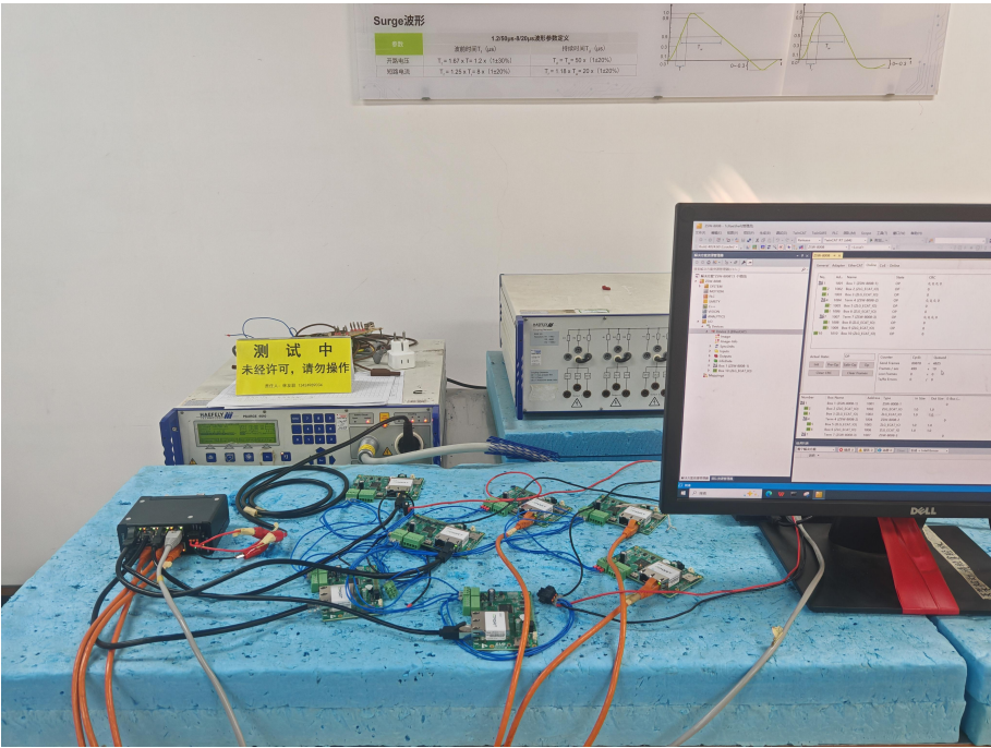
图 5 浪涌试验现场配置图
