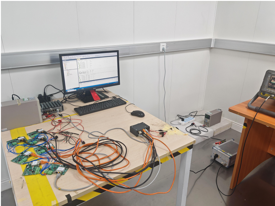
图 7 传导骚扰试验现场配置图
