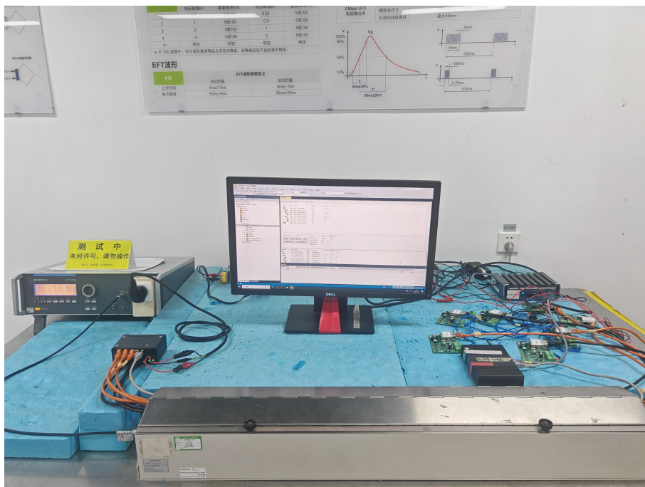
图 4 EFT 试验现场配置图
