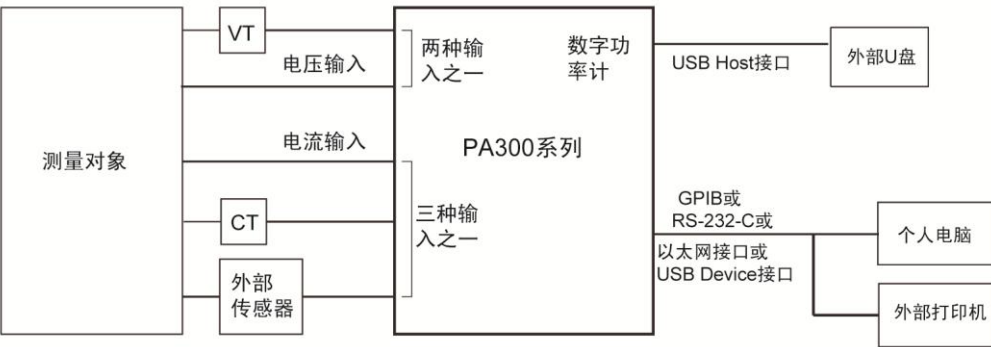
图 1.5 应用系统示意图
