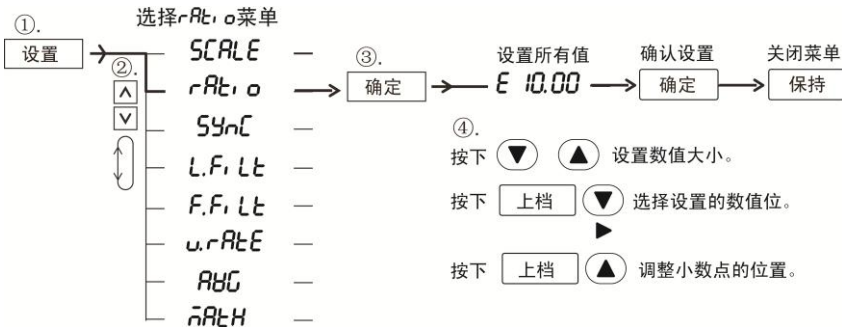
图 6.22 外部电压型电流传感器的转换比例菜单设置流程
