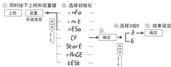
图 6.24 峰值因数选择的菜单操作流程
