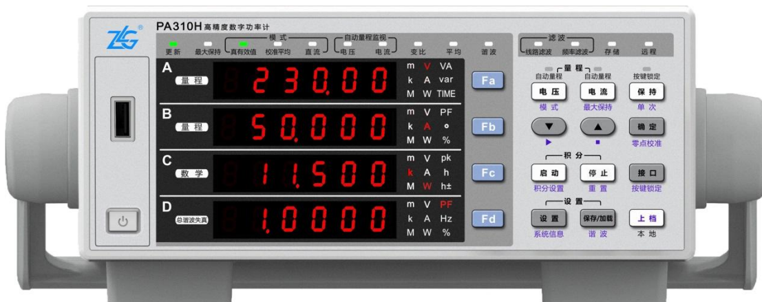
图 1.2 PA300 系列高精度功率计（PA310H 型）
