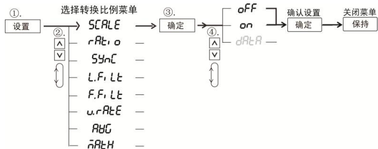
图 6.15 开启/关闭转换比例功能
