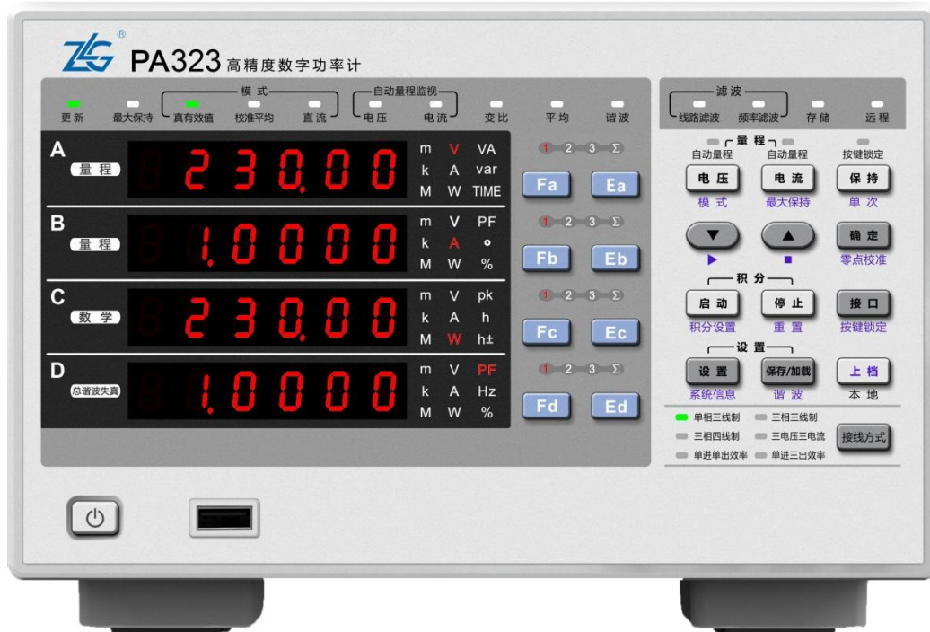
图 1.3 PA300 系列高精度功率计（PA323 型）
