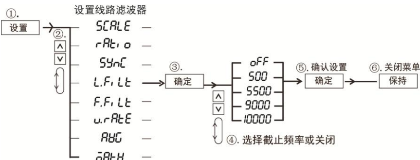
图 6.5 线路滤波器菜单设置流程（PA310/PA310H 型）
