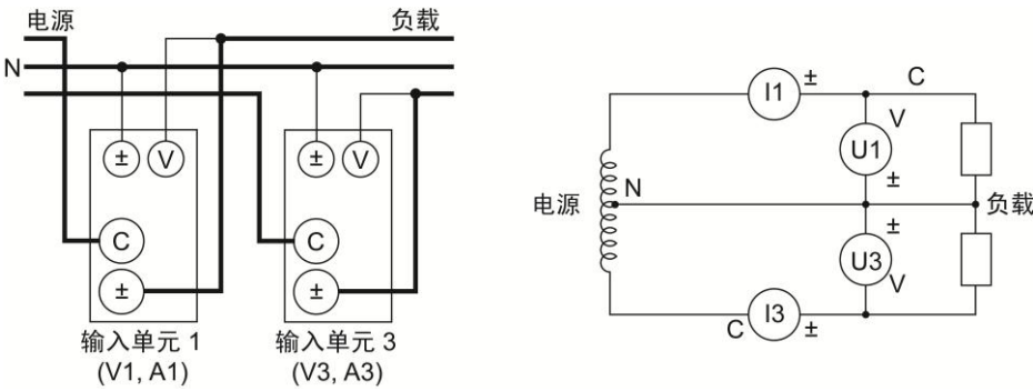
图 4.4 单相三线连接原理图
