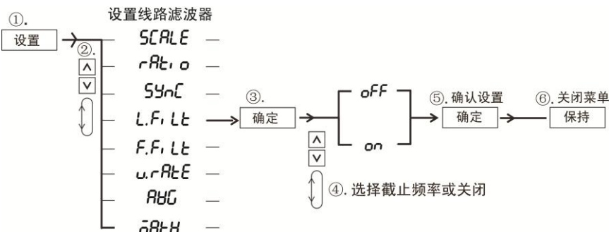
图 6.4 线路滤波器菜单设置流程（PA323/PA333H 型）
