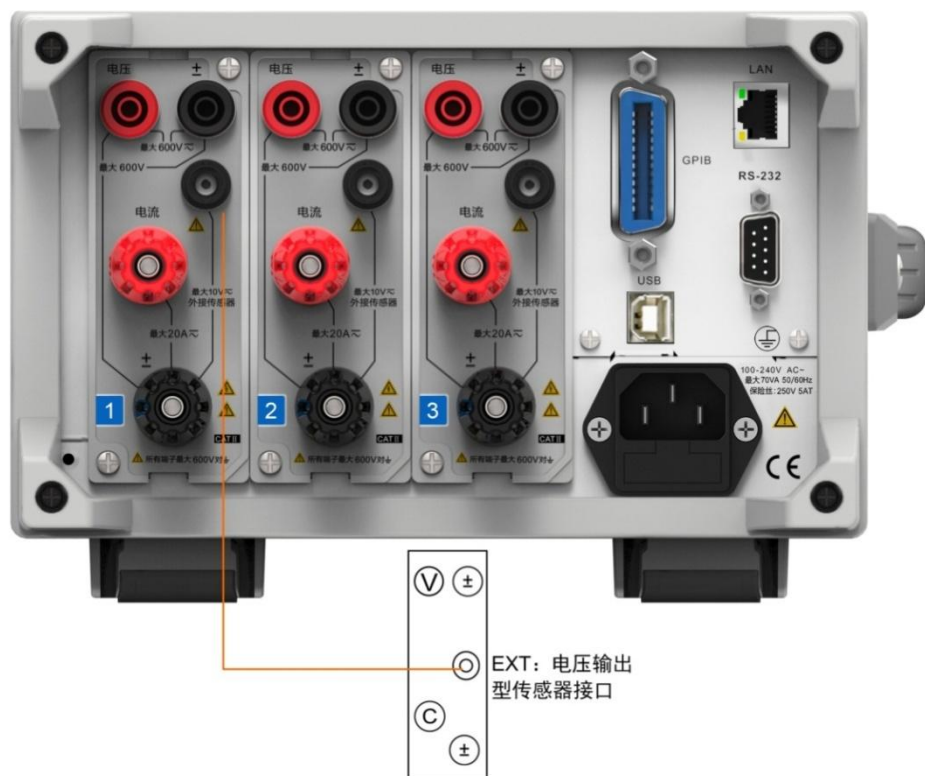
图 4.10 PA323 外部电流传感器端子符号
