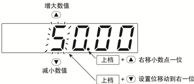
图 3.10 通用键功能说明
