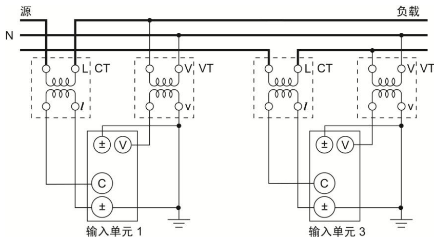
图 4.20 单相三线测量电路
