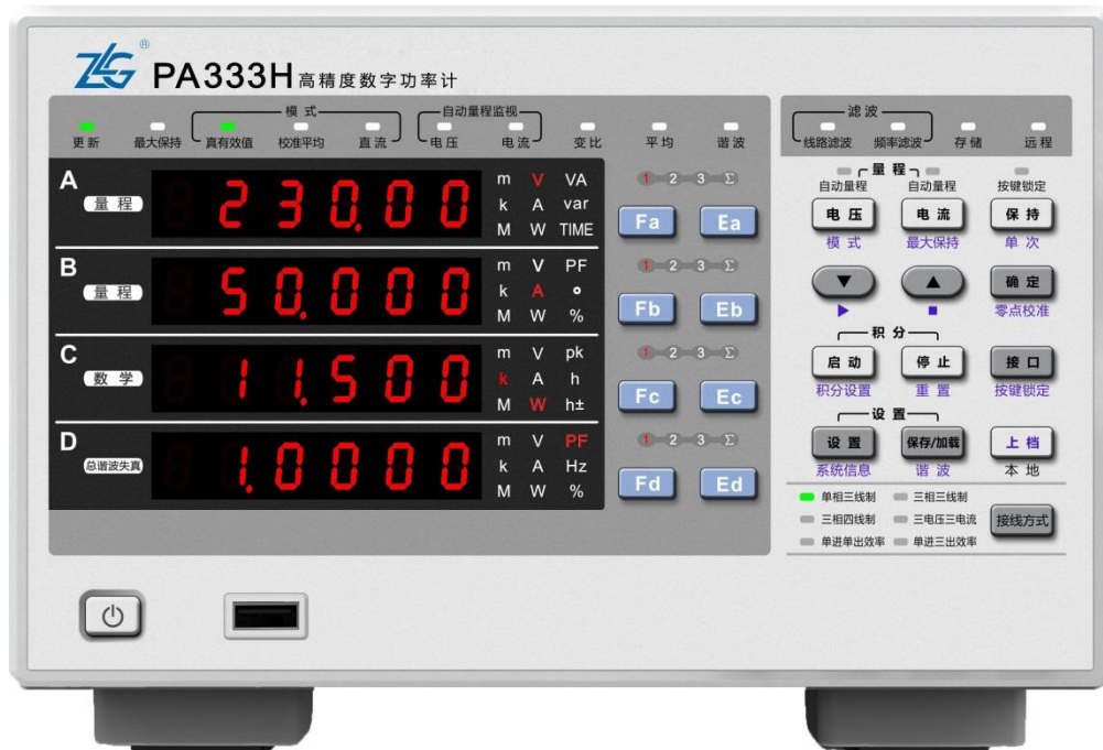
图 1.4 PA300 系列高精度功率计（PA333H 型）
