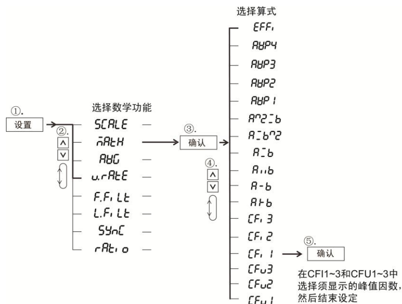
图 6.29 计算峰值因数 (PA323/PA333H 型)
