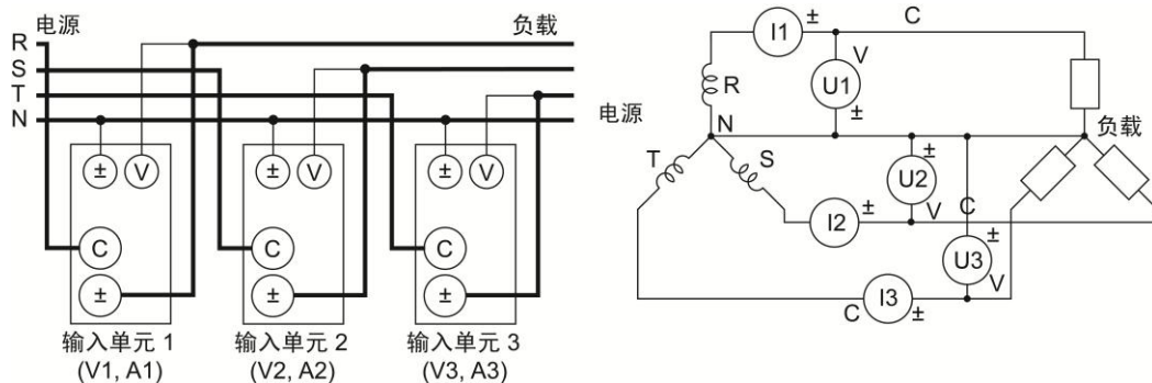
图 4.6 三相四线连接原理图
