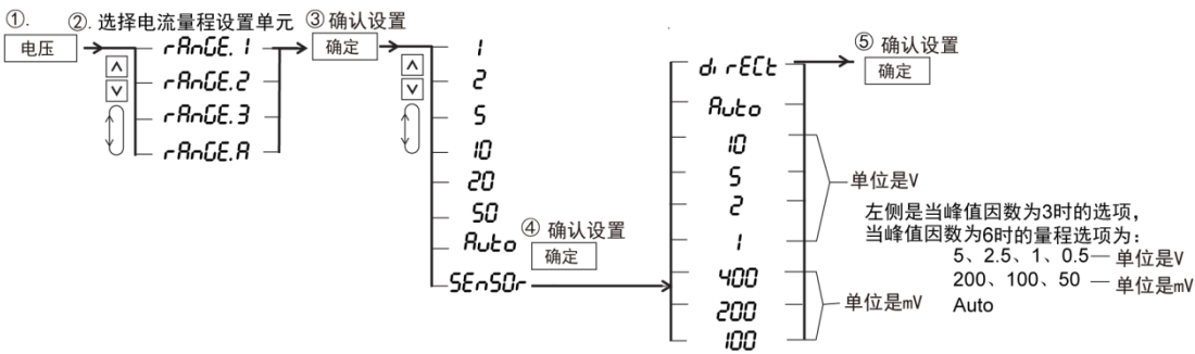
图 6.21 PA333H 型外部电压输出型传感器选择量程示例
