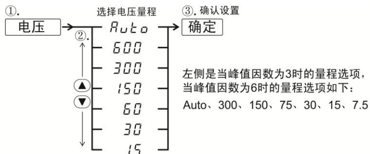
图 6.6 PA310 电压量程选择示例
