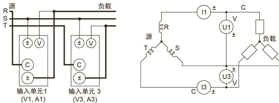
图 4.5 三相三线连接原理图
