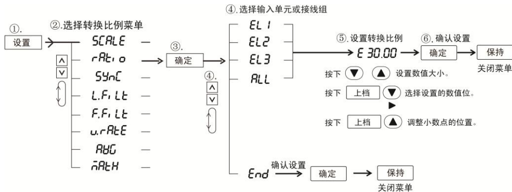
图 6.18 外部电压型电流传感器的转换比例菜单设置流程
