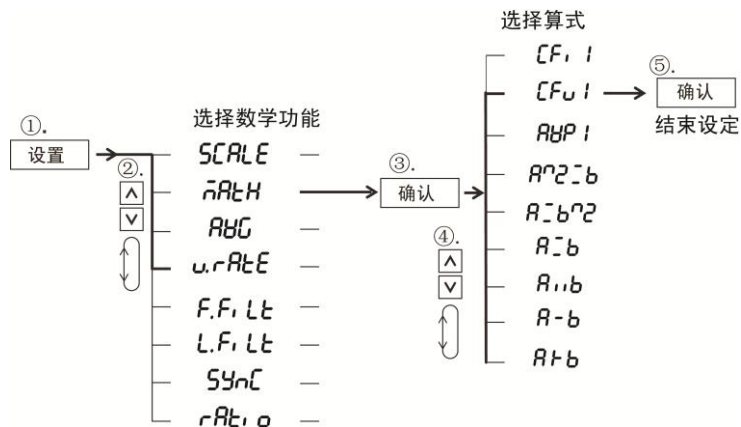
图 6.30 计算峰值因数 (PA310/PA310H 型)
