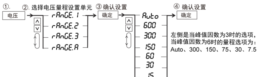
图 6.9 PA323 型功率计电压量程选择示例
