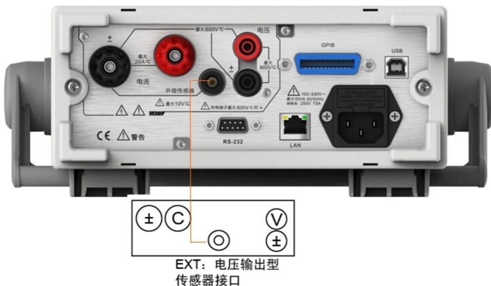
图 4.11 外部电流传感器端子符号
