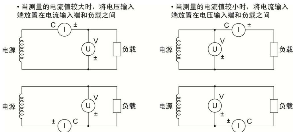
图 4.2 对电压和电流幅值测量的影响
