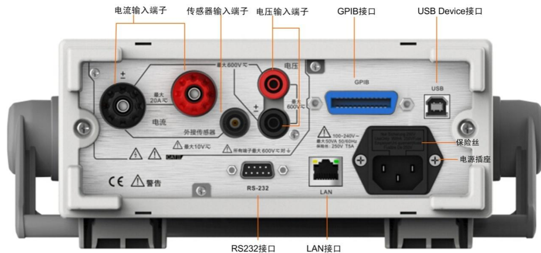
图 3.25 PA310 后面板描述
