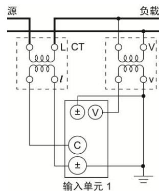
图 4.19 单相两线测量电路
