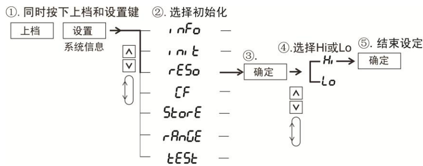
图 6.28 显示位数设置
