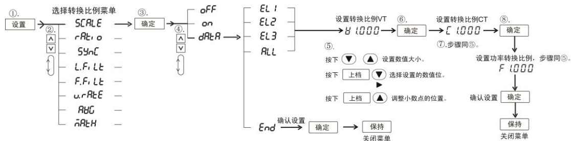
图 6.17 外部 VT/CT 比例常数设置流程
