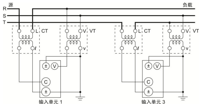
图 4.21 三相三线测量电路接法
