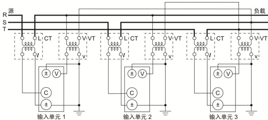
图 4.23 基于 VT 和 CT 的 3V3A 接线方法
