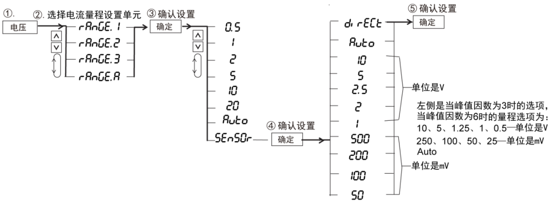
图 6.20 PA323 外部电压输出型传感器选择量程示例
