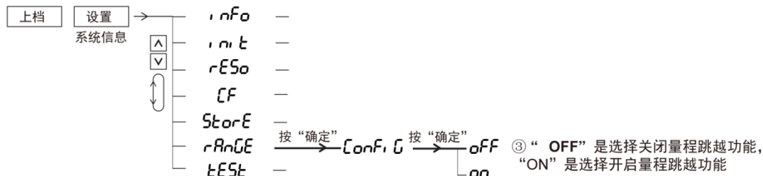
图 6.23 量程跳越功能使用平均功能
