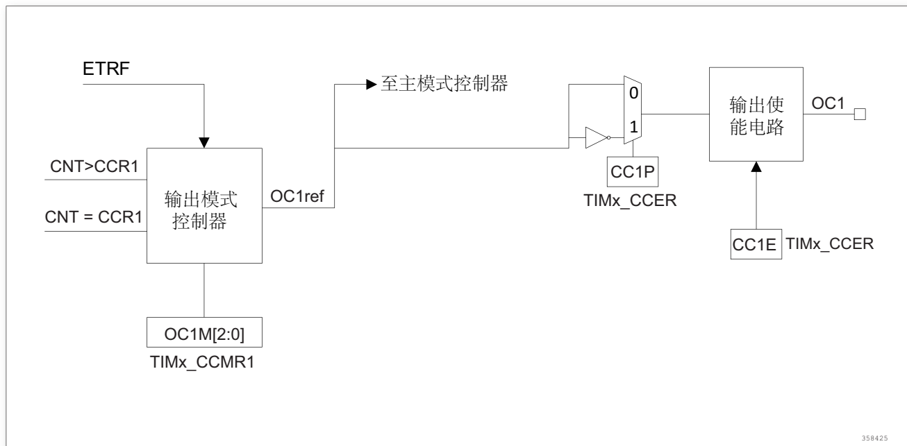
图 182. 捕获/比较通道的输出部分 (通道 1)
