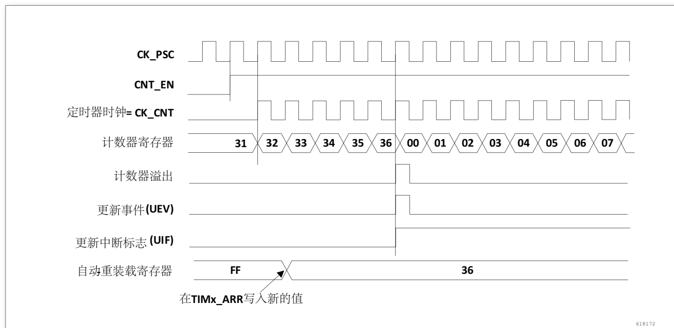
图 192. 计数器时序图，当 ARPE = 0 时的更新事件 (TIMx_ARR 没有预装入)
