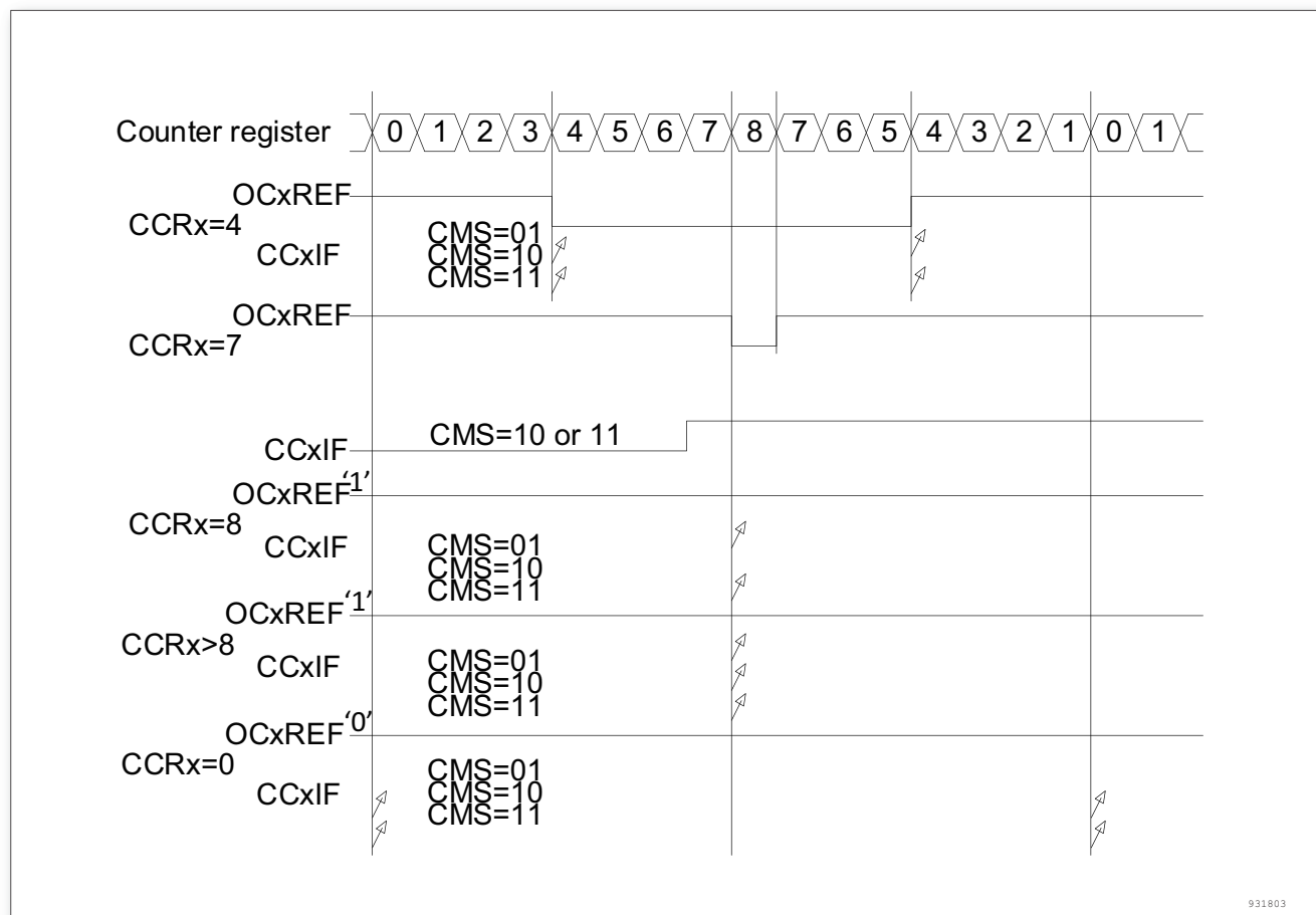
图 63. 中央对齐的 PWM 波形 (ARR = 8)
