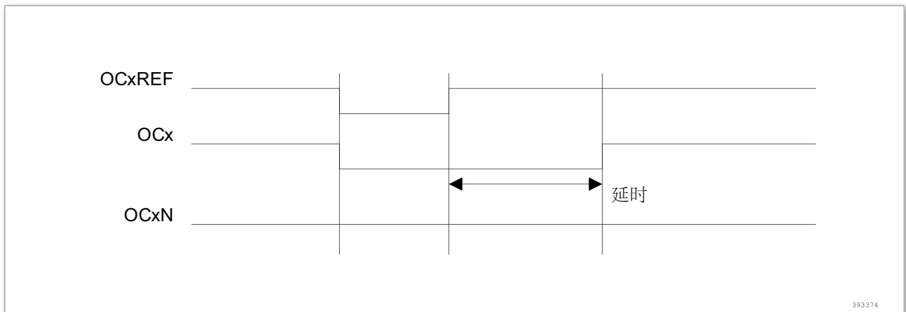
图 65. 死区波形延迟大于负脉冲
