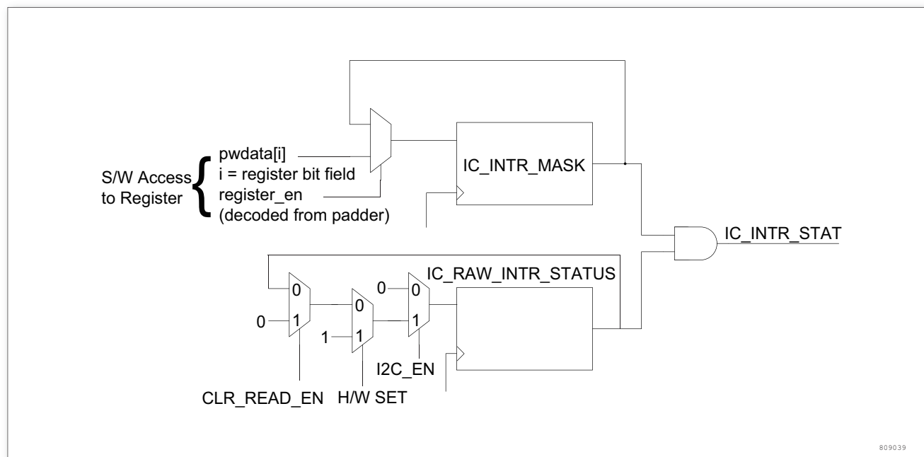
图 225. 中断机制
