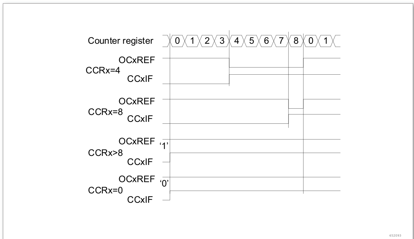
图 62. 边沿对齐的 PWM 波形 (ARR = 8)
