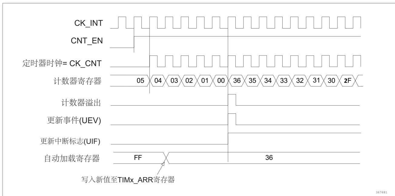
图 137. 计数器时序图，当没有使用重复计数器时的更新事件
