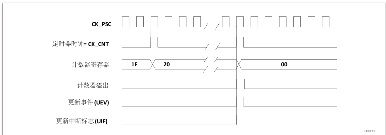
图 191. 计数器时序图，内部时钟分频因子为 N
