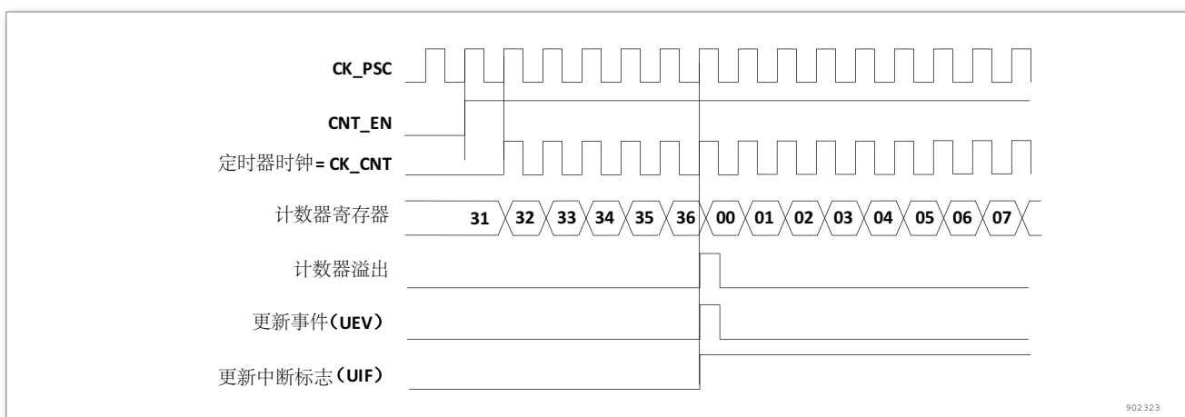
图 188. 计数器时序图，内部时钟分频因子为 1
