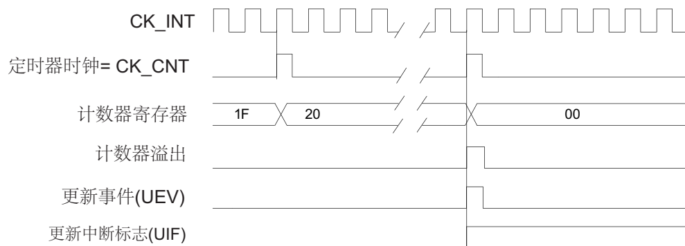
图 130. 计数器时序图，内部时钟分频因子为 N
