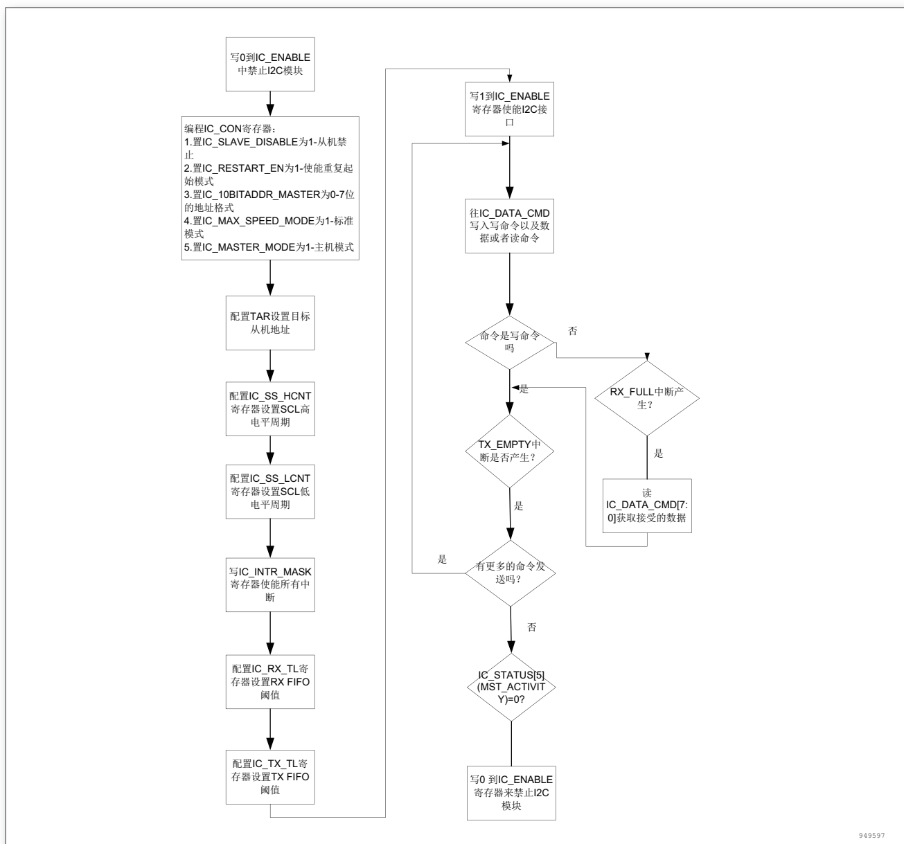
图 224. I 2 C 接口主机流程图
