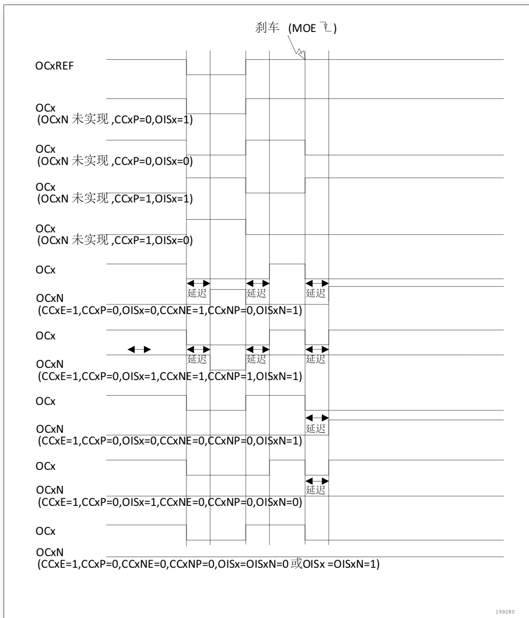
图 204. 响应刹车的输出
