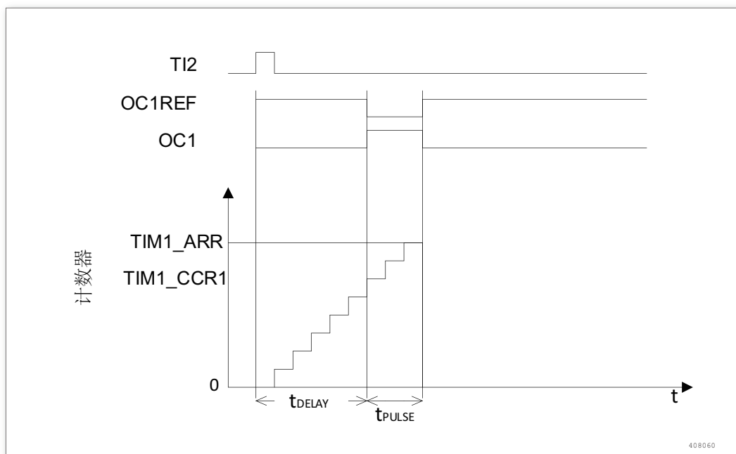
图 205. 单脉冲模式的例子
