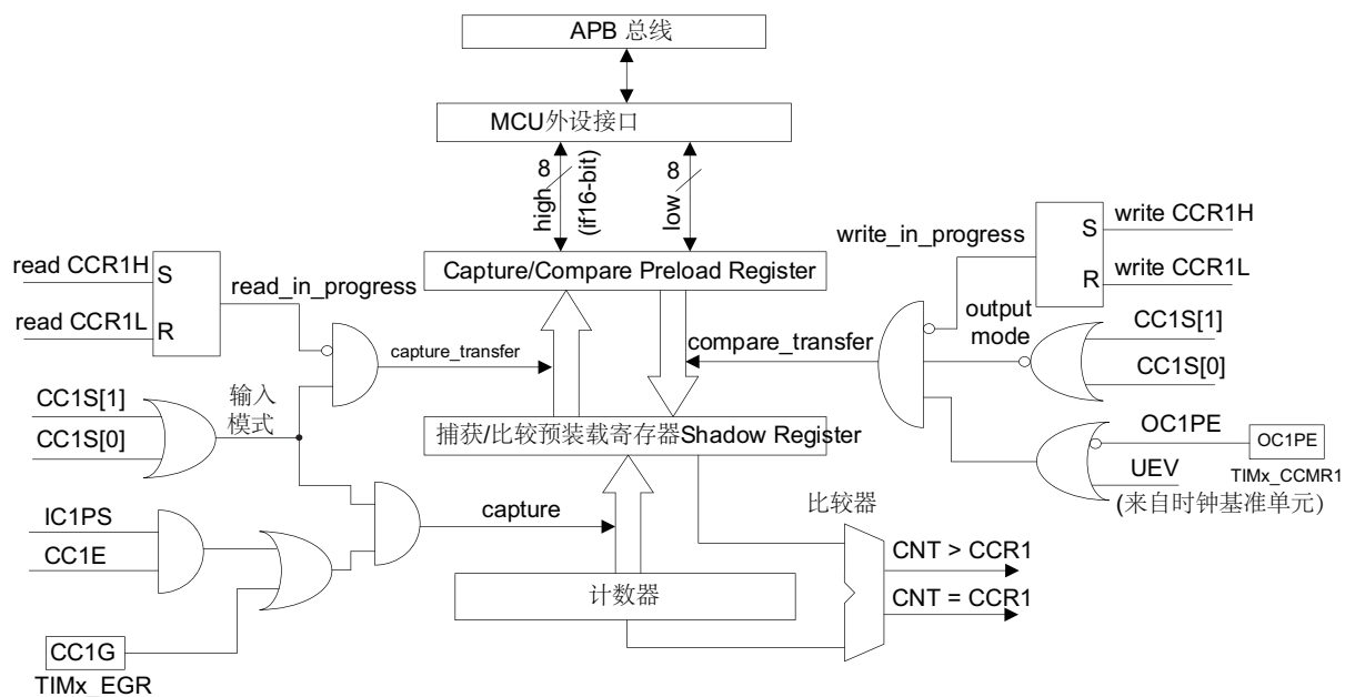
图 57. 捕获/比较通道 1 的主电路
