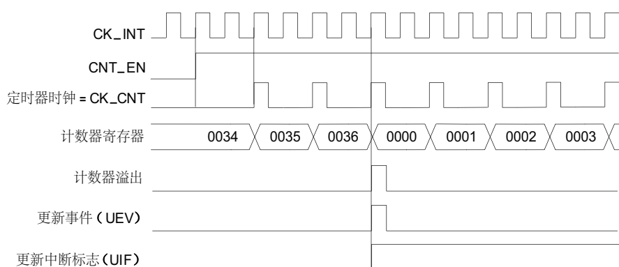
图 128. 计数器时序图，内部时钟分频因子为 2
