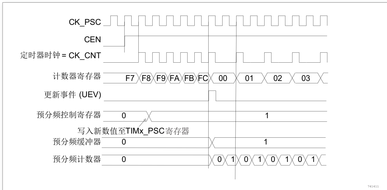
图 186. 当预分频器的参数从 1 变到 2 时, 计数器的时序图
