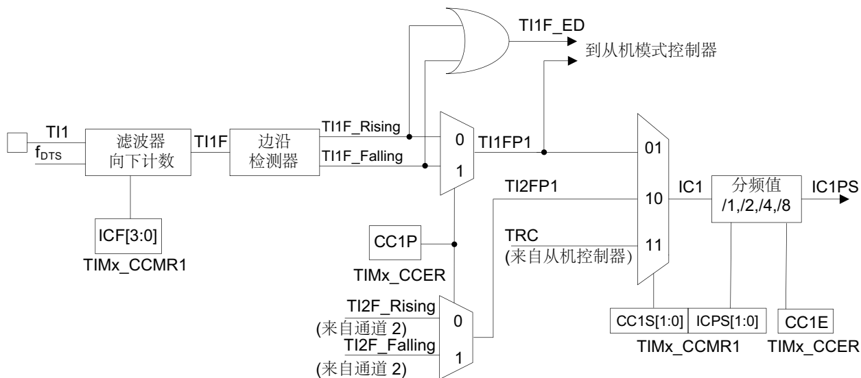
图 56. 捕获/比较通道 (如：通道 1 输入部分)
