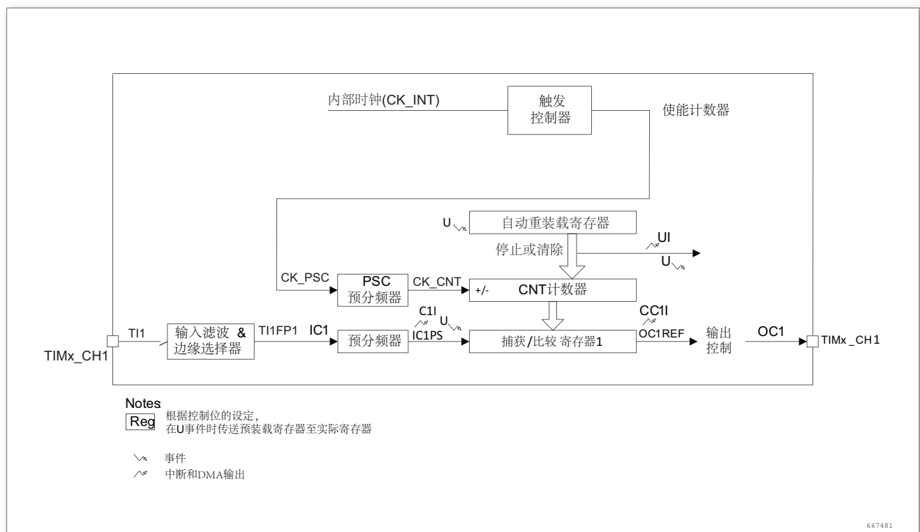
图 170. 基础定时器框图
