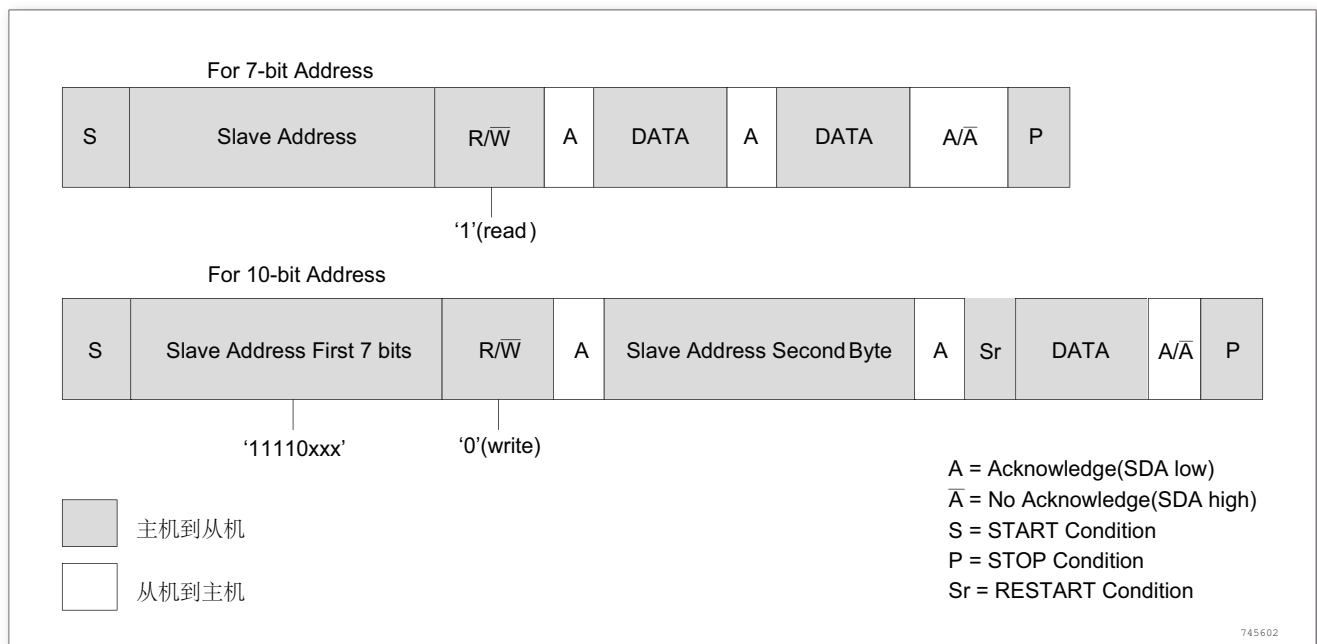
图 216. 主接收协议
