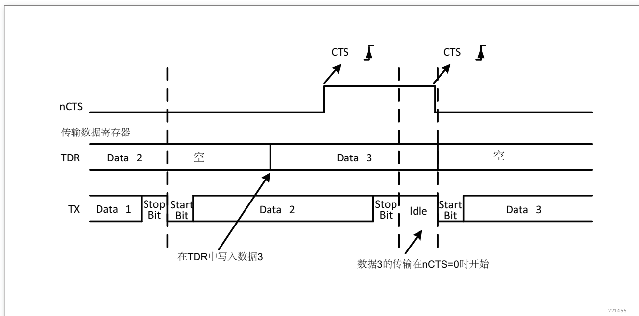
图 232. CTS 流控制
