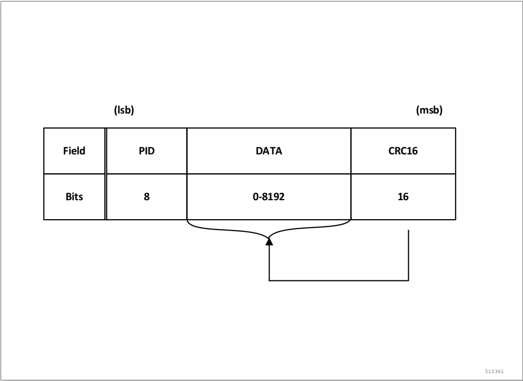
图 234. 包的基本格式
