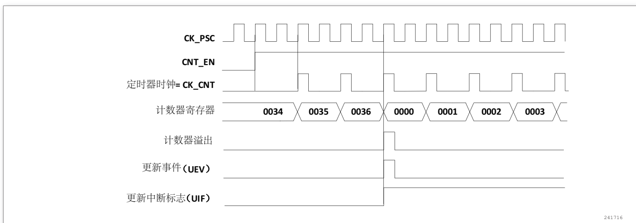
图 189. 计数器时序图，内部时钟分频因子为 2
