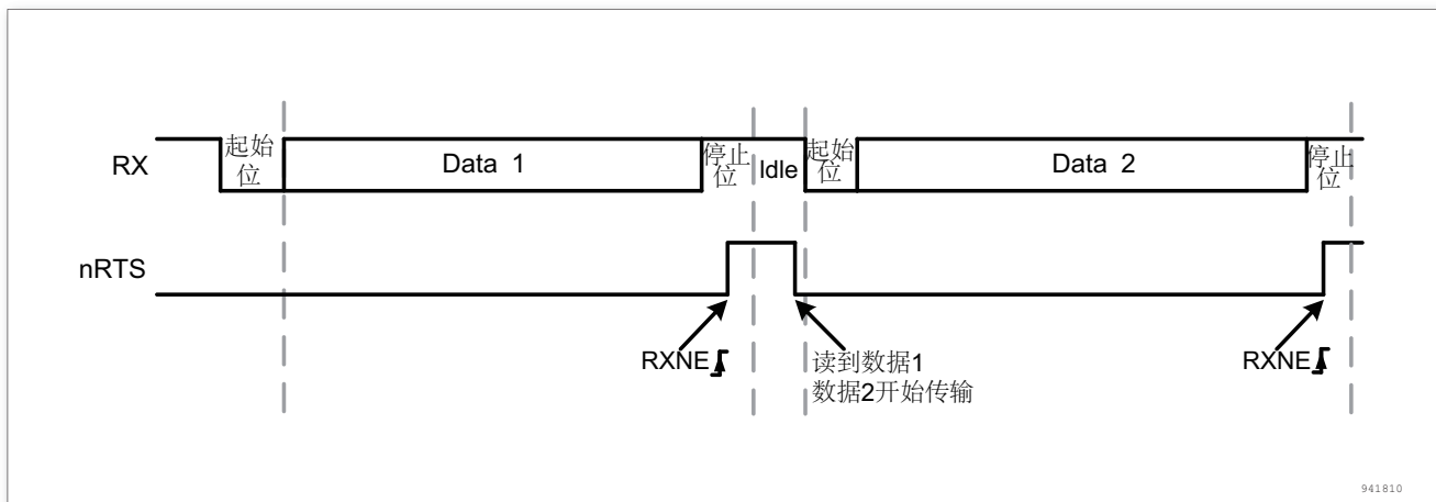
图 231. RTS 流控制
