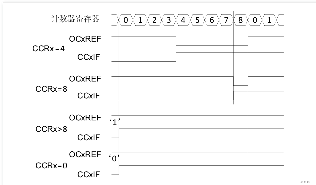
图 184. 边沿对齐的 PWM 波形 (ARR = 8)
