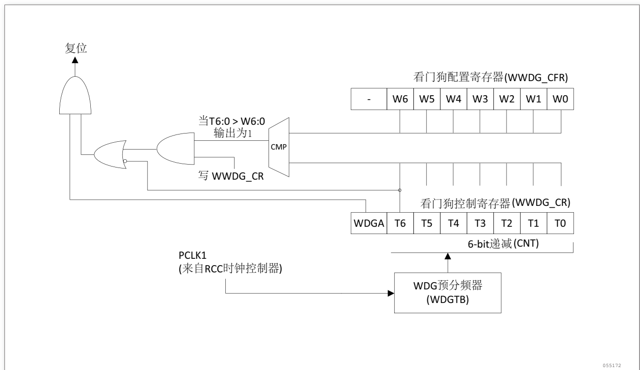
图 207. 看门狗框图
