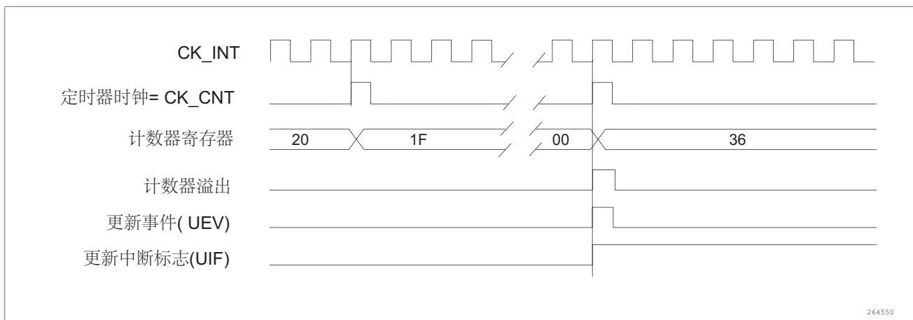
图 136. 计数器时序图，内部时钟分频因子为 N
