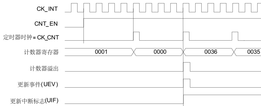
图 135. 计数器时序图，内部时钟分频因子为 4
