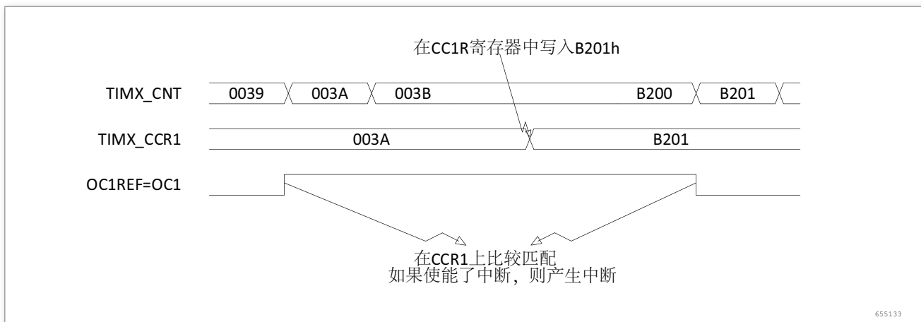
图 199. 输出比较模式，翻转 OC1
