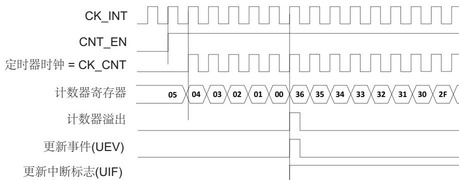
图 133. 计数器时序图，内部时钟分频因子为 1
