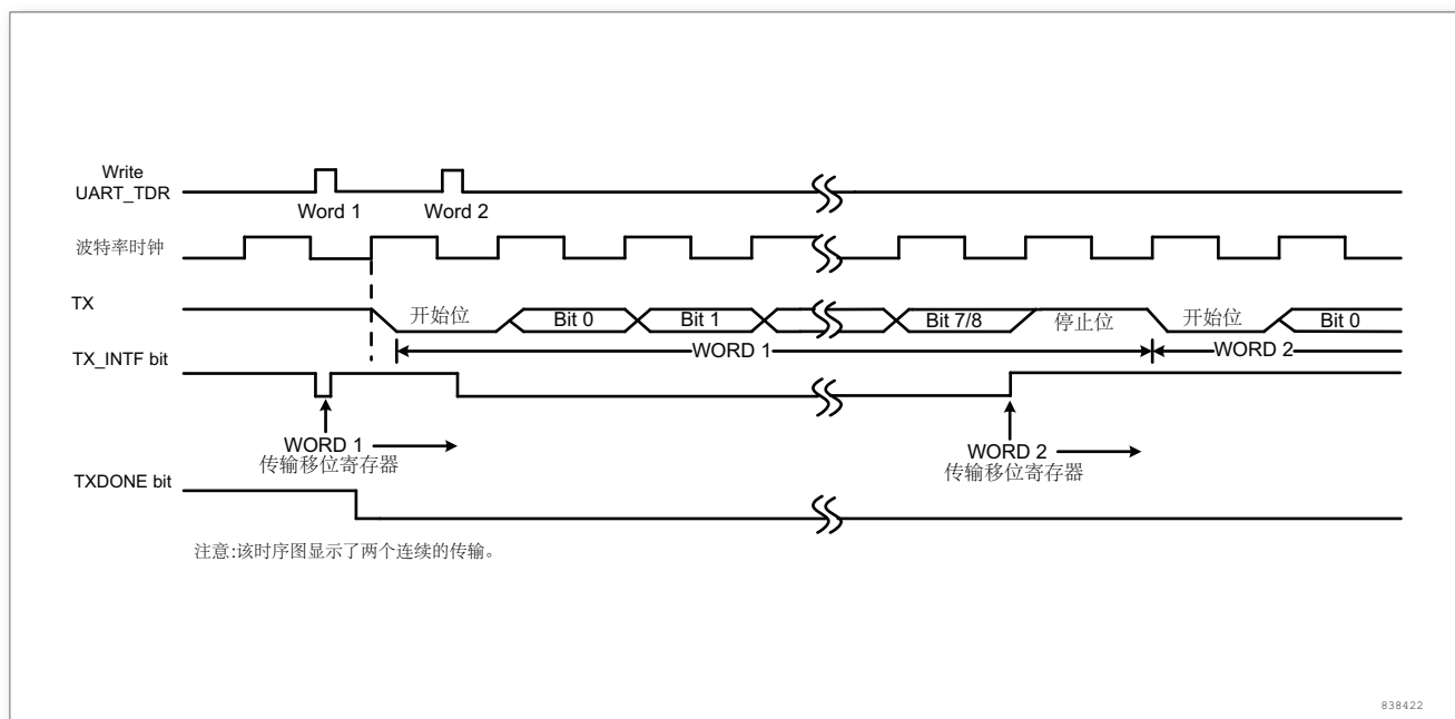
图 228. 发送时状态位变化
