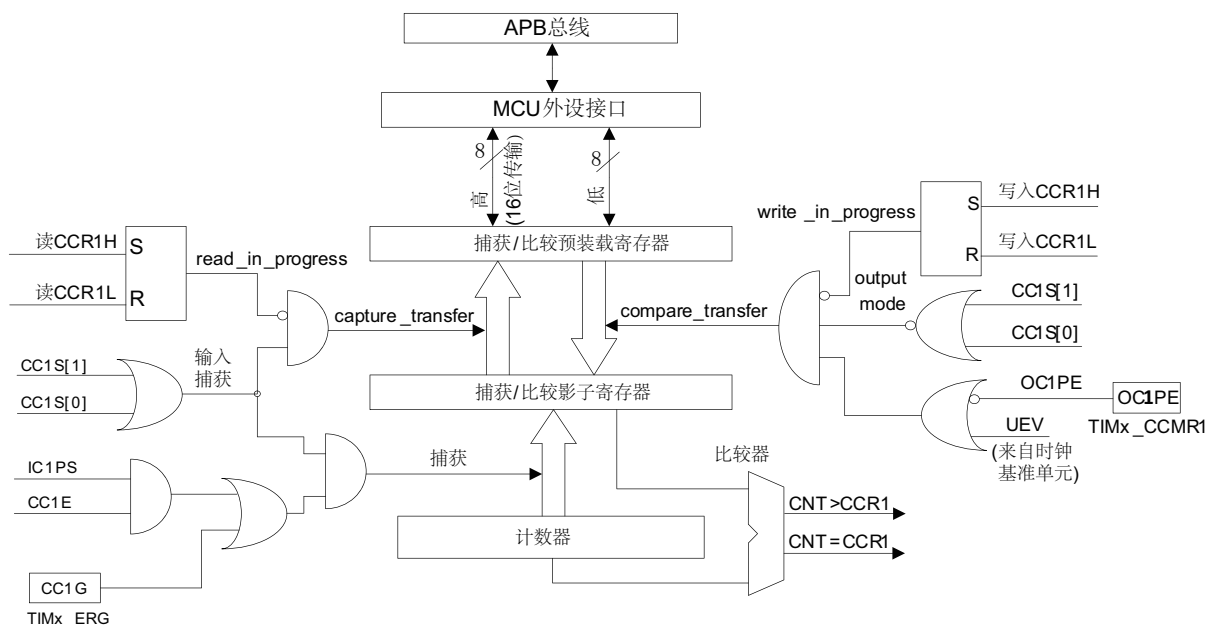
图 181. 捕获/比较通道 1 的主电路
