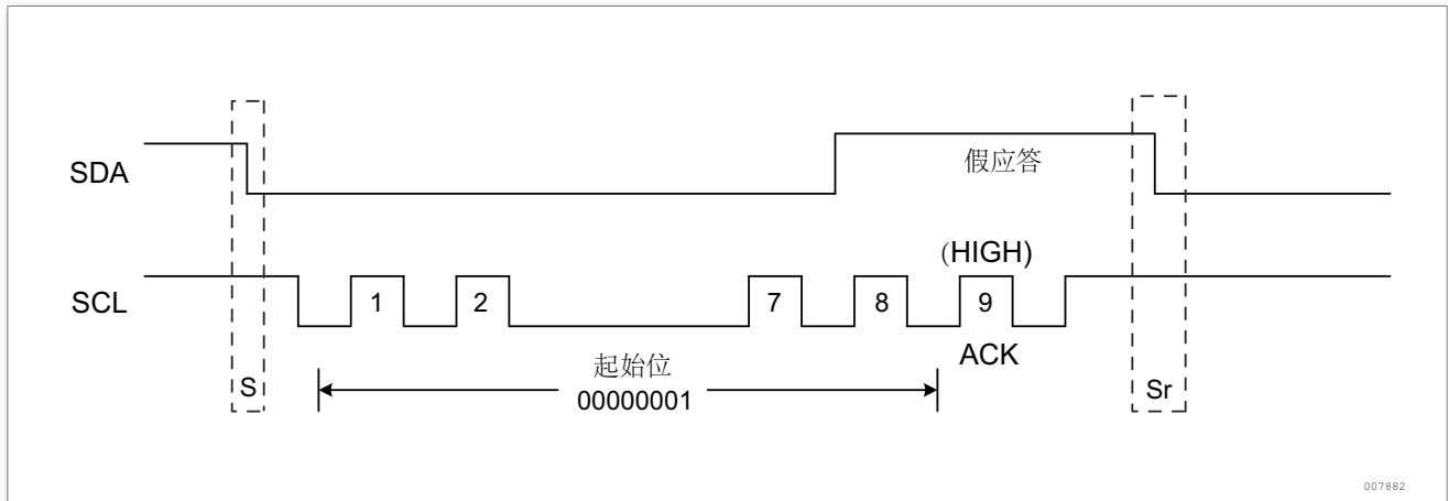
图 217. 起始字节传输
