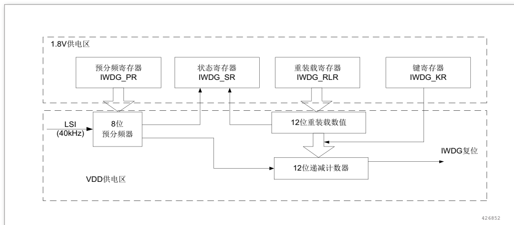
图 206. 独立看门狗框图
