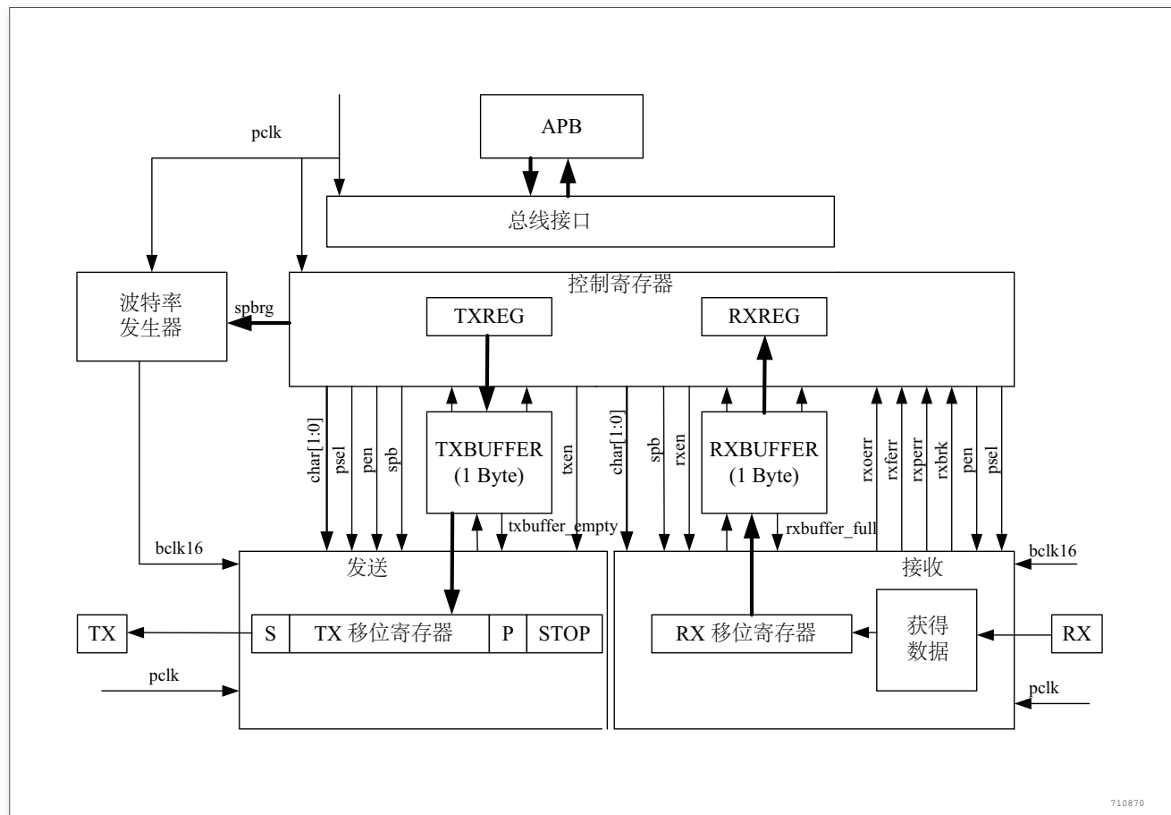
图 226. UART 方框图
