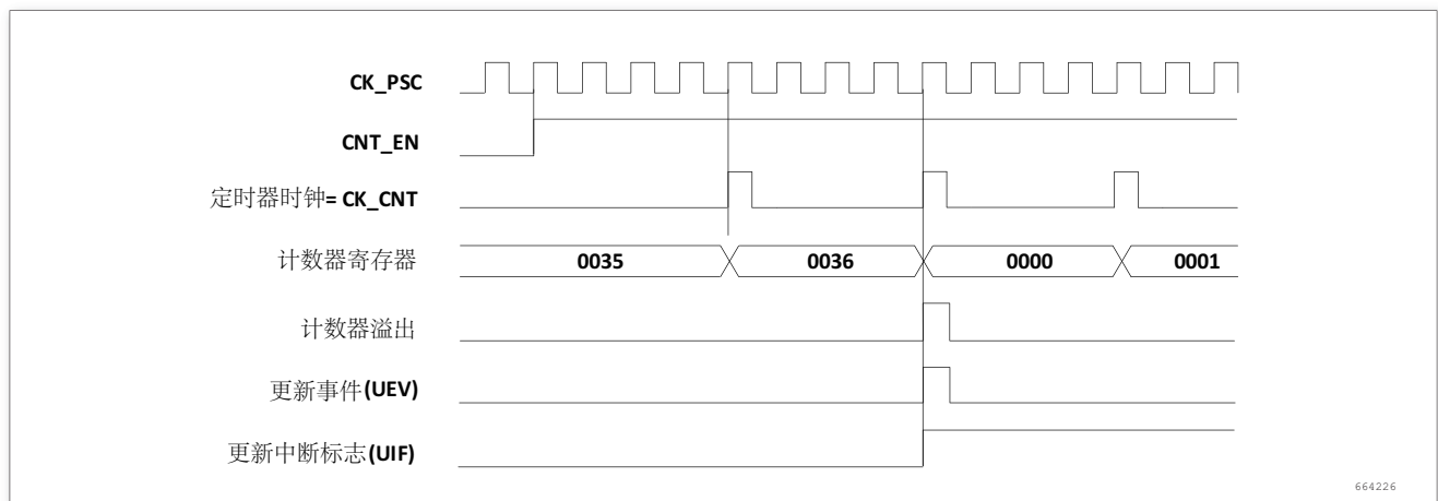
图 190. 计数器时序图，内部时钟分频因子为 4
