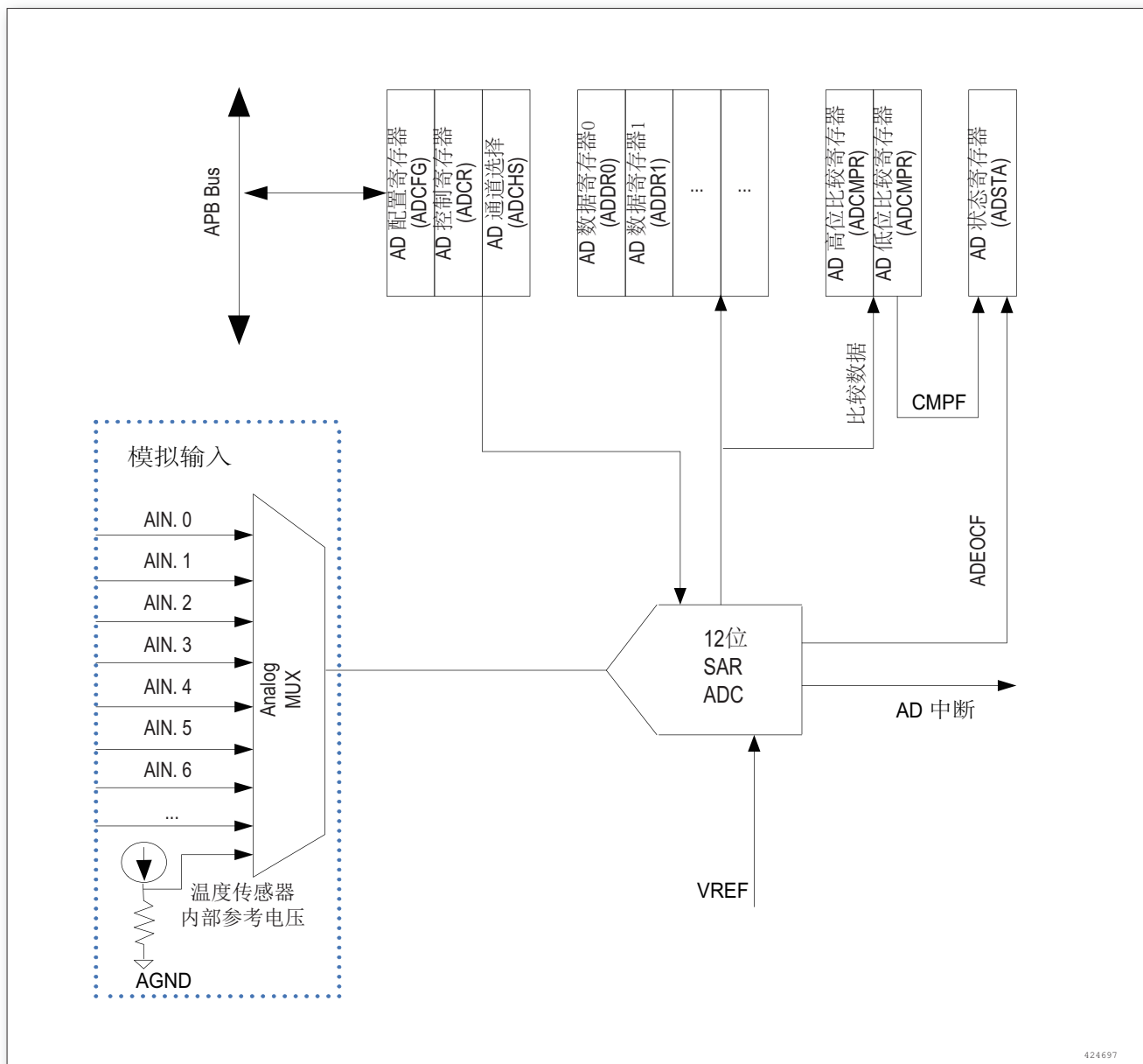
图 23. ADC 框图
