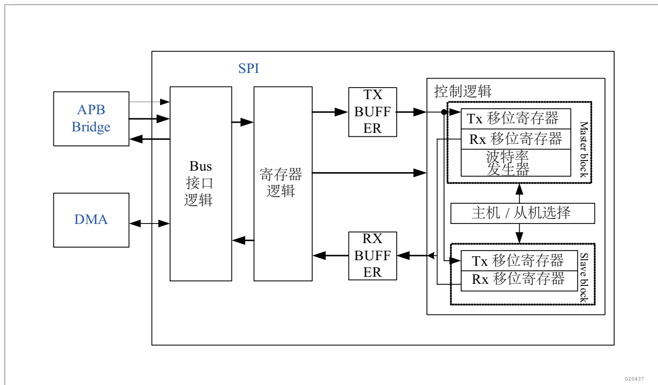
图 209. SPI 框图
