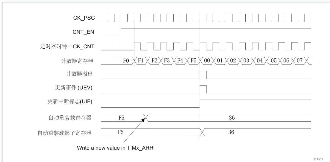
图 178. 计数器时序图，当 ARPE = 1 时的更新事件 (预装入了 TIM14_ARR)
