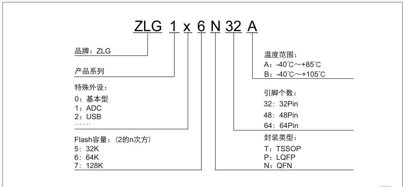
图 239. ZLG1x6 型号命名
