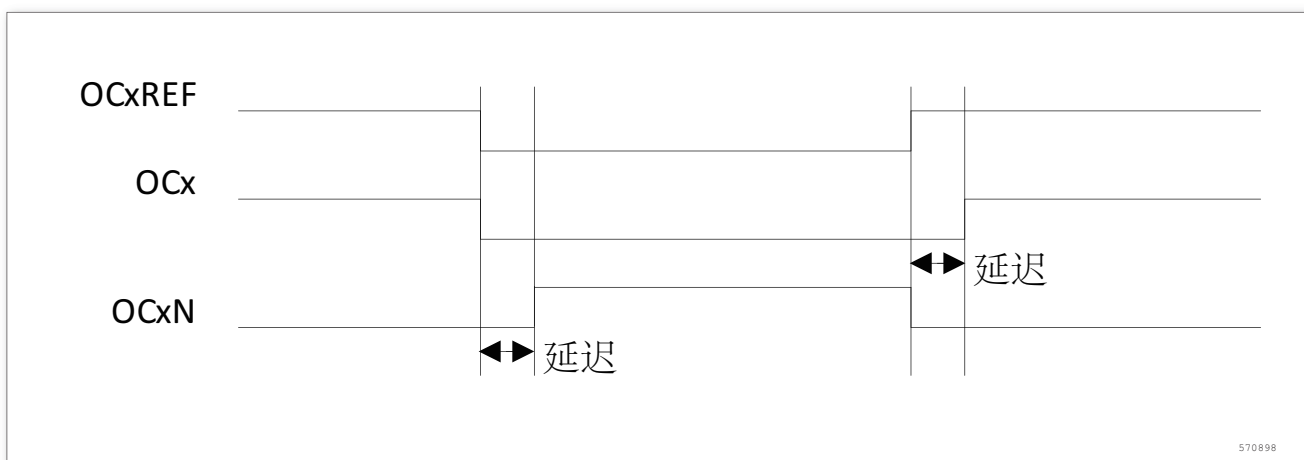
图 201. 带死区插入的互补输出
