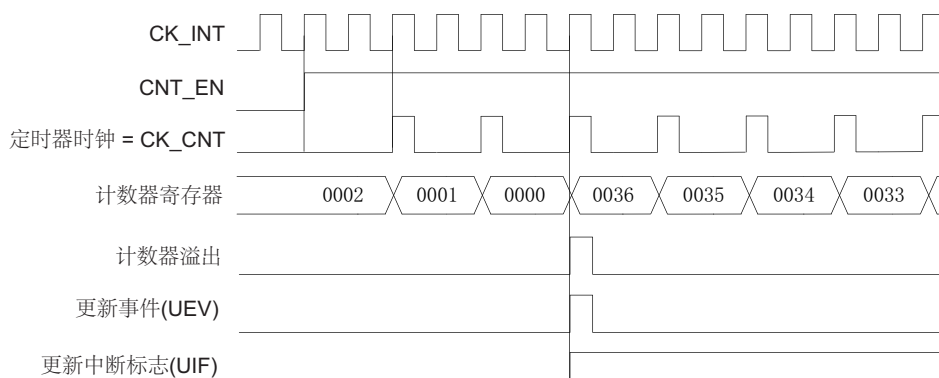
图 134. 计数器时序图，内部时钟分频因子为 2
