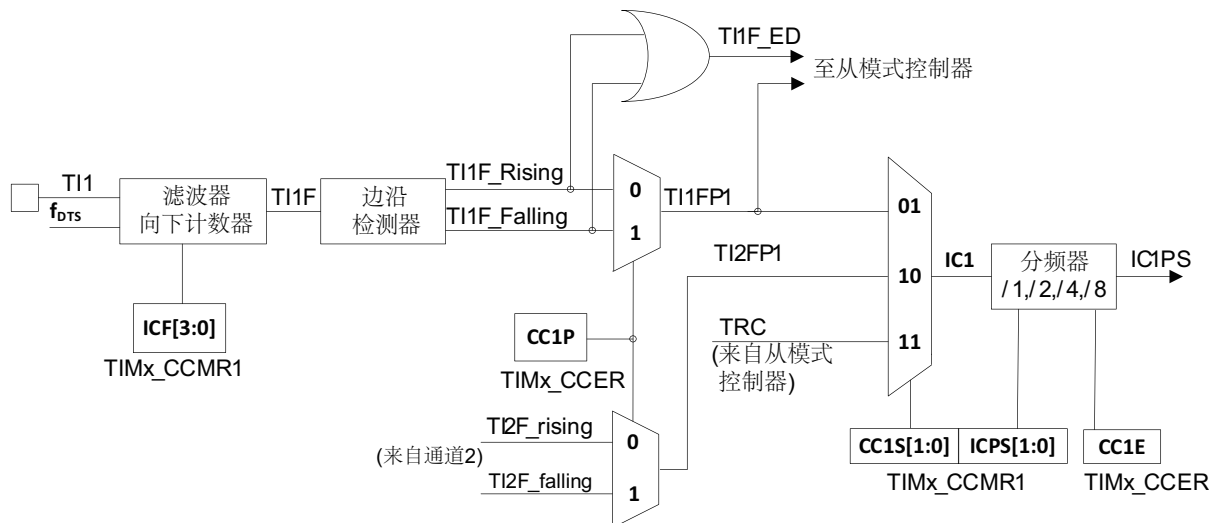
图 180. 捕获/比较通道 (如: 通道 1 输入部分)
