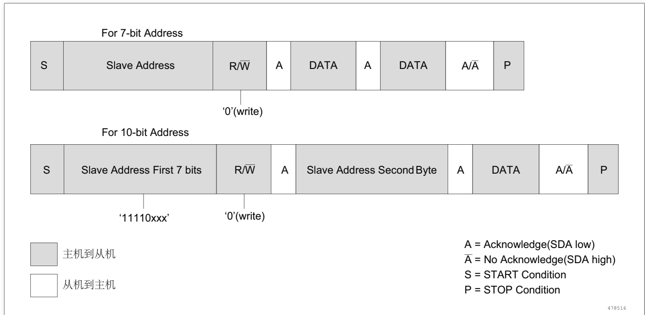
图 215. 主发送协议
