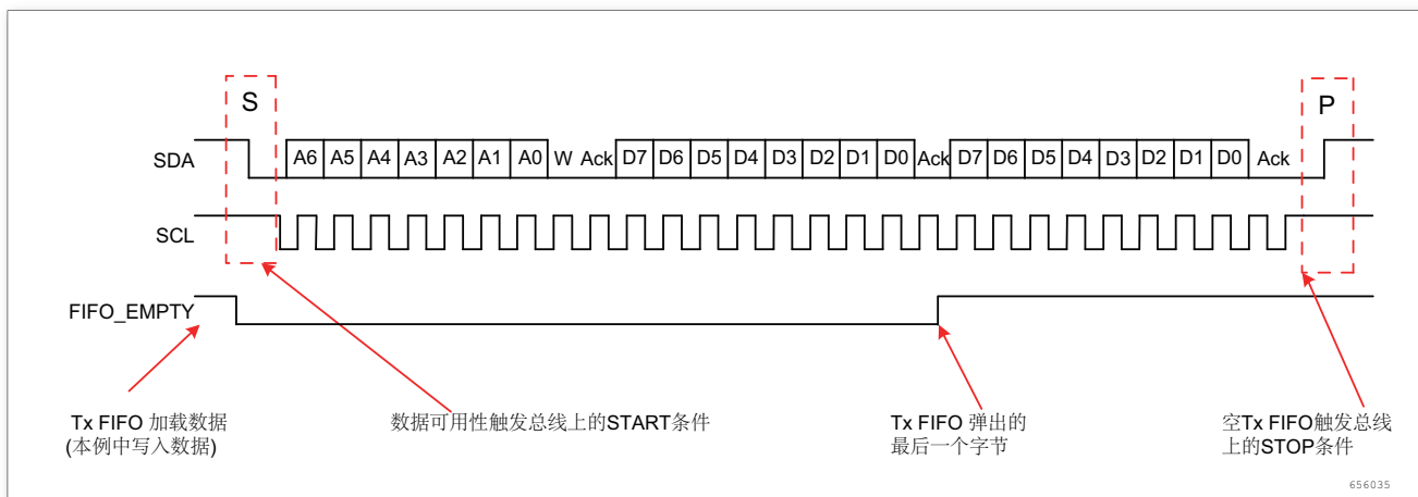
图 219. 主发送 - Tx FIFO 为空
