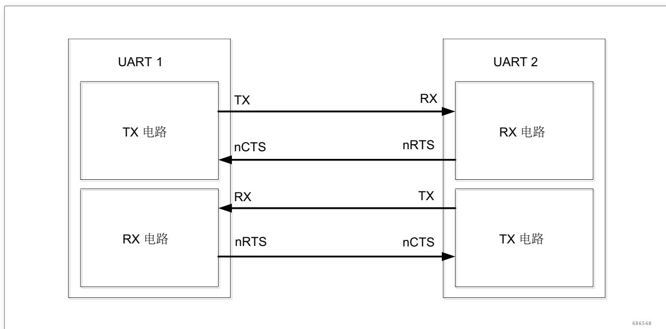
图 230. 两个 UART 间的硬件流控制
