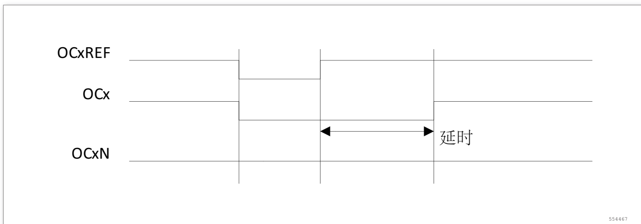
图 202. 死区波形延迟大于负脉冲
