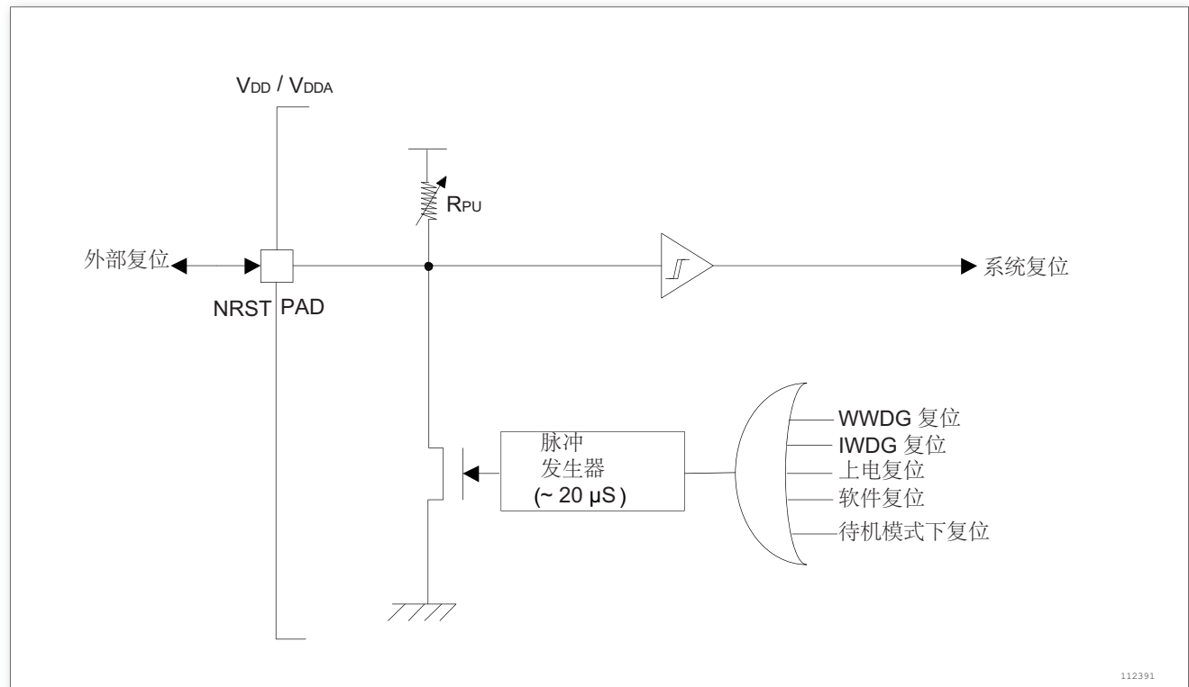
图 10. 复位电路
