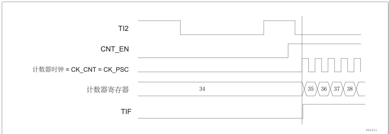
图 162. 触发器模式下的控制电路
