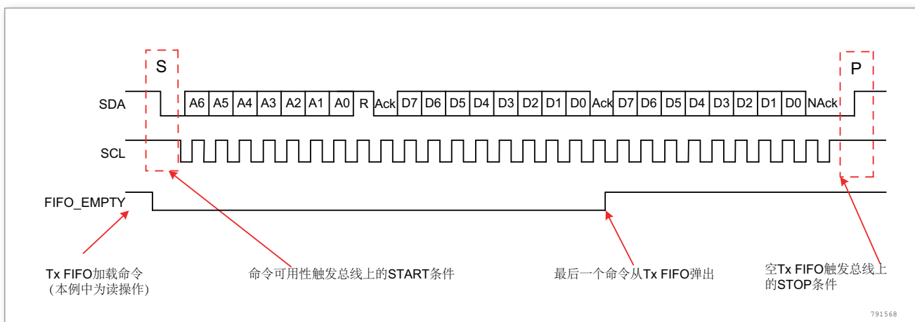
图 220. 主接收 - Tx FIFO 为空
