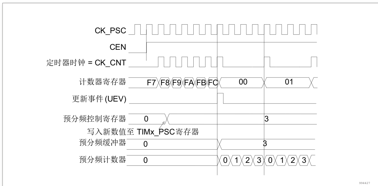
图 187. 当预分频器的参数从 1 变到 4 时, 计数器的时序图
