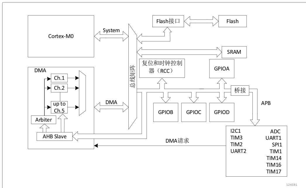
图 21. DMA 框图
