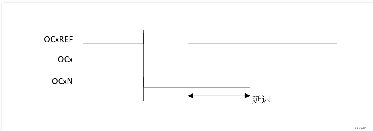
图 203. 死区波形延迟大于正脉冲
