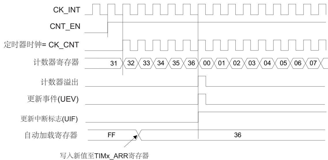
图 177. 计数器时序图，当 ARPE = 0 时的更新事件 (TIM14_ARR 没有预装入)
