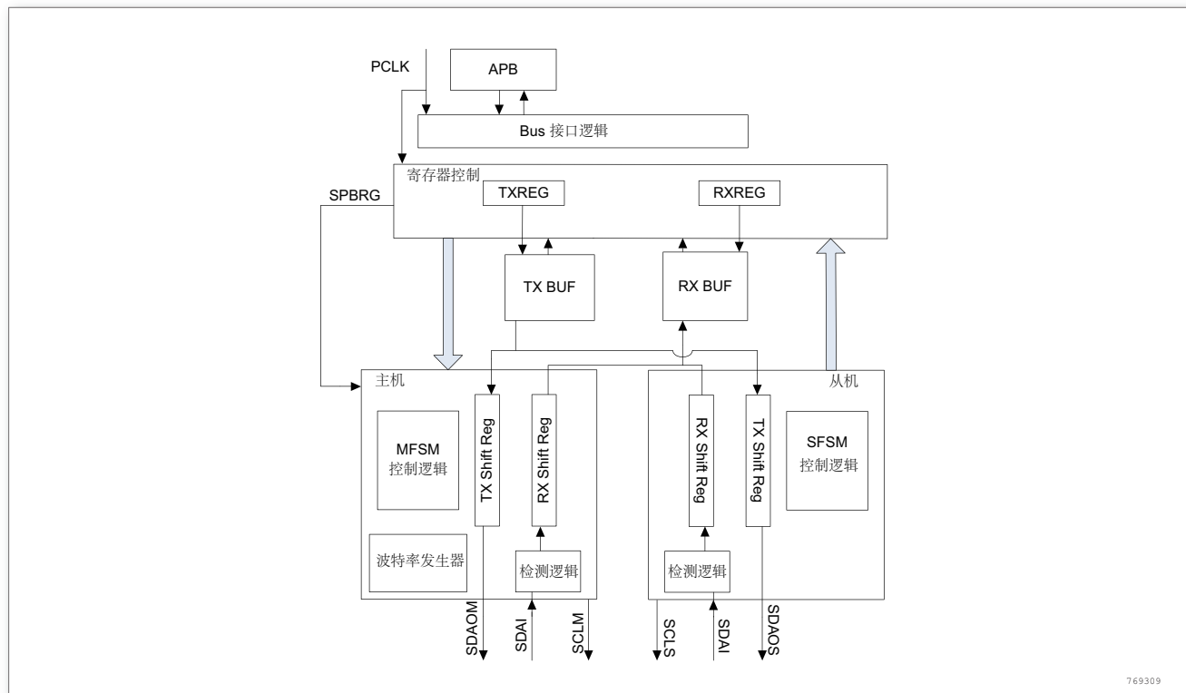
图 223. I 2 C 功能框图
