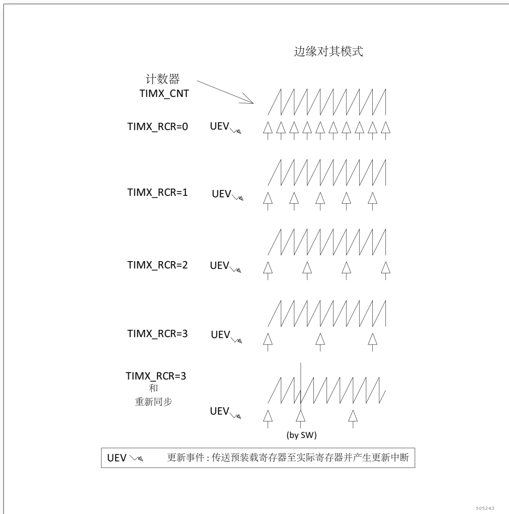
图 194. 不同模式及不同 TIMx_RCR 寄存器设置下更新速率的例子
