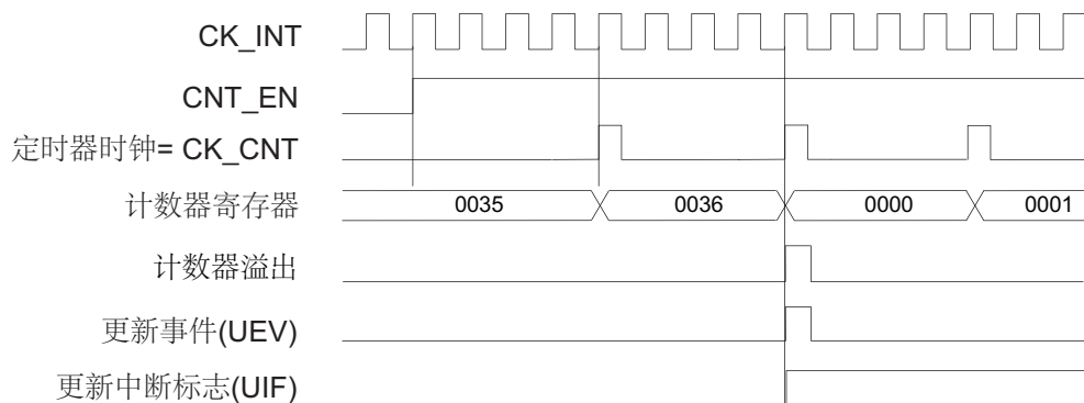
图 129. 计数器时序图，内部时钟分频因子为 4
