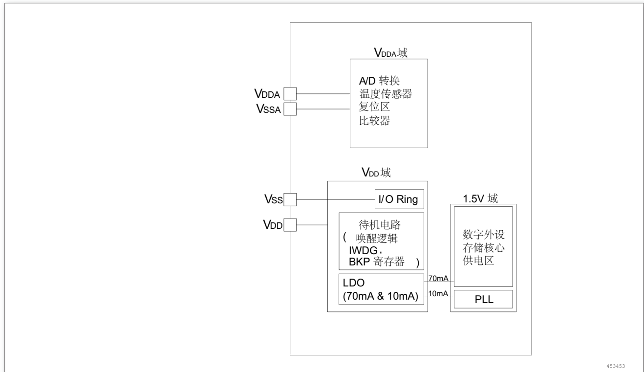
图 7. 电源框图
