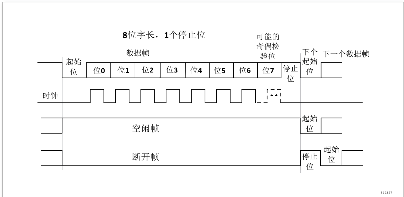
图 227. UART 时序
