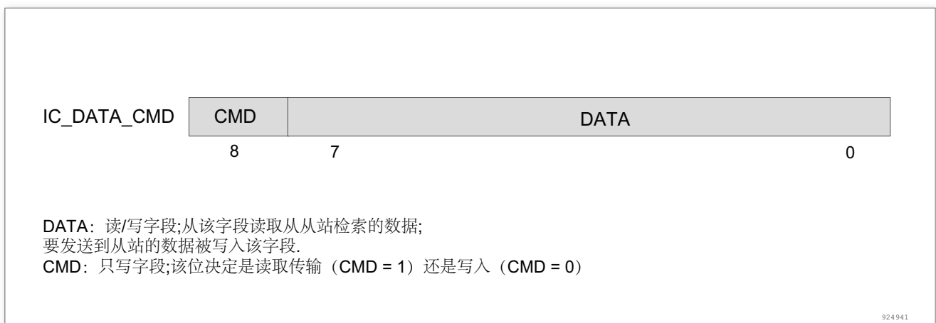
图 218. IC_DATA_CMD 寄存器
