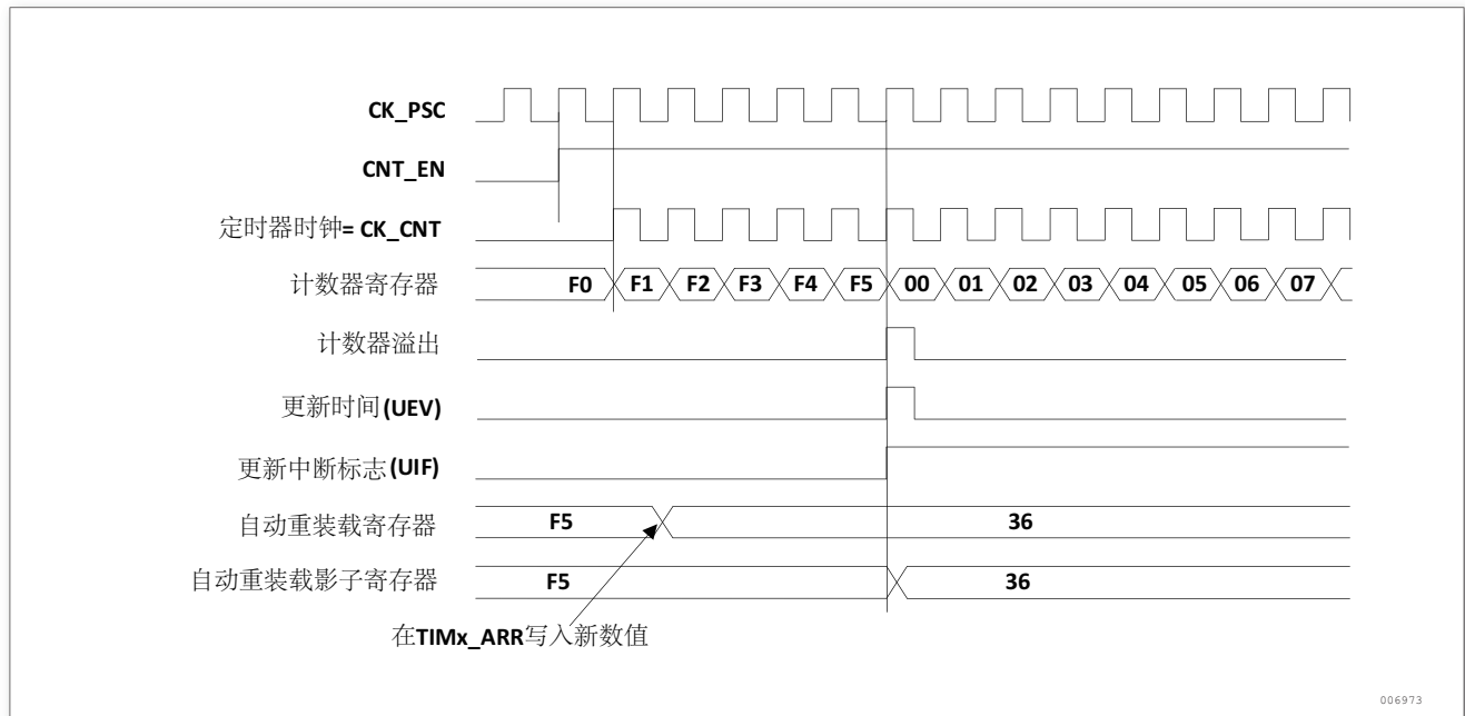
图 193. 计数器时序图，当 ARPE = 1 时的更新事件 (TIMx_ARR 预装载)
