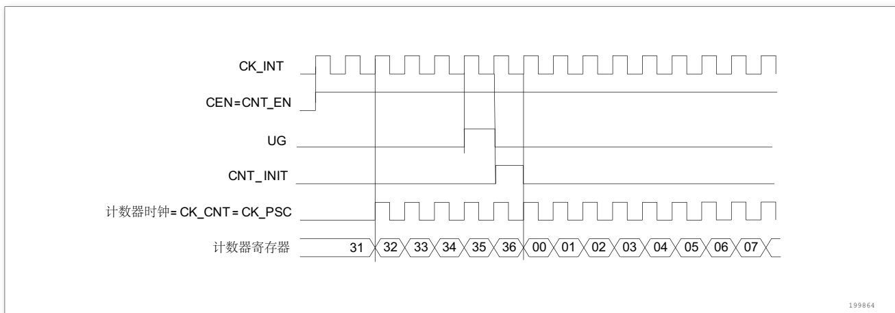
图 179. 一般模式下的控制电路，内部时钟分频因子为 1
