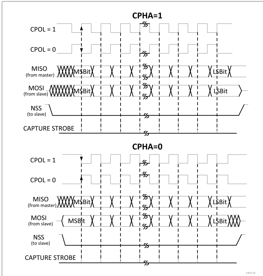
图 211. 数据时钟时序图
