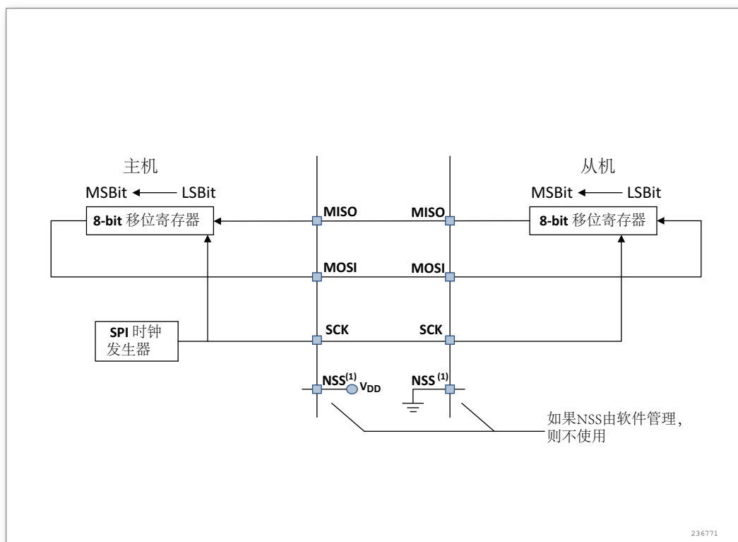
图 210. 单主和单从应用
