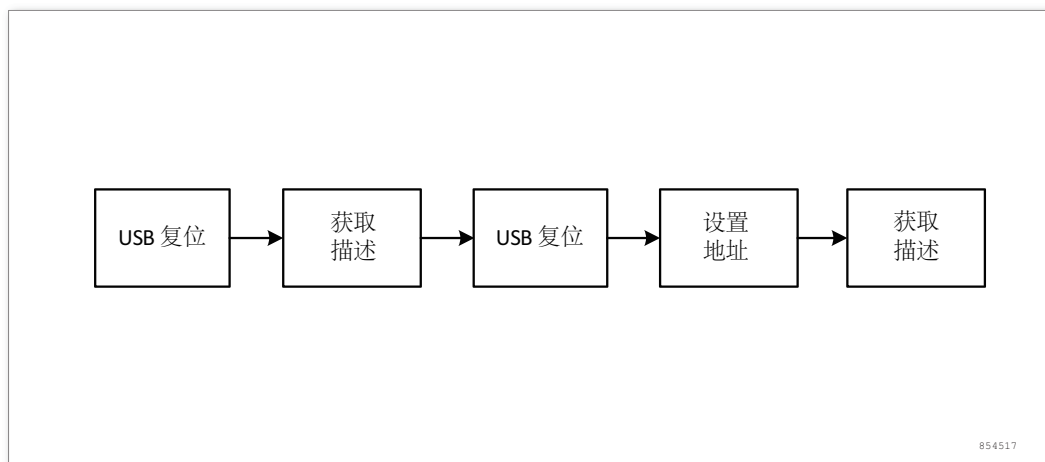
图 237. 枚举过程
