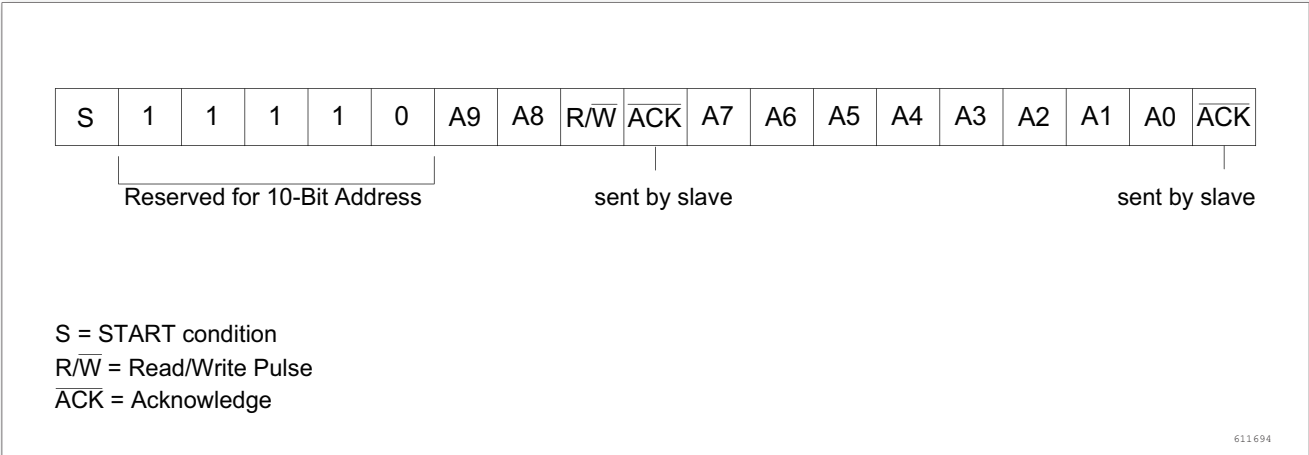
图 214. 10 位的地址格式
