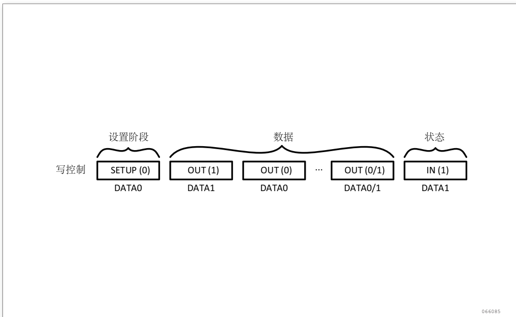
图 236. USB 传输
