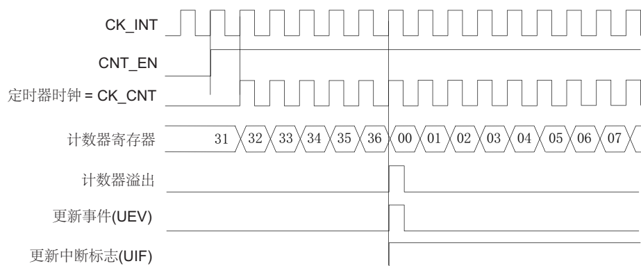
图 173. 计数器时序图，内部时钟分频因子为 1
