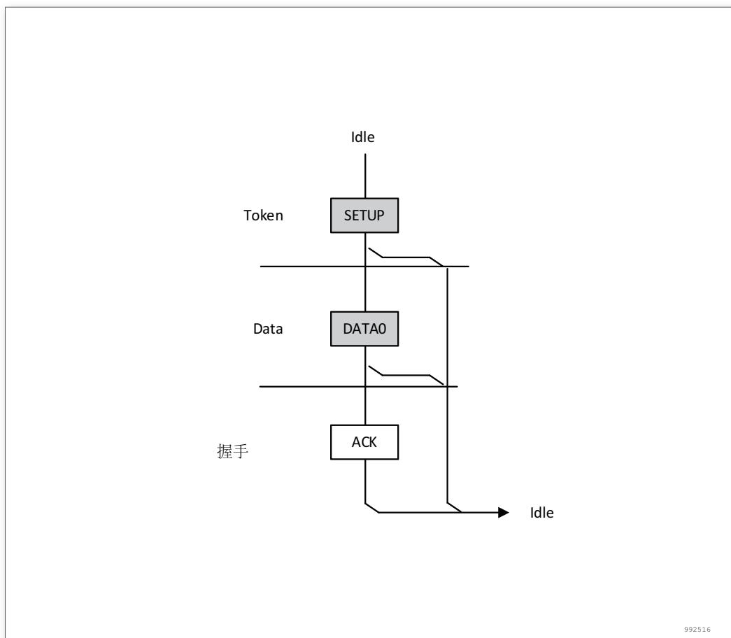
图 235. USB 事务
