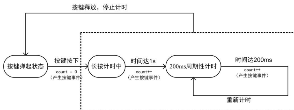
图 2.1 长按普通按键时的事件产生过程
