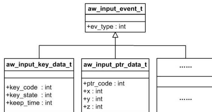
图 5.1 各种类型的输入事件对应的实际数据类图
