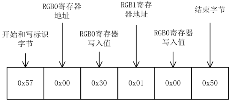
图 7.7 修改波特率为 115200bps 命令字节
