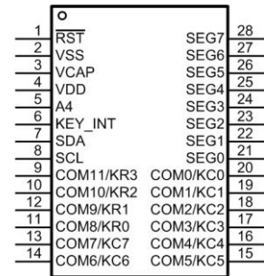
图 1.1 ZLG72128 管脚排列图
