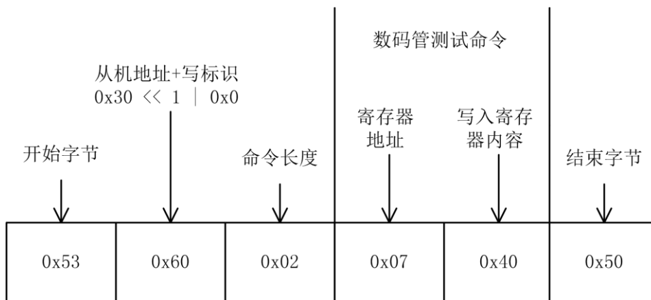
图 7.2 数码管测试命令字节
