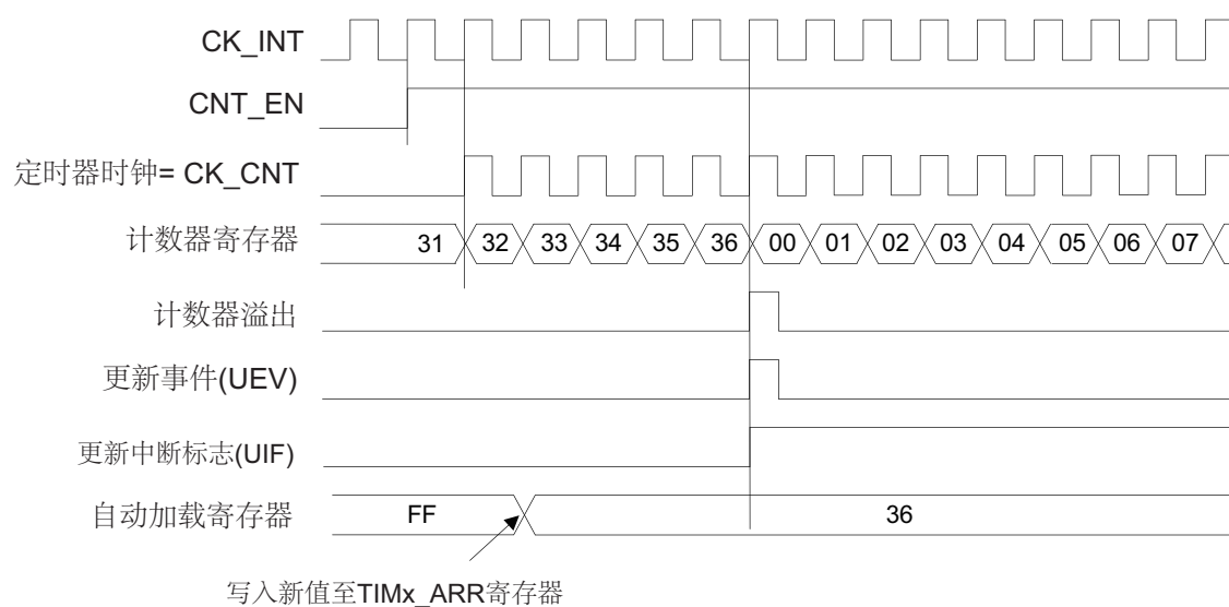
图 178. 计数器时序图，当 ARPE = 0 时的更新事件 (TIM14_ARR 没有预装入)
