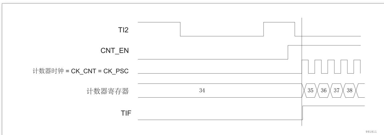
图 117. 触发器模式下的控制电路
