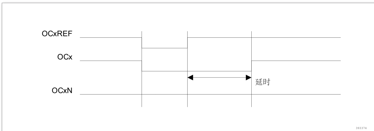
图 66. 死区波形延迟大于负脉冲
