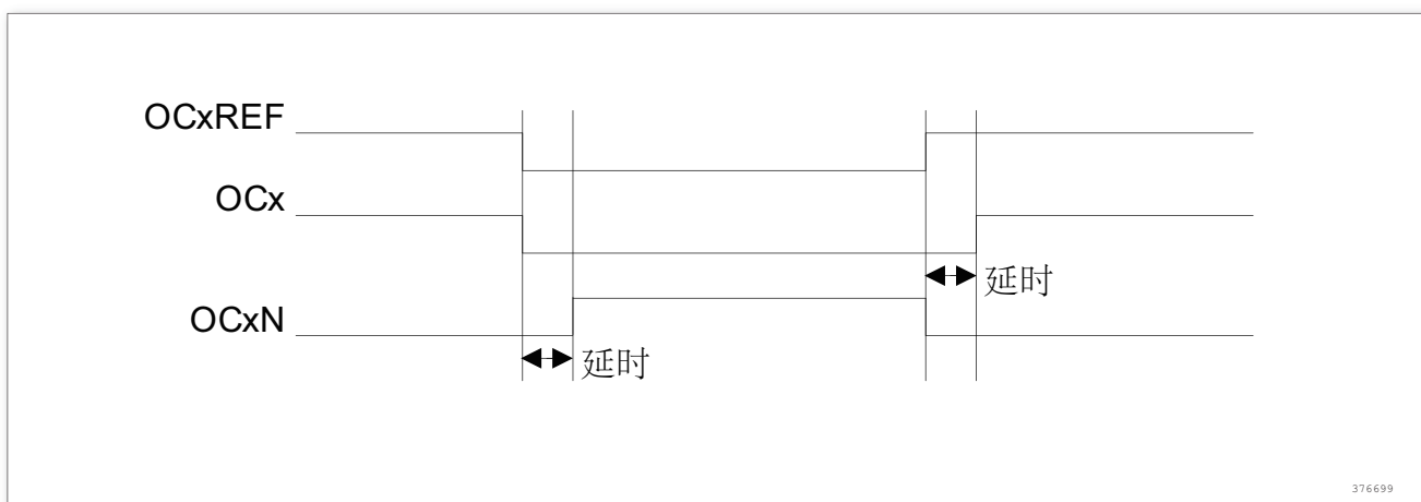
图 65. 带死区插入的互补输出
