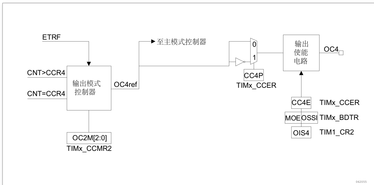
图 60. 捕获/比较通道的输出部分 (通道 4)
