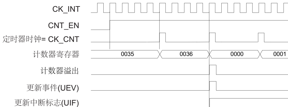
图 84. 计数器时序图，内部时钟分频因子为 4
