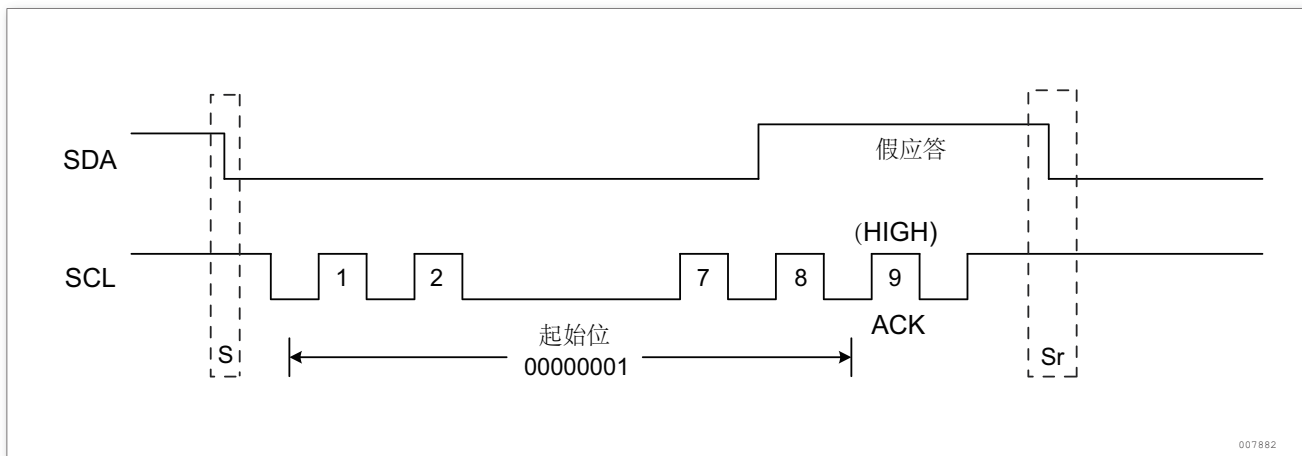
图 218. 起始字节传输
