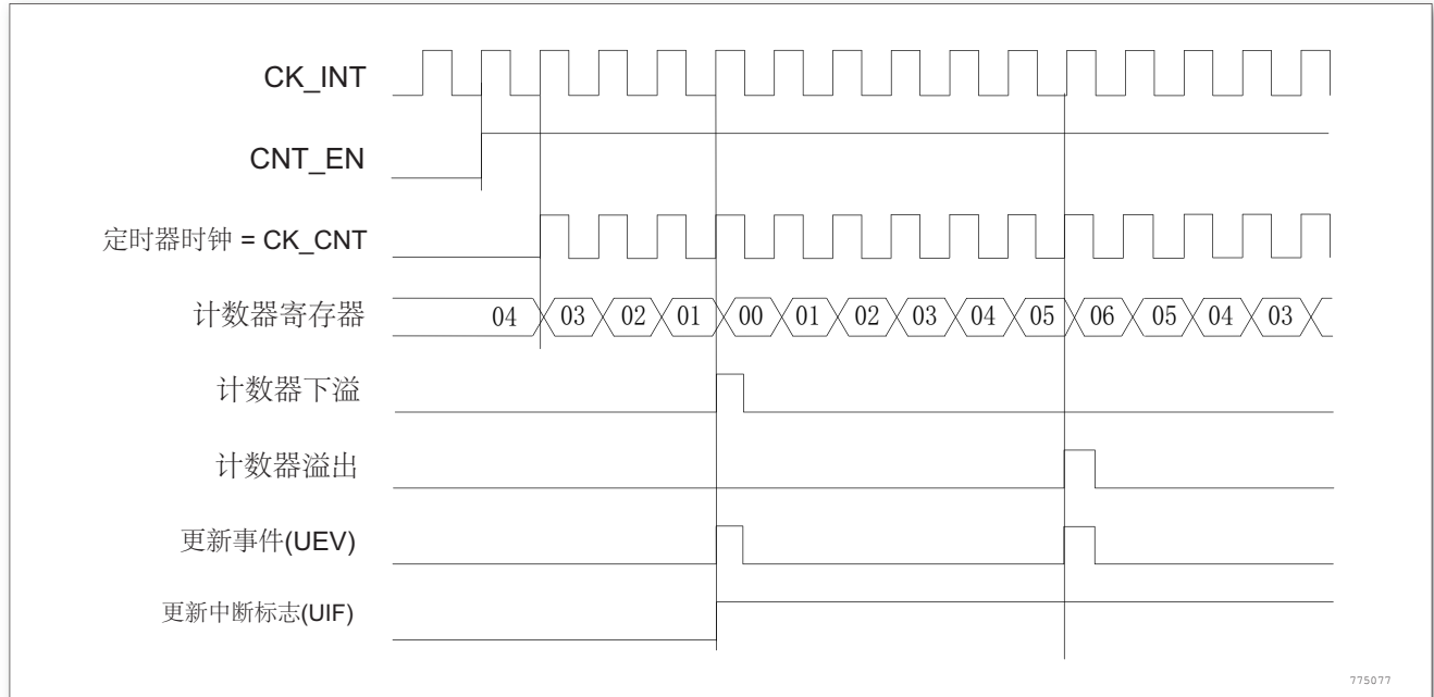
图 93. 计数器时序图，内部时钟分频因子为 1，TIMx_ARR = 0x6
