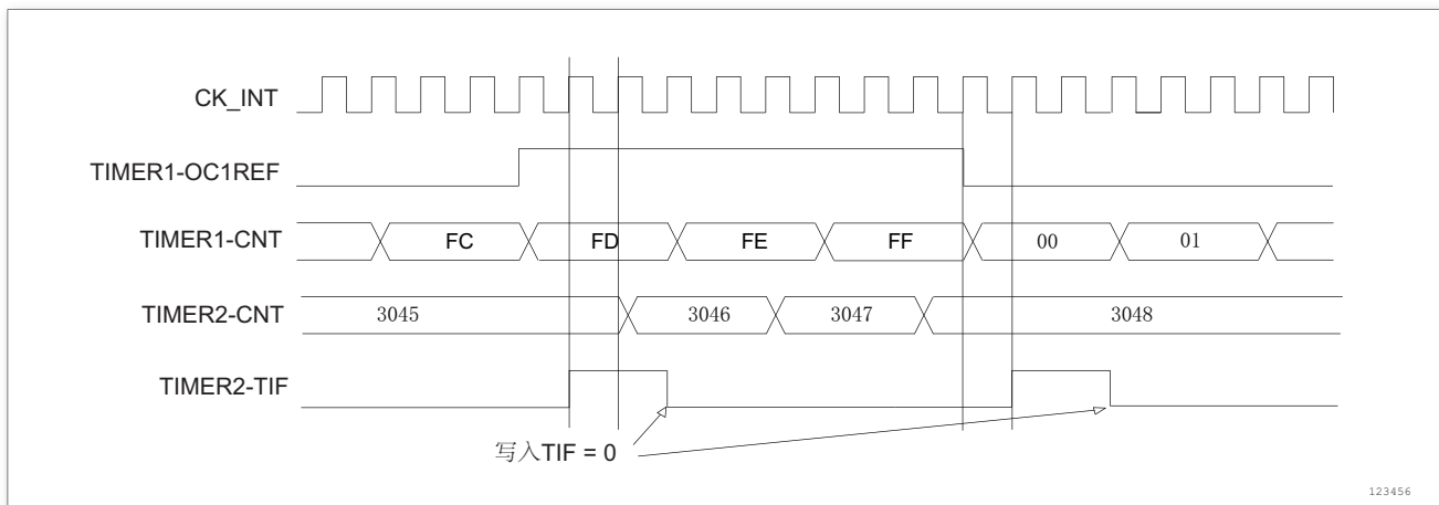
图 166. 定时器 1 的 OC1REF 控制定时器 2
