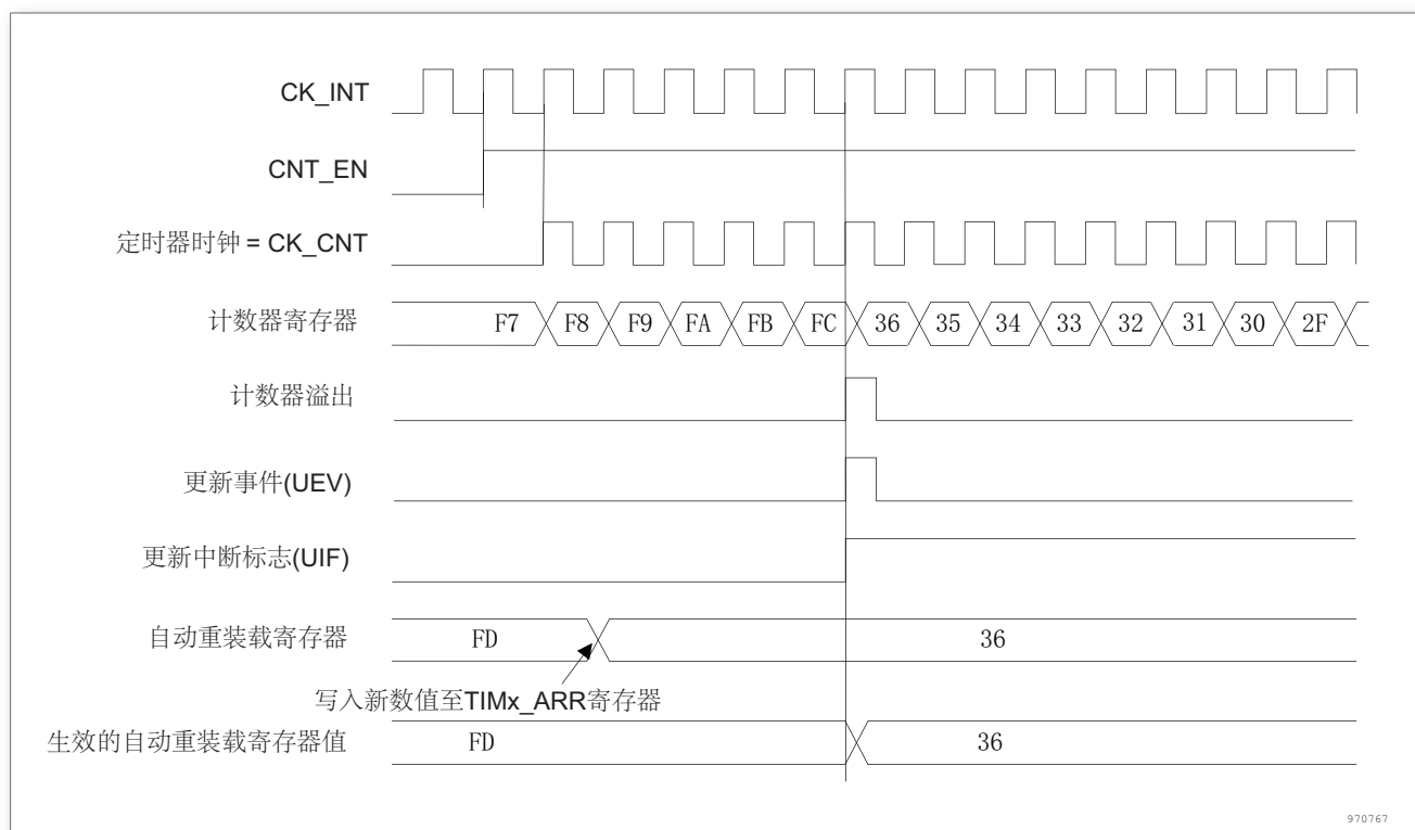
图 98. 计数器时序图, ARPE = 1 时的更新事件 (计数器溢出)
