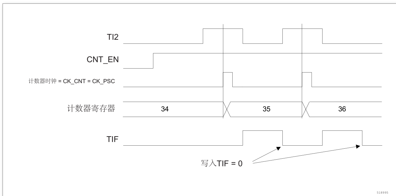
图 101. 外部时钟模式 1 下的控制电路
