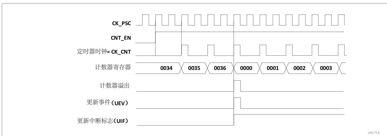
图 190. 计数器时序图，内部时钟分频因子为 2
