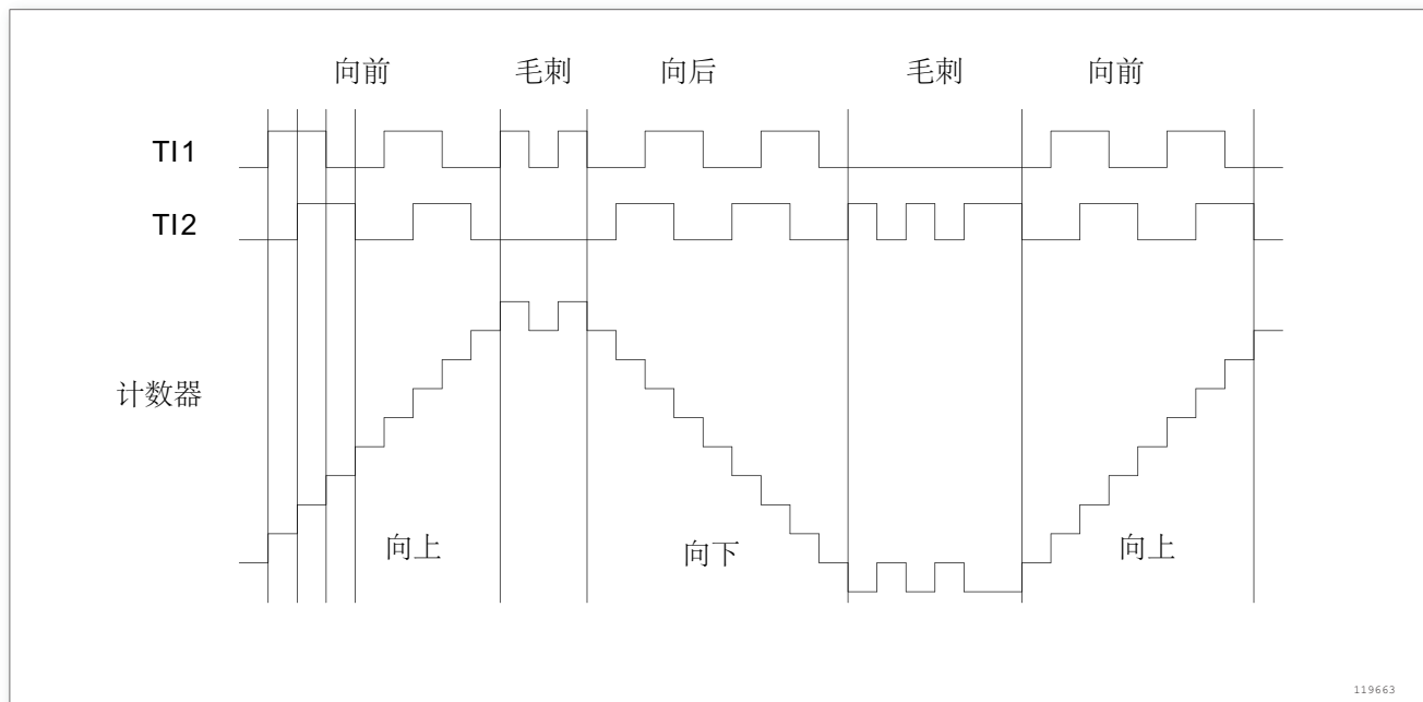
图 159. 编码器模式下的计数器操作实例
