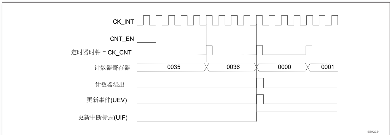
图 36. 计数器时序图，内部时钟分频因子为 4
