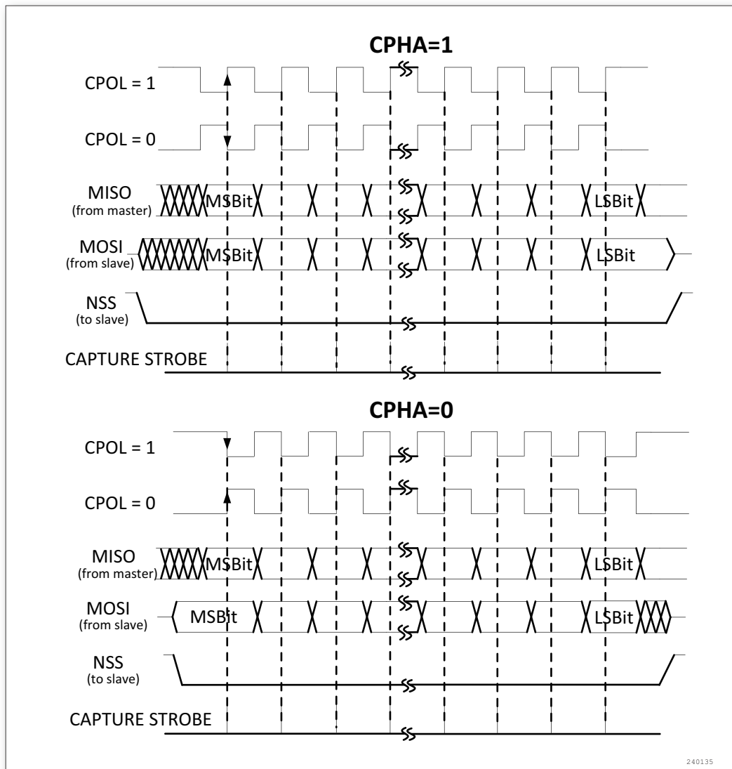
图 212. 数据时钟时序图
