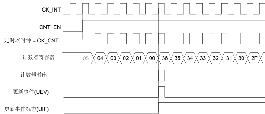
图 40. 计数器时序图，内部时钟分频因子为 1
