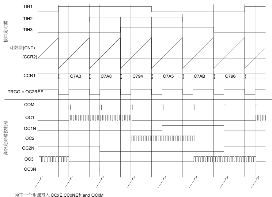
图 74. 霍尔传感器接口的实例
