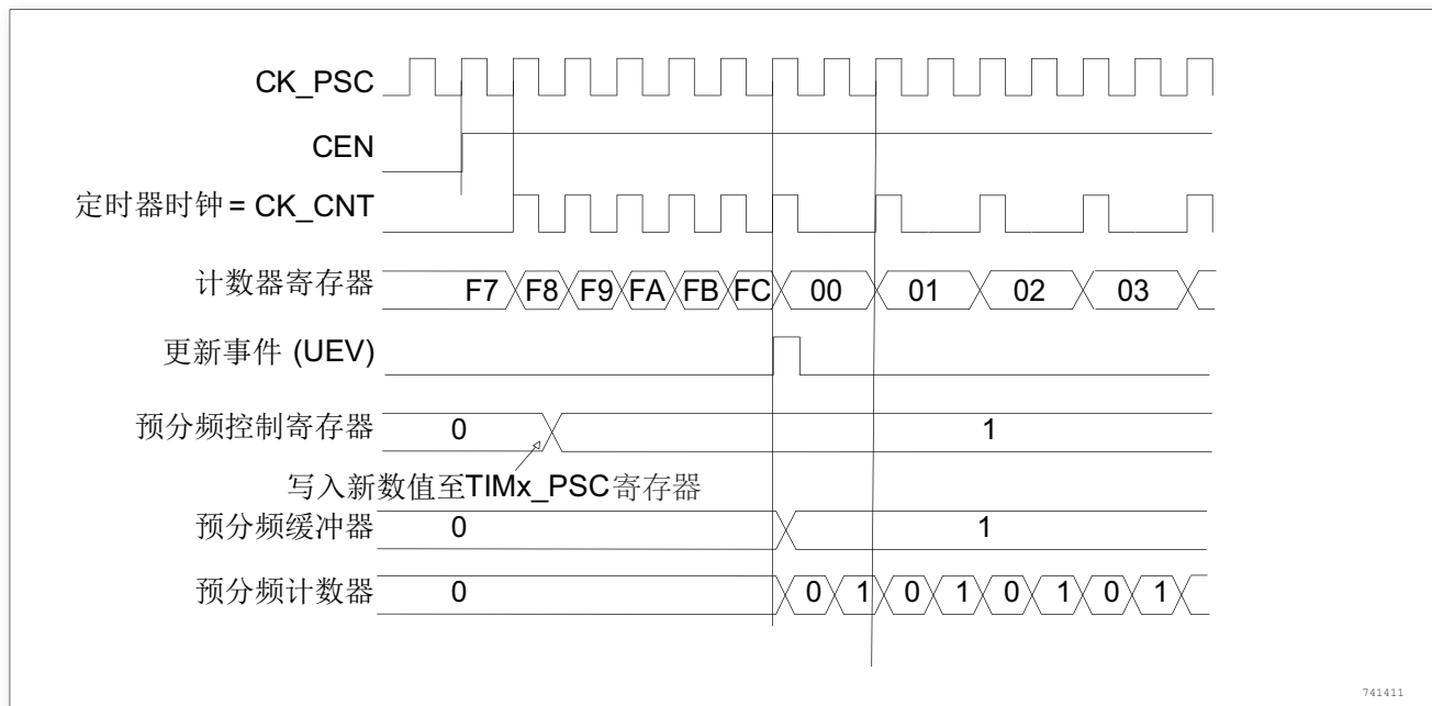
图 187. 当预分频器的参数从 1 变到 2 时, 计数器的时序图
