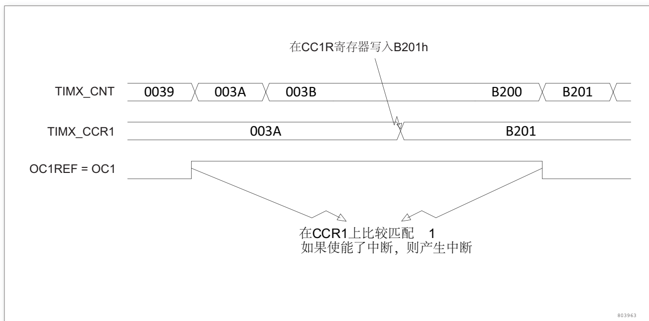
图 108. 输出比较模式，翻转 OC1
