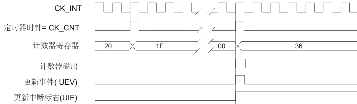
图 137. 计数器时序图，内部时钟分频因子为 N
