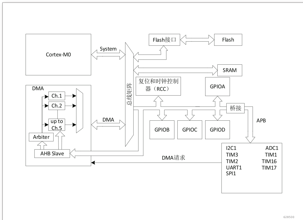
图 22. DMA 框图
