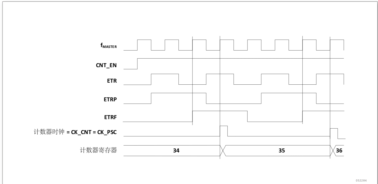
图 149. 外部时钟模式 2 下的控制电路
