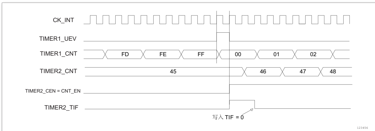
图 122. 使用定时器 1 的更新触发定时器 2
