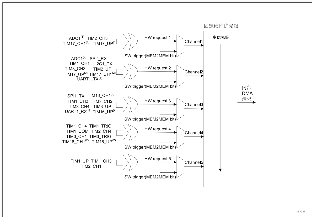
图 23. 外设 DMA 请求映射
