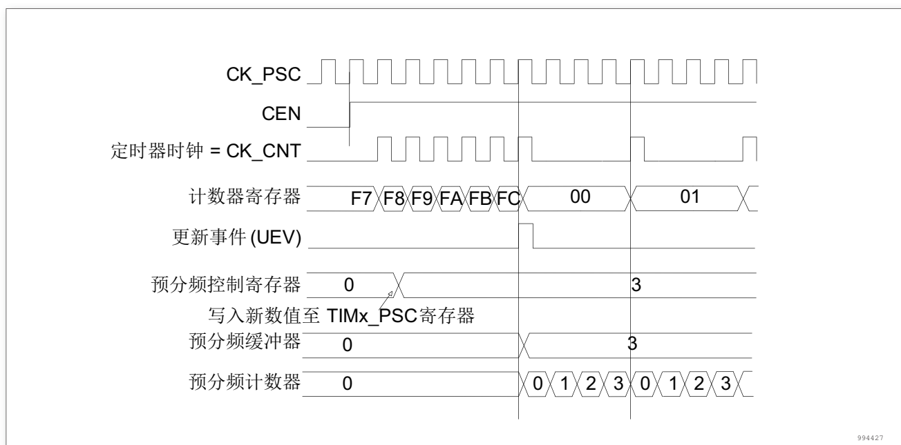
图 188. 当预分频器的参数从 1 变到 4 时, 计数器的时序图
