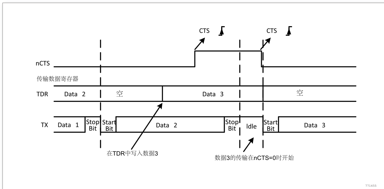
图 235. CTS 流控制
