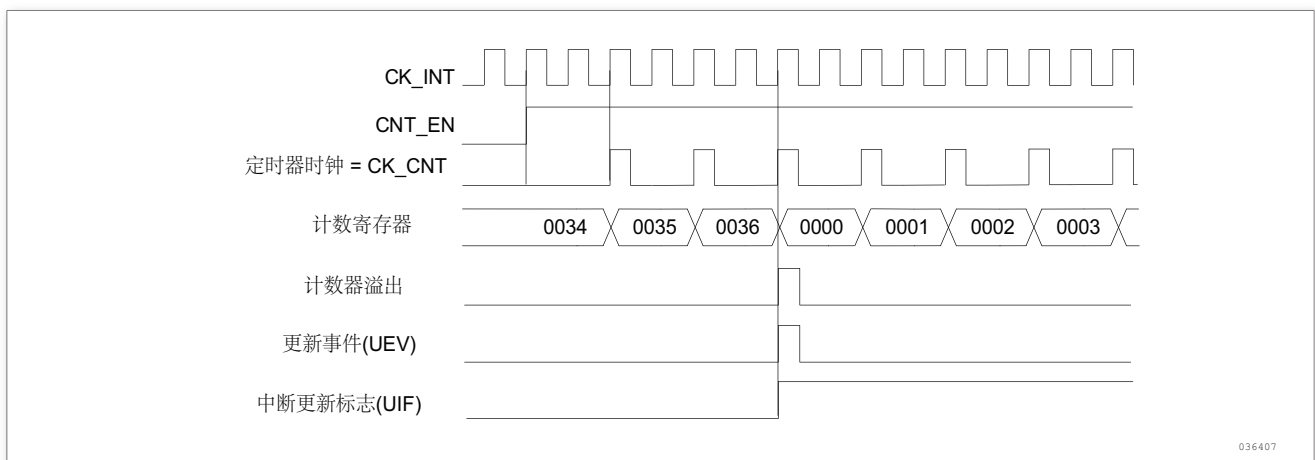
图 35. 计数器时序图，内部时钟分频因子为 2
