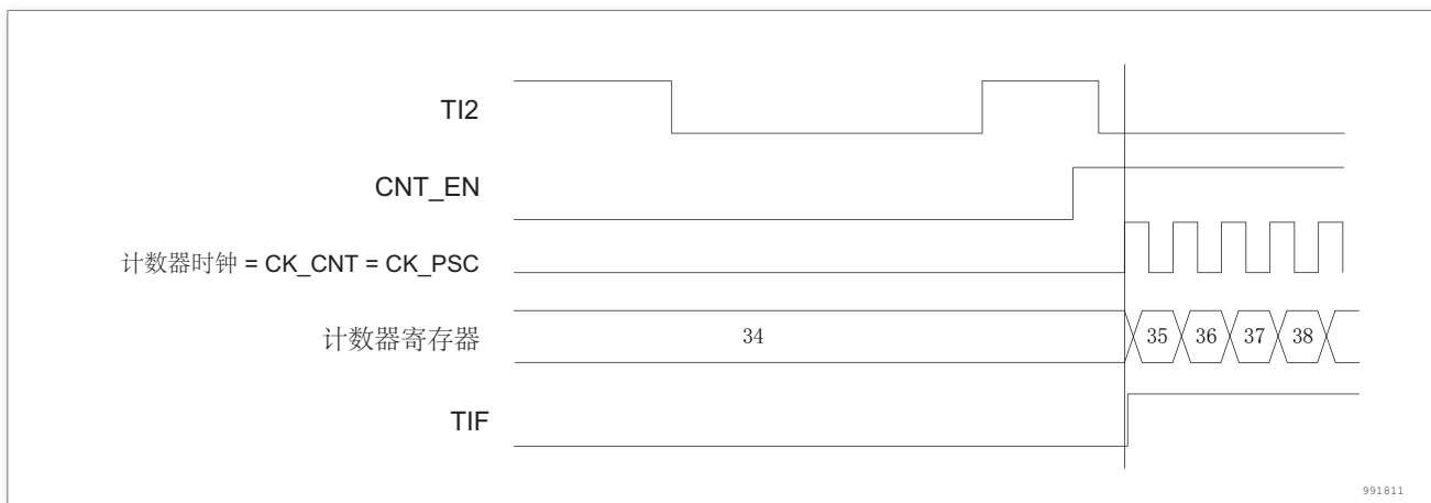
图 163. 触发器模式下的控制电路
