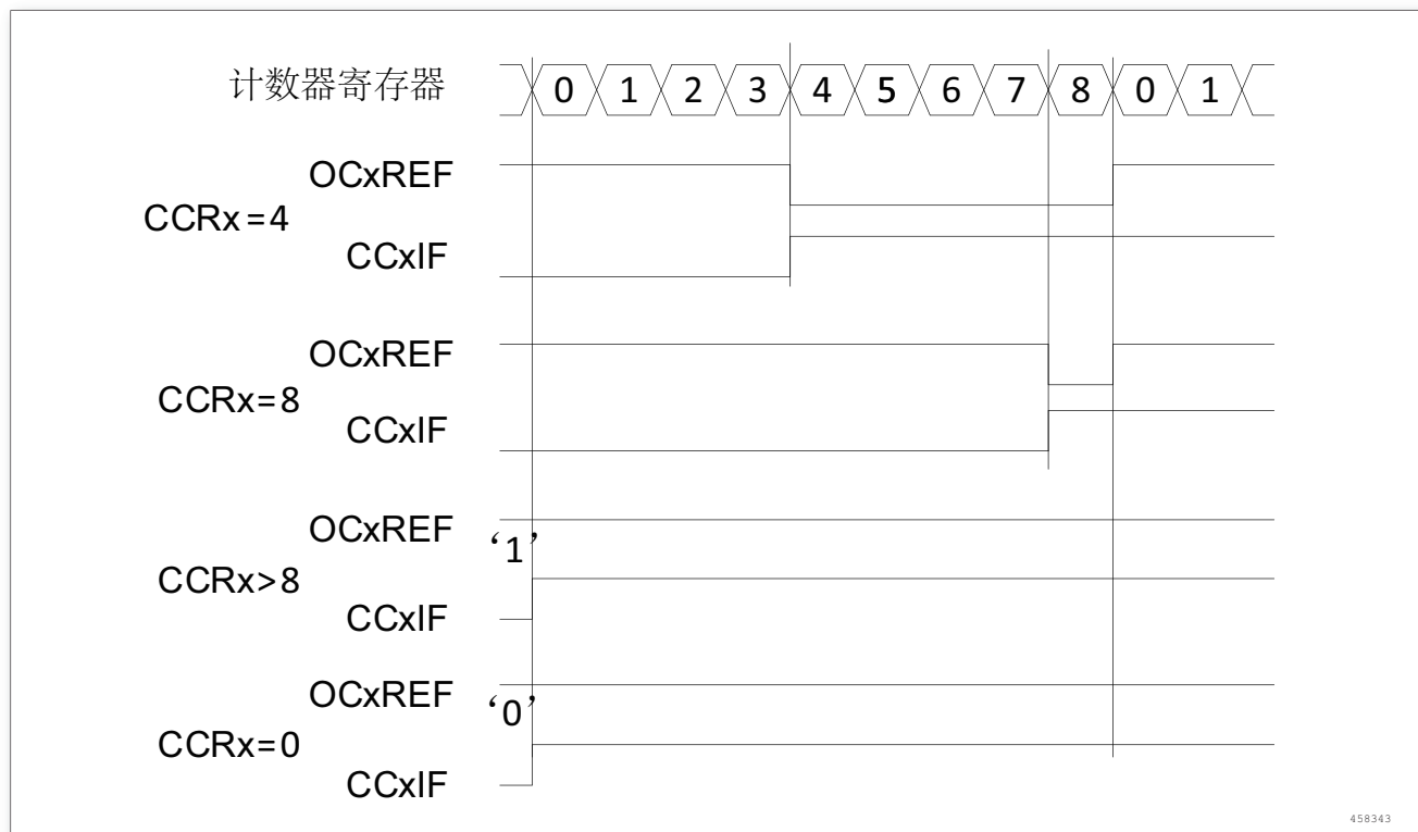
图 185. 边沿对齐的 PWM 波形 (ARR = 8)
