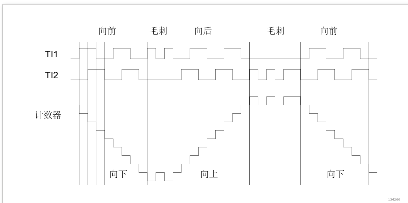
图 73. IC1FP1 反相的编码器接口模式实例
