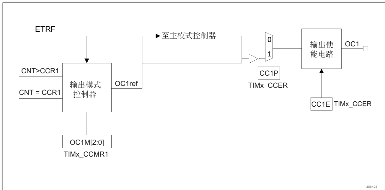
图 183. 捕获/比较通道的输出部分 (通道 1)
