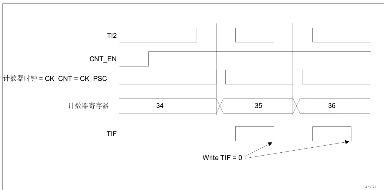
图 54. 外部时钟模式 1 下的控制电路
