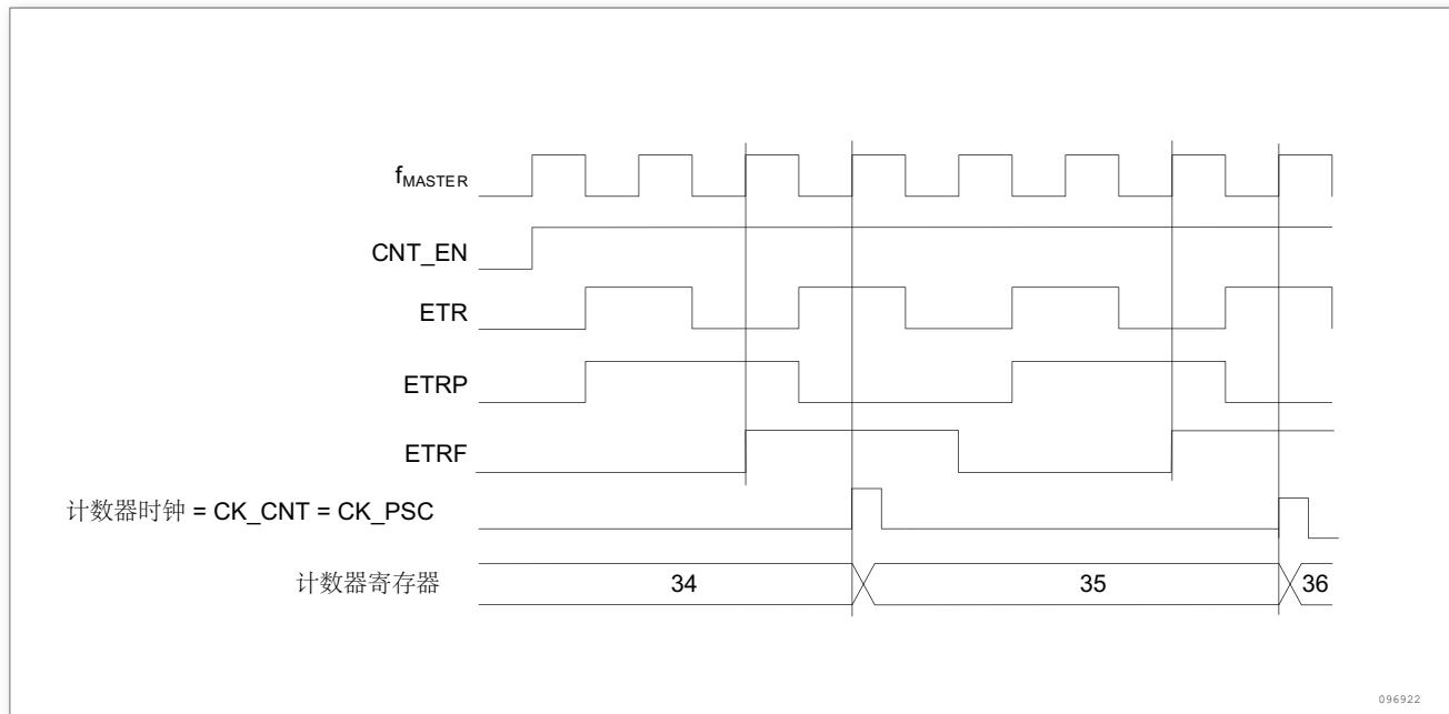
图 56. 外部时钟模式 2 下的控制电路
