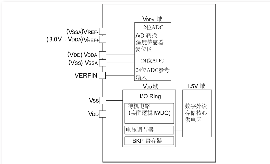
图 7. 电源框图
