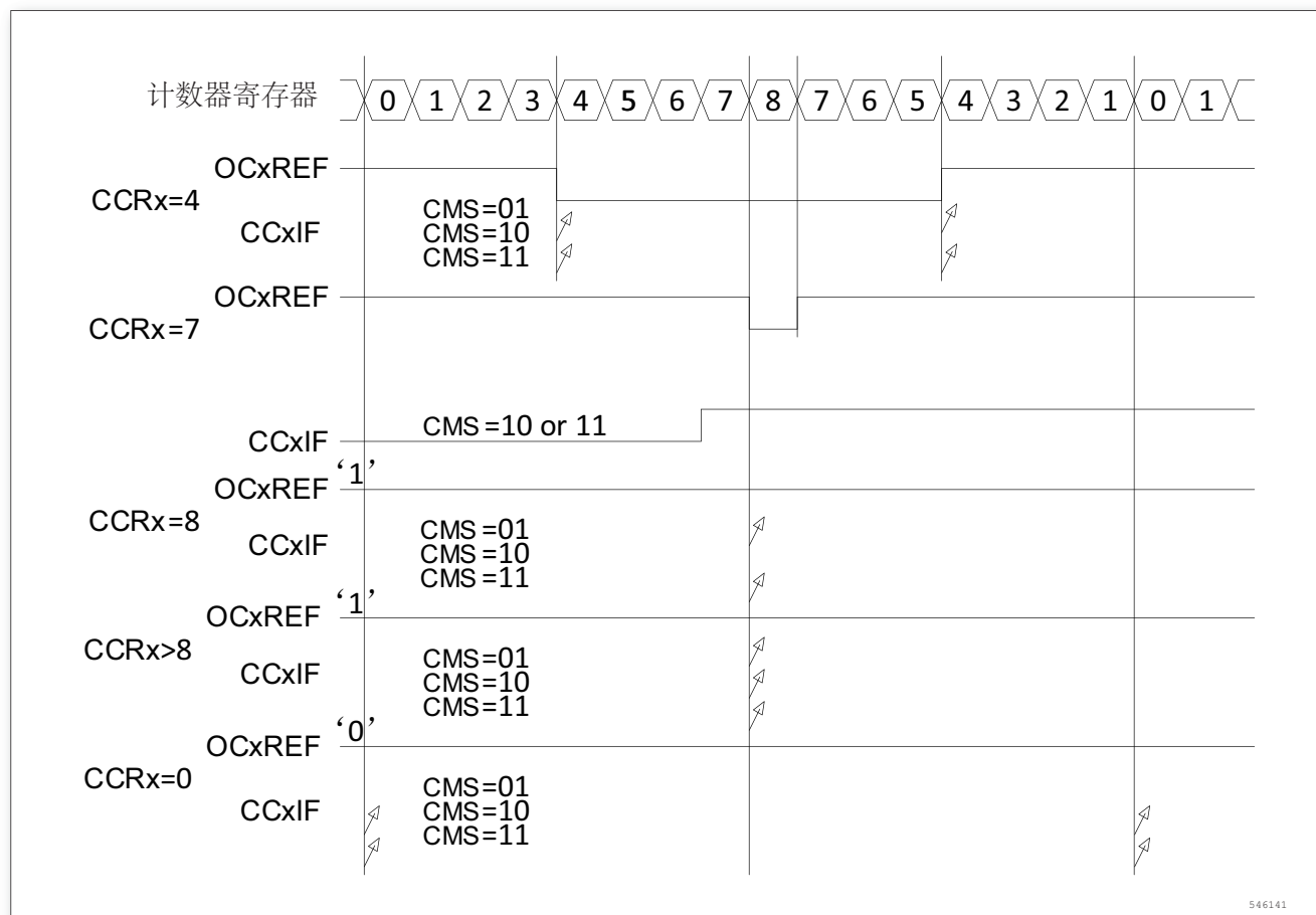
图 110. 中央对齐的 PWM 波形 (APR = 8)
