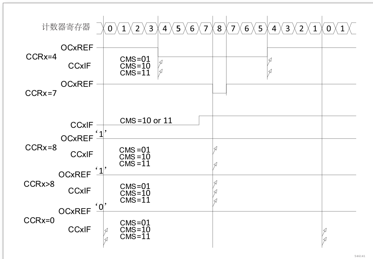
图 156. 中央对齐的 PWM 波形 (APR = 8)
