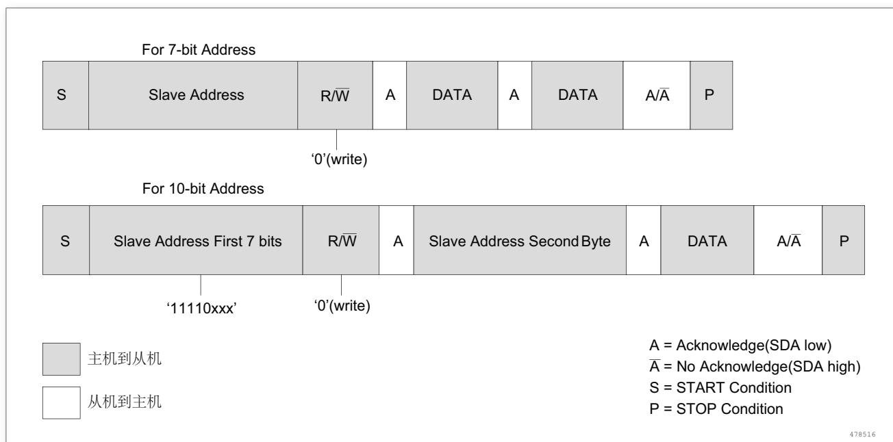
图 216. 主发送协议
