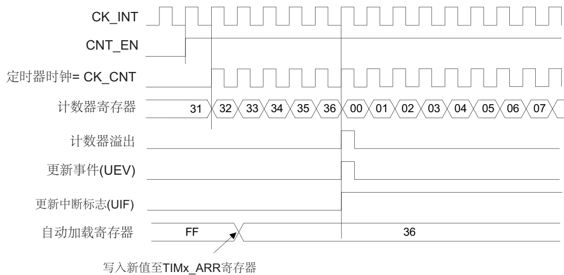
图 132. 计数器时序图, 当 ARPE = 0 时的更新事件 (TIMx_ARR 没有预装入)
