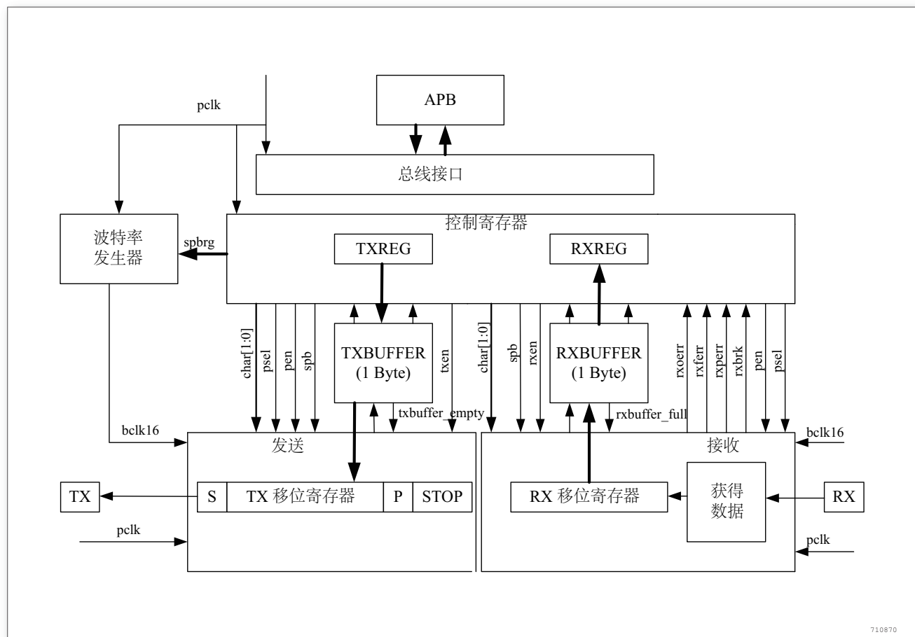
图 227. UART 方框图
