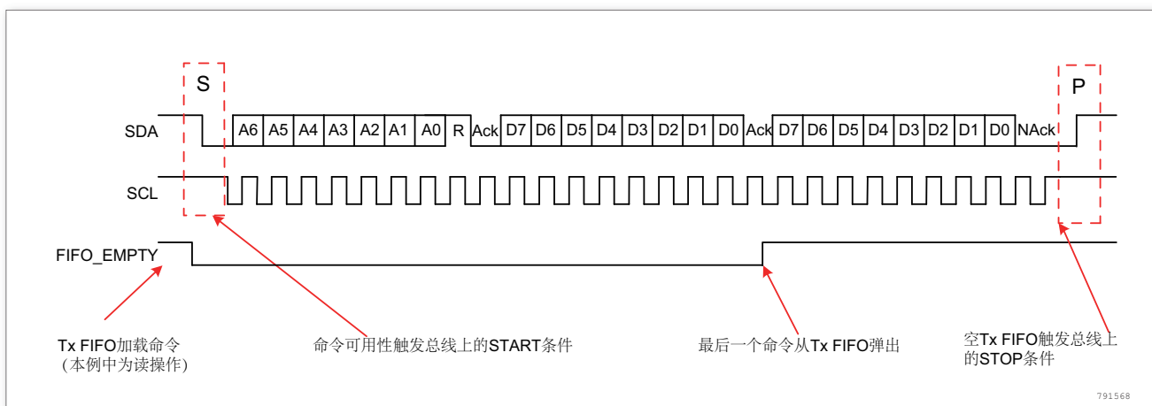
图 221. 主接收 - Tx FIFO 为空
