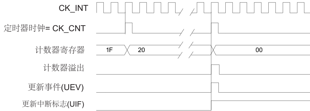
图 131. 计数器时序图, 内部时钟分频因子为 N
