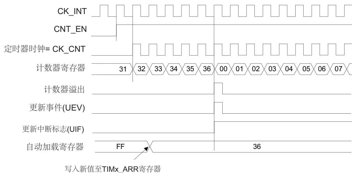
图 86. 计数器时序图，当 ARPE = 0 时的更新事件 (TIMx_ARR 没有预装入)
