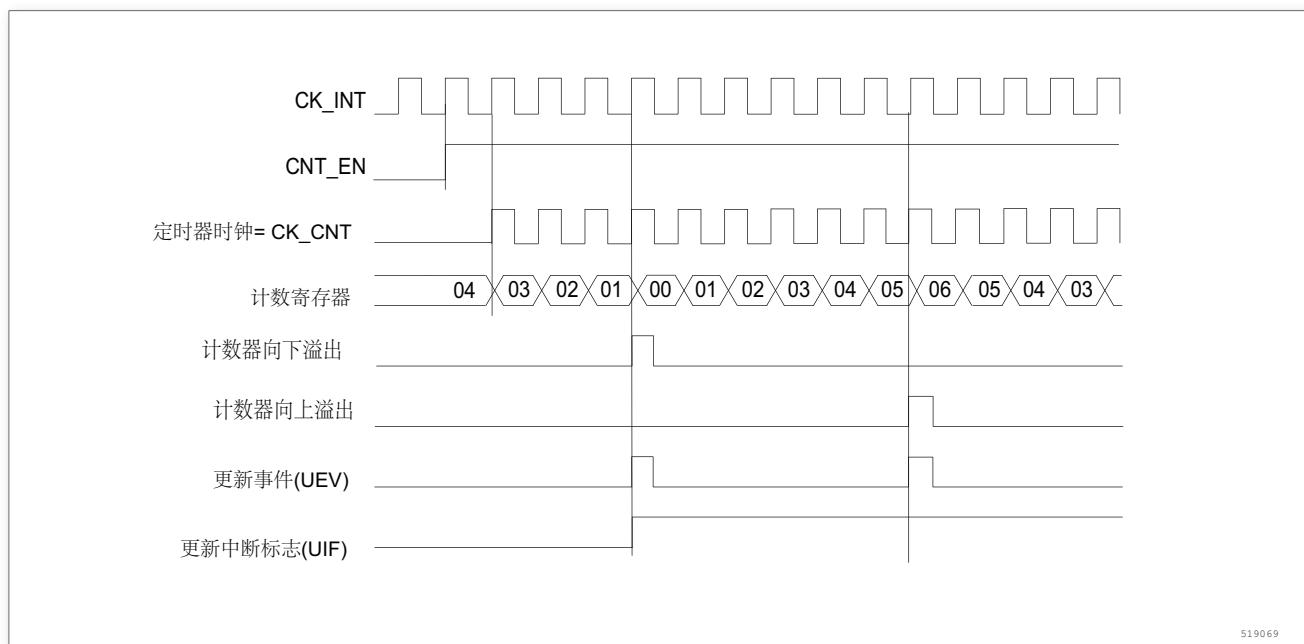
图 45. 计数器时序图，内部时钟分频因子为 1，TIMx_ARR = 0x6
