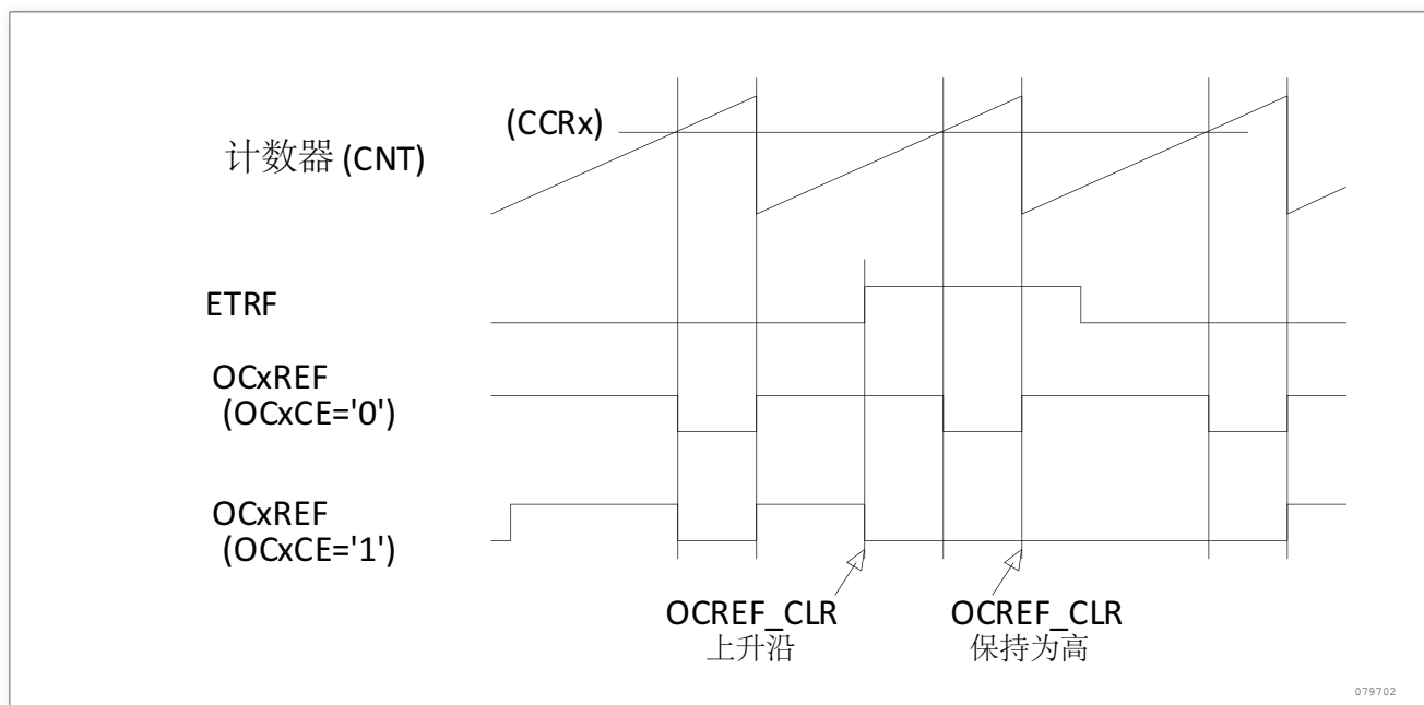
图 158. 清除 TIMx 的 OCxREF
