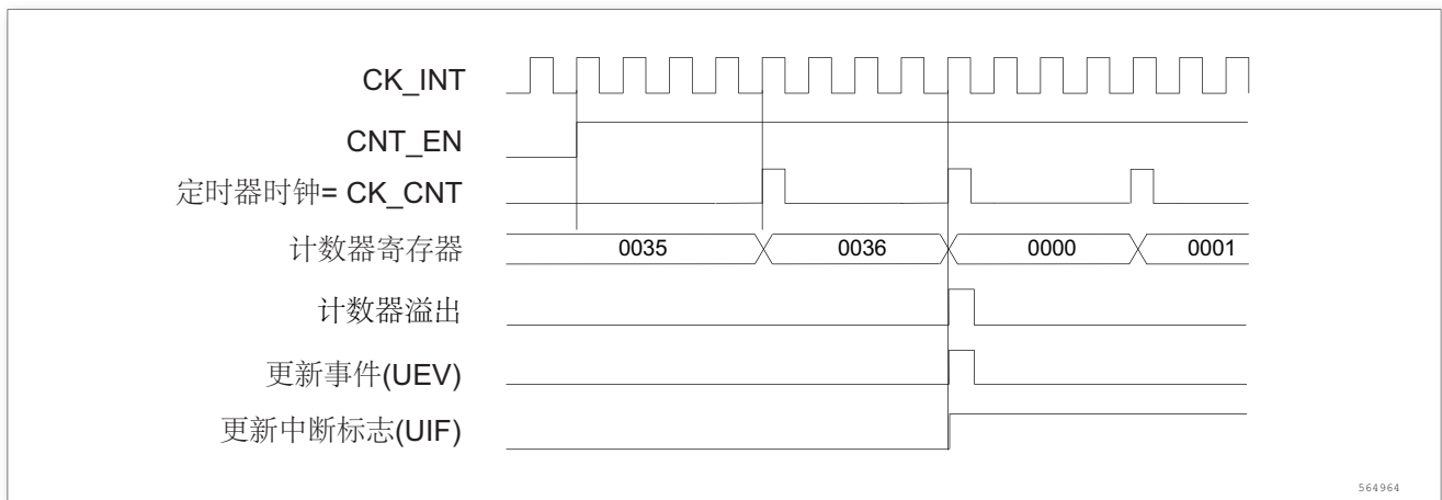
图 176. 计数器时序图，内部时钟分频因子为 4
