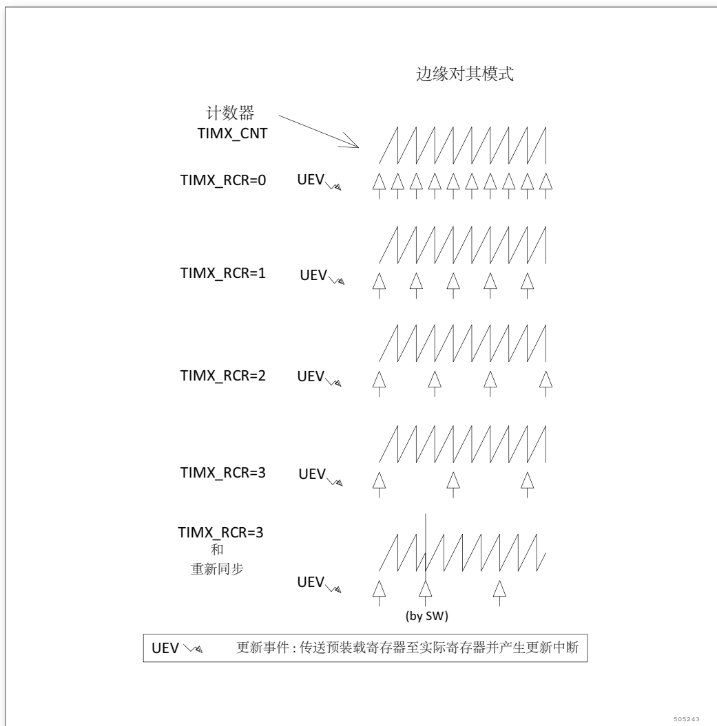
图 195. 不同模式及不同 TIMx_RCR 寄存器设置下更新速率的例子
