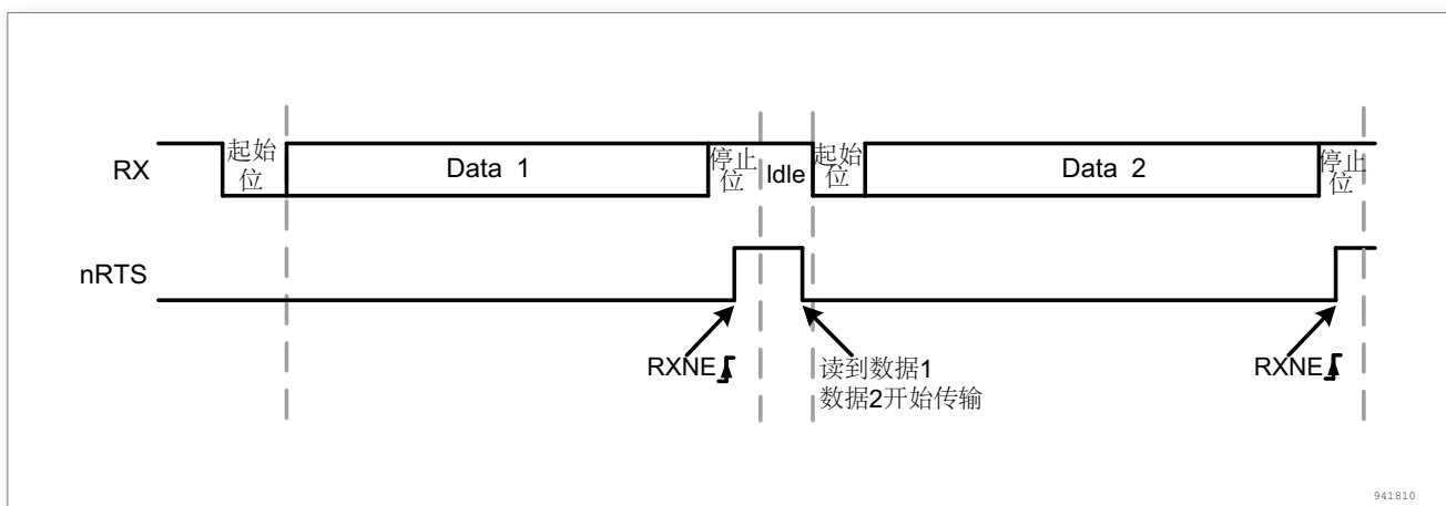
图 234. RTS 流控制
