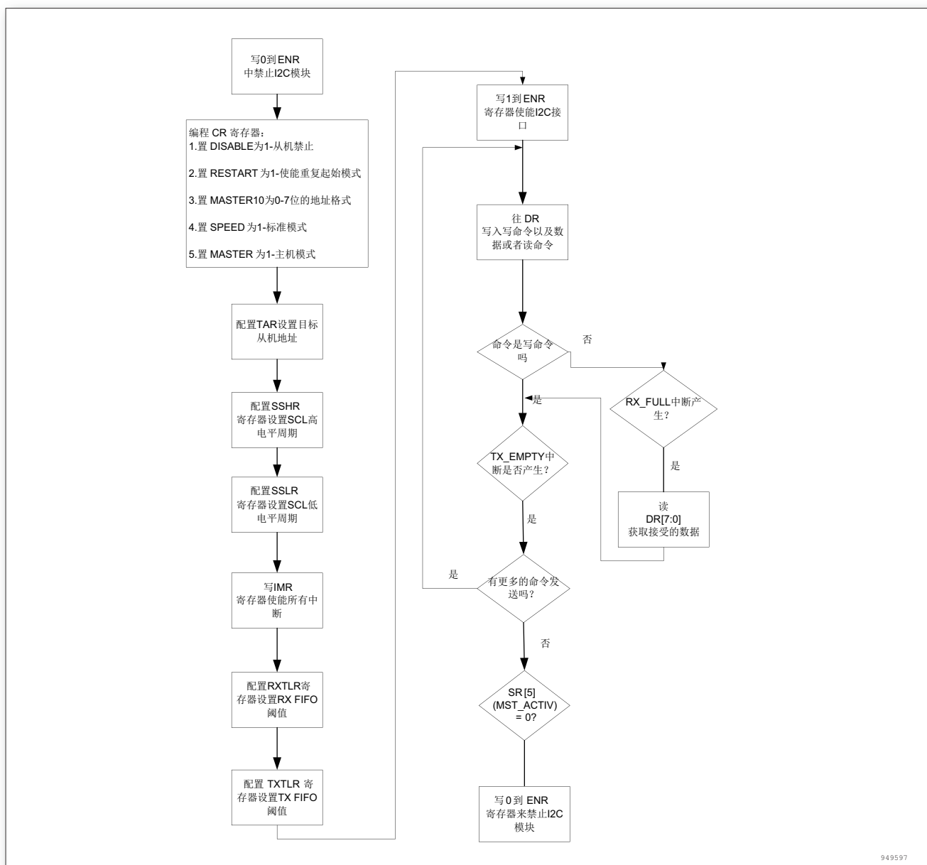
图 225. I 2 C 接口主机流程图
