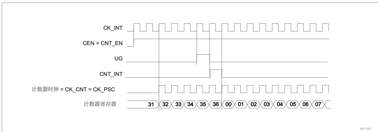
图 52. 一般模式下的控制电路，内部时钟分频因子为 1
