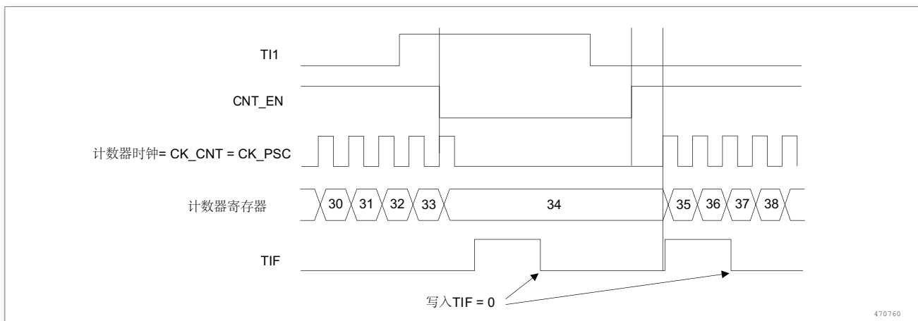
图 76. 门控模式下的控制电路
