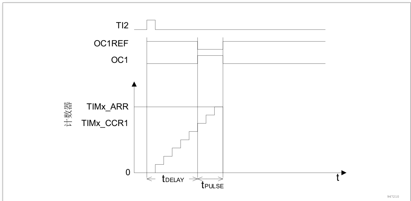
图 71. 单脉冲模式的例子
