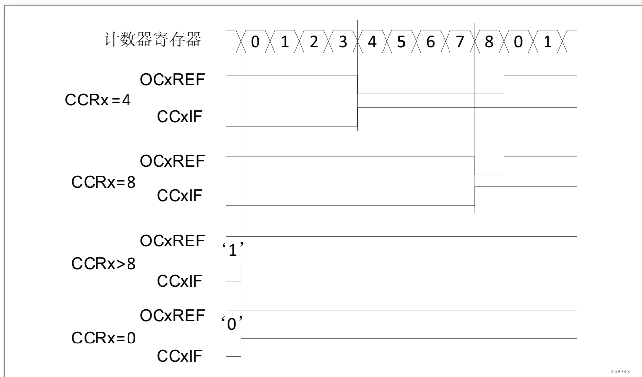
图 155. 边沿对齐的 PWM 波形 (ARR = 8)
