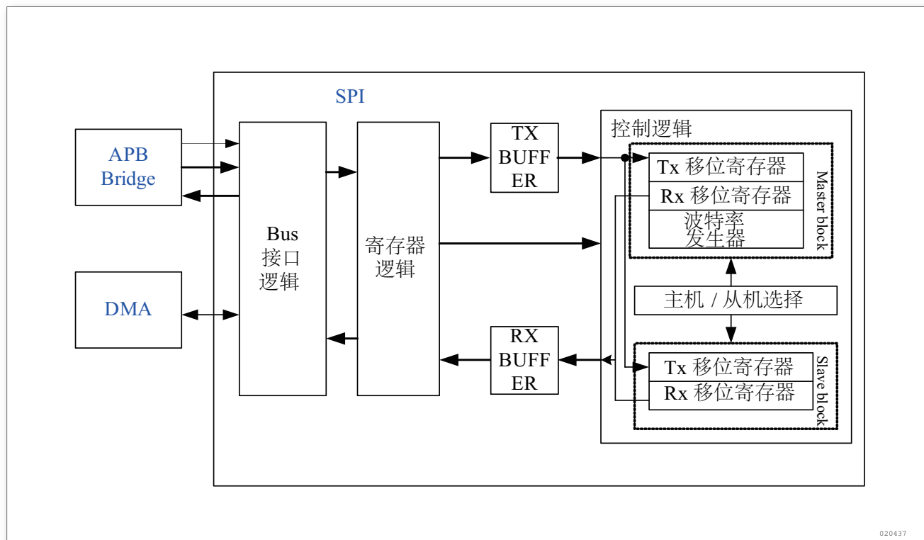
图 210. SPI 框图
