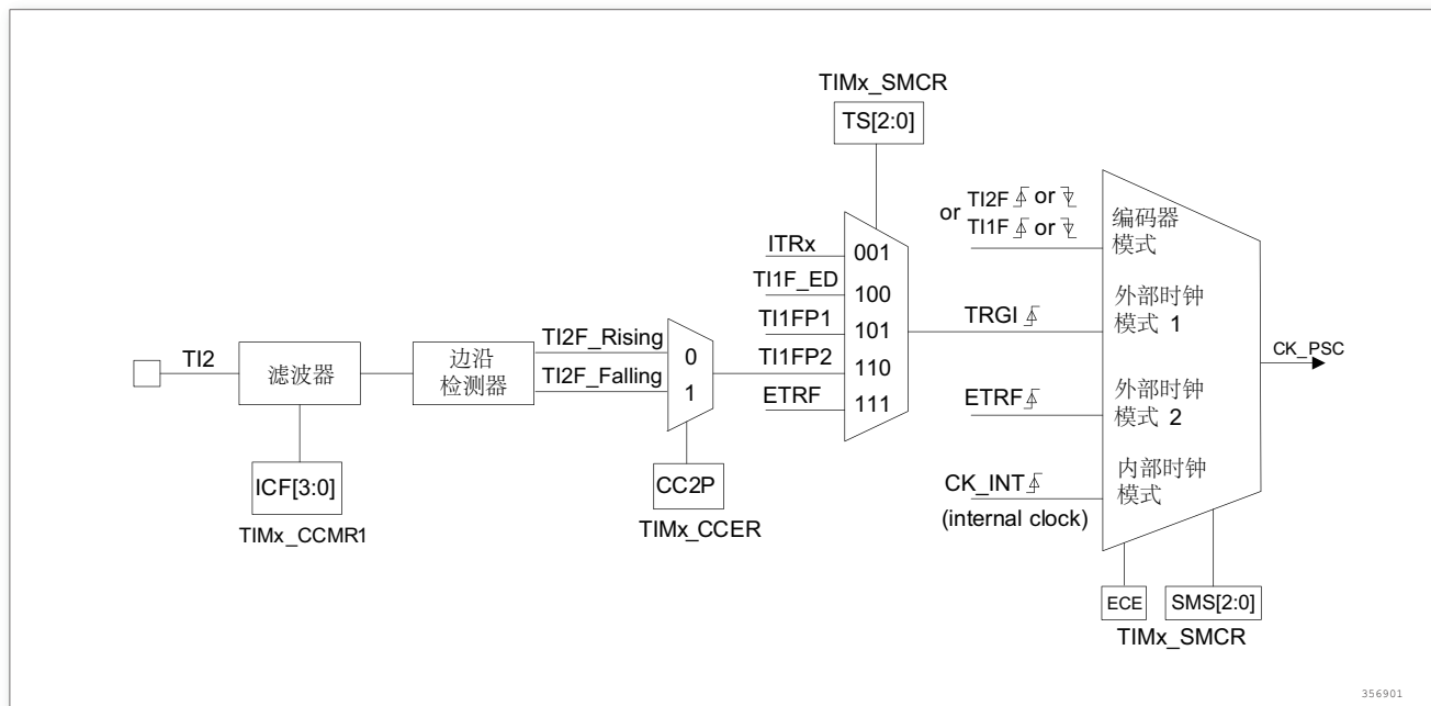
图 100. TI2 外部时钟连接例子
