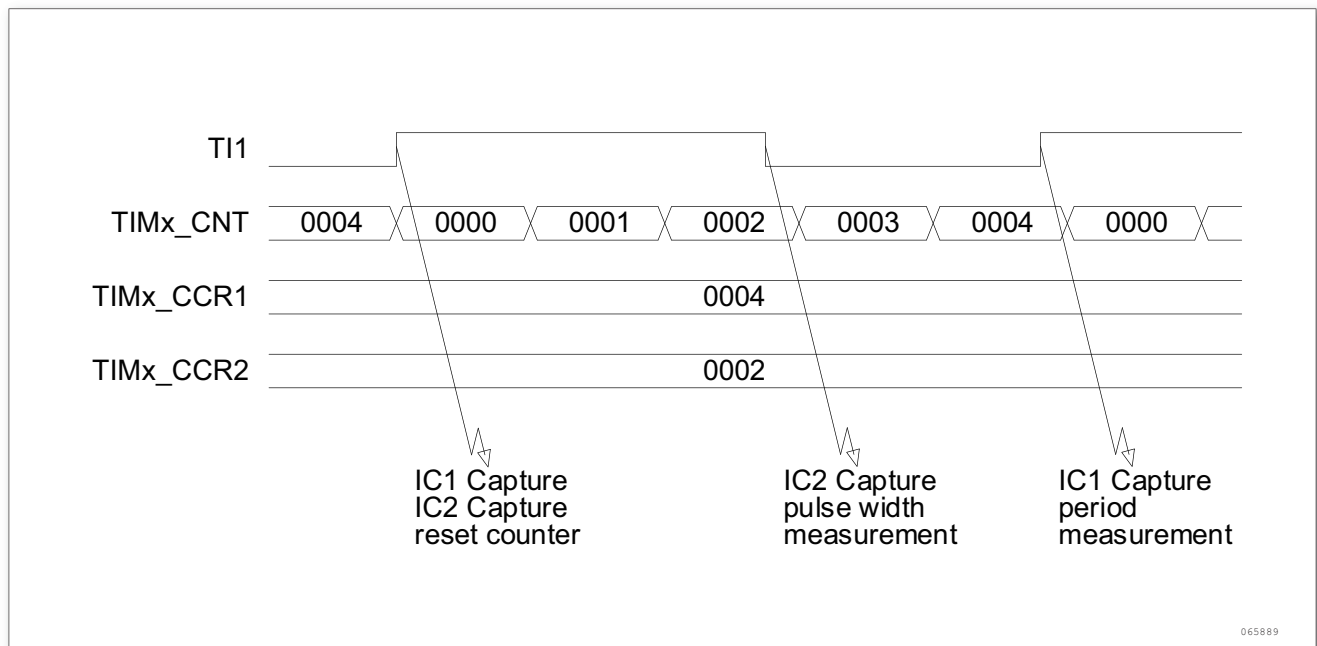
图 61. PWM 输入模式时序
