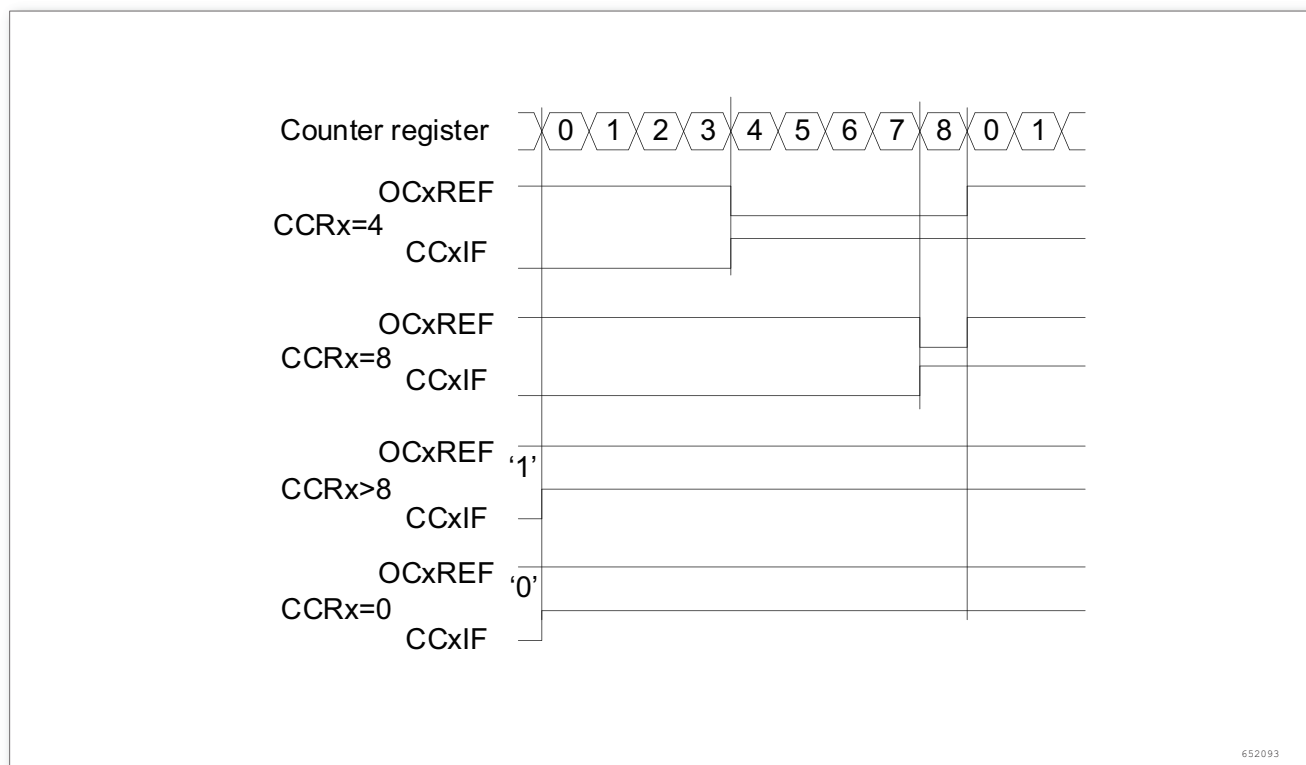
图 63. 边沿对齐的 PWM 波形 (ARR = 8)
