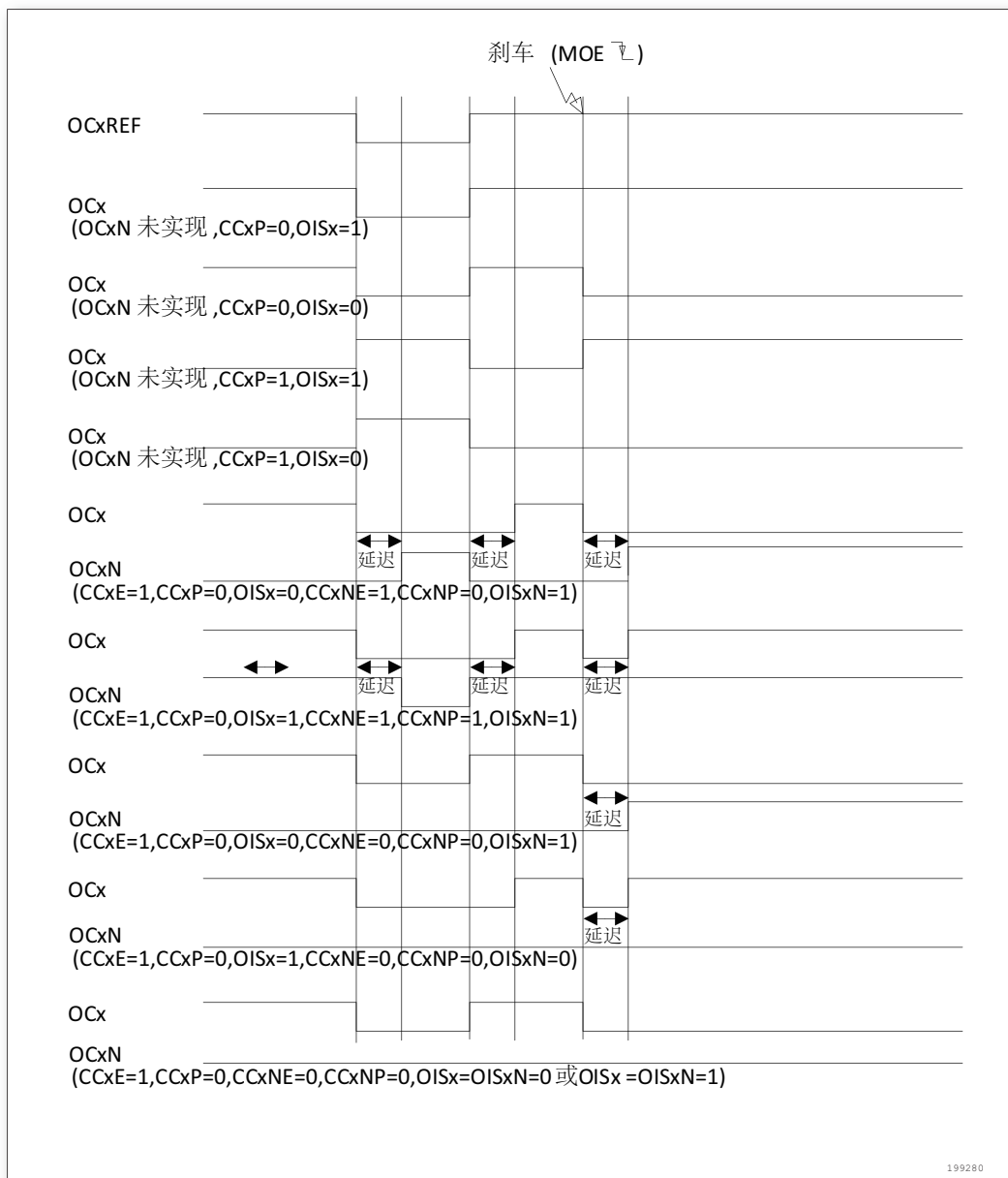
图 205. 响应刹车的输出
