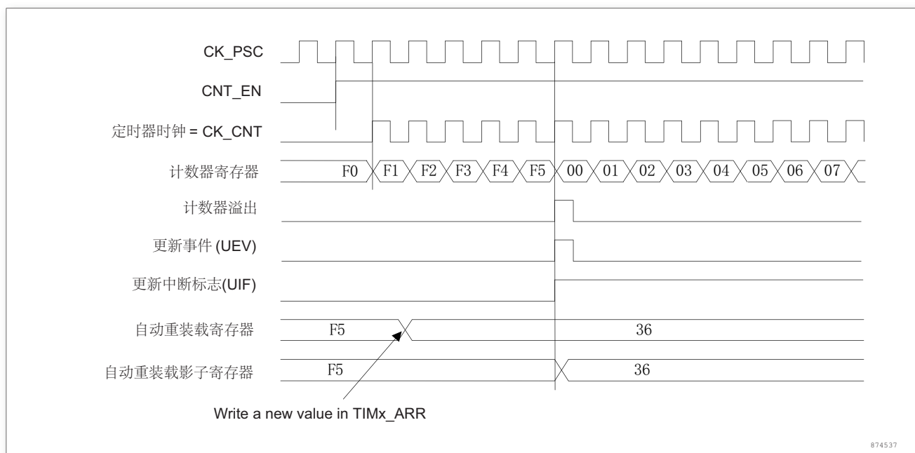
图 179. 计数器时序图，当 ARPE = 1 时的更新事件 (预装入了 TIM14_ARR)
