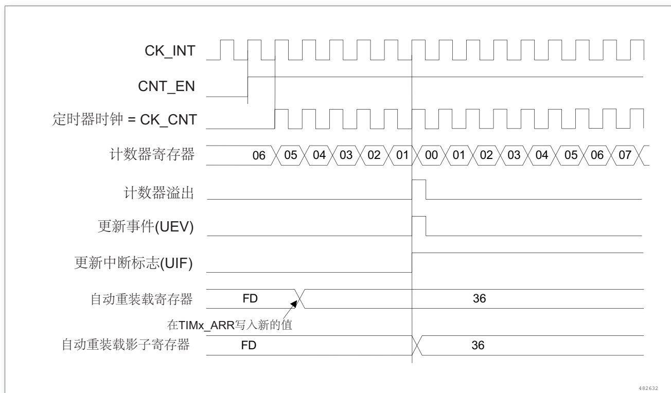
图 143. 计数器时序图, ARPE = 1 时的更新事件 (计数器下溢)
