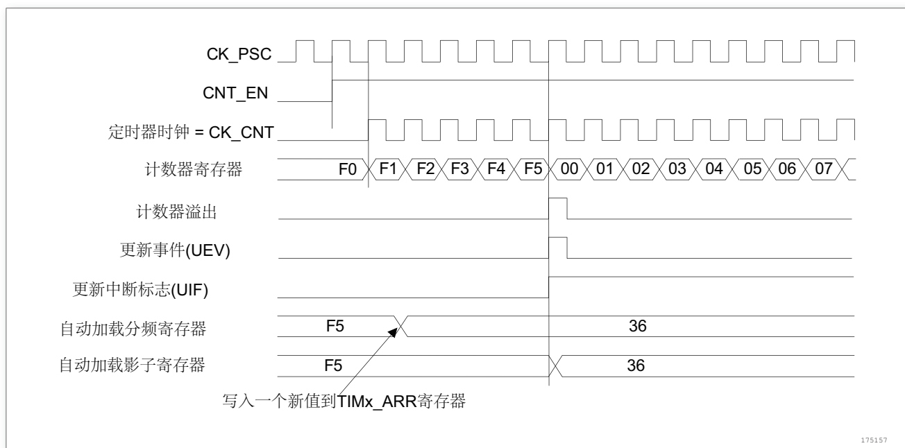
图 39. 计数器时序图，当 ARPE = 1 时的更新事件 (预装入了 TIMx_ARR)
