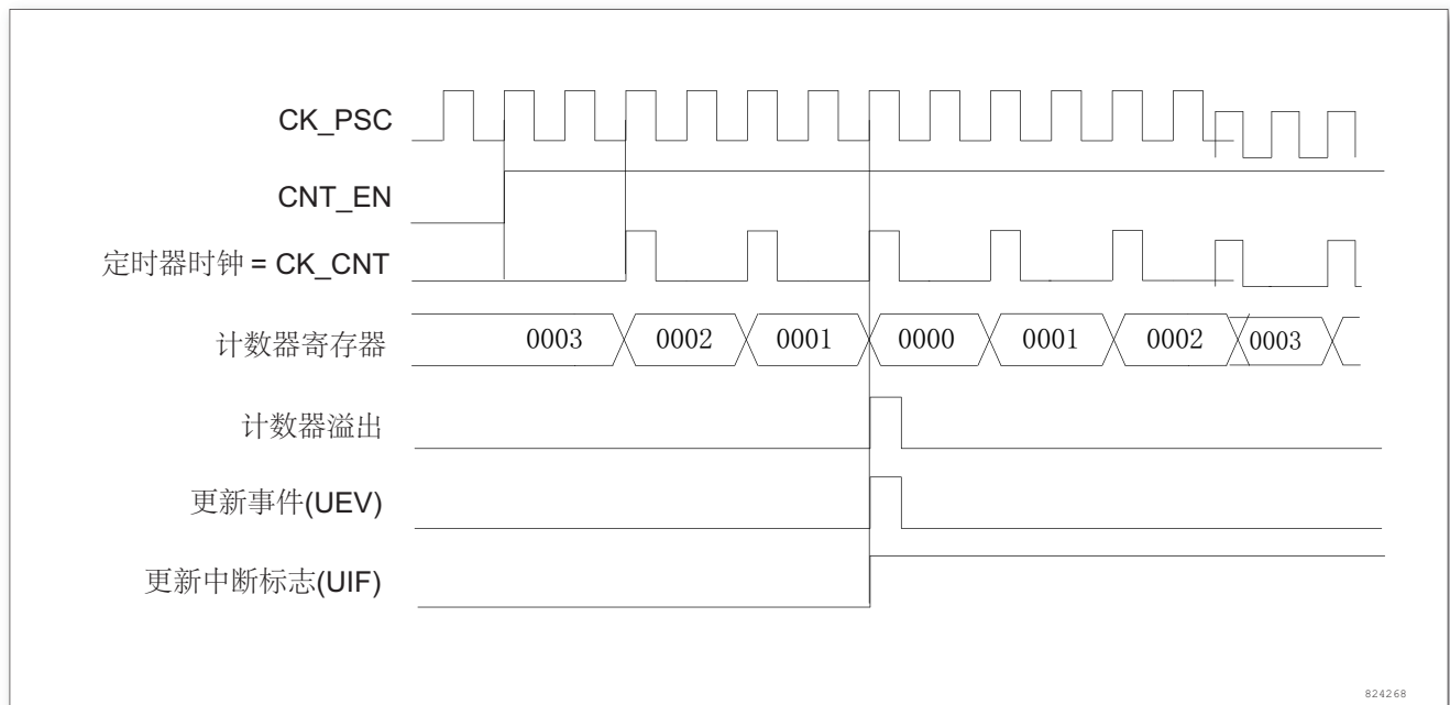
图 94. 计数器时序图，内部时钟分频因子为 2
