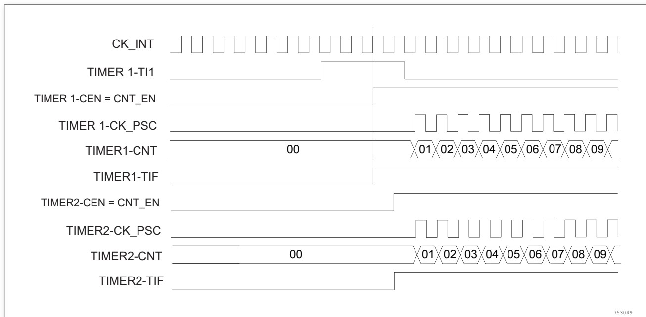
图 170. 使用定时器 1 的 TI1 输入触发定时器 1 和定时器 2
