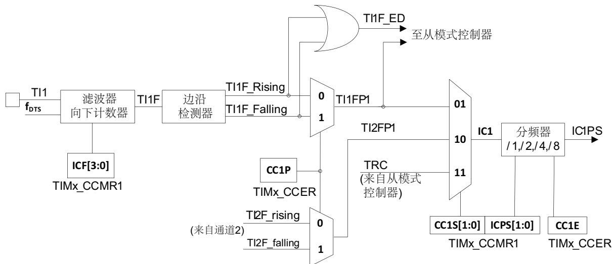
图 104. 捕获/比较通道 (如: 通道 1 输入部分)
