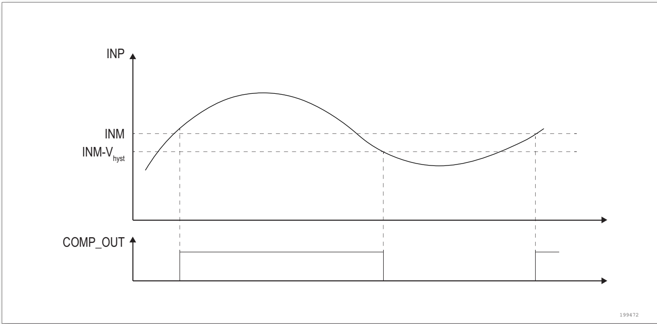
图 30. 比较器的迟滞现象
