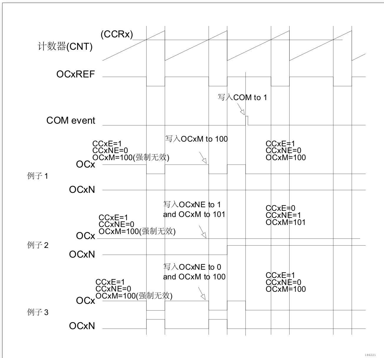
图 70. 产生六步 PWM，使用 COM 的例子 (OSSR = 1)
