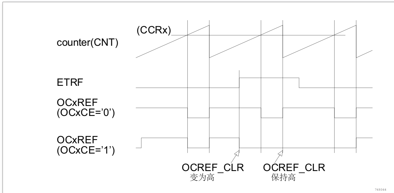
图 69. 清除 TIMx 的 OCxREF
