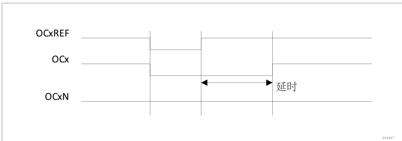
图 203. 死区波形延迟大于负脉冲
