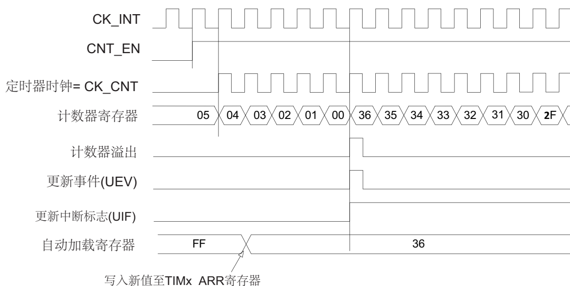
图 138. 计数器时序图，当没有使用重复计数器时的更新事件
