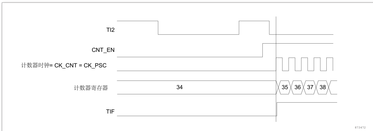
图 77. 触发器模式下的控制电路
