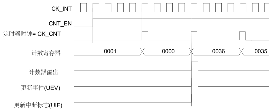
图 42. 计数器时序图，内部时钟分频因子为 4
