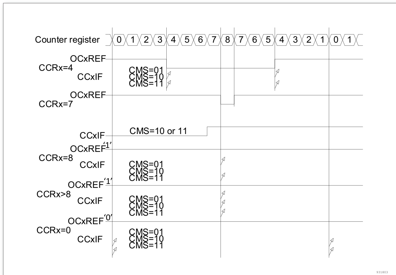
图 64. 中央对齐的 PWM 波形 (APR = 8)
