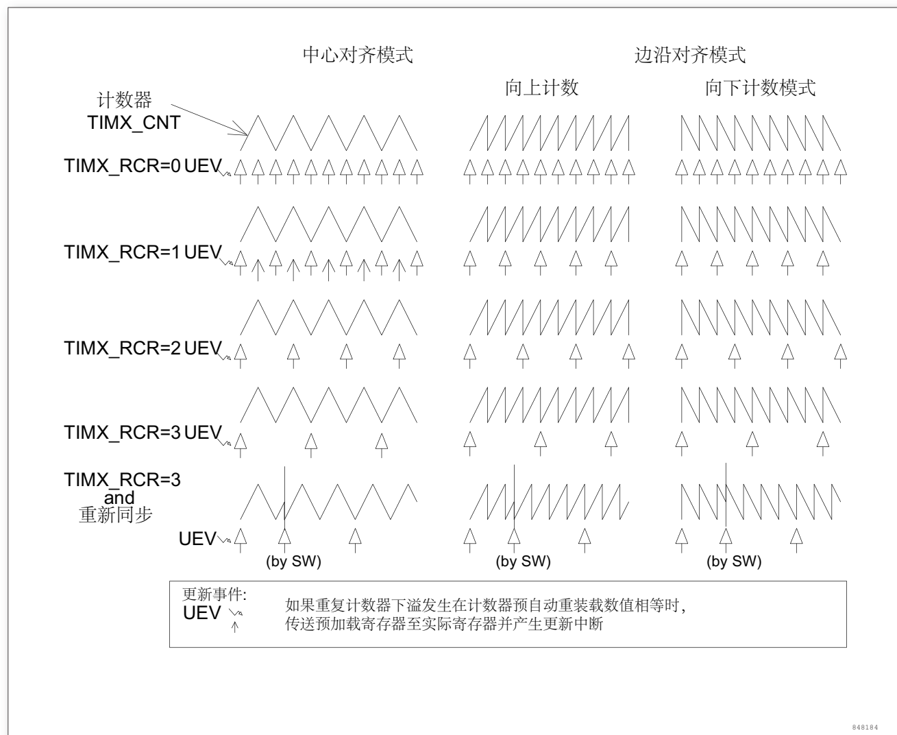
图 51. 不同模式下更新速率的例子，及 TIMx_RCR 的寄存器设置
