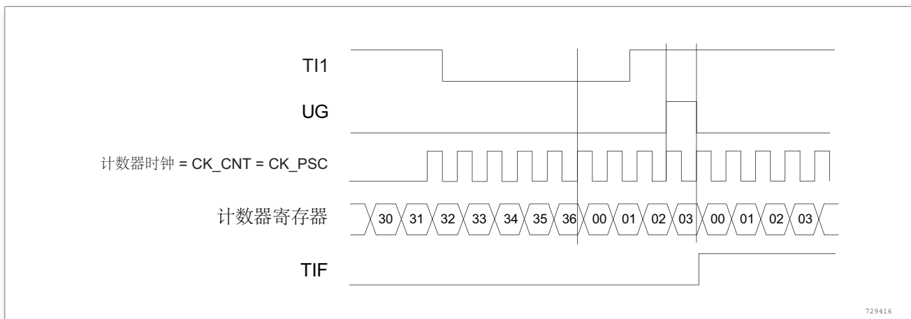
图 161. 复位模式下的控制电路
