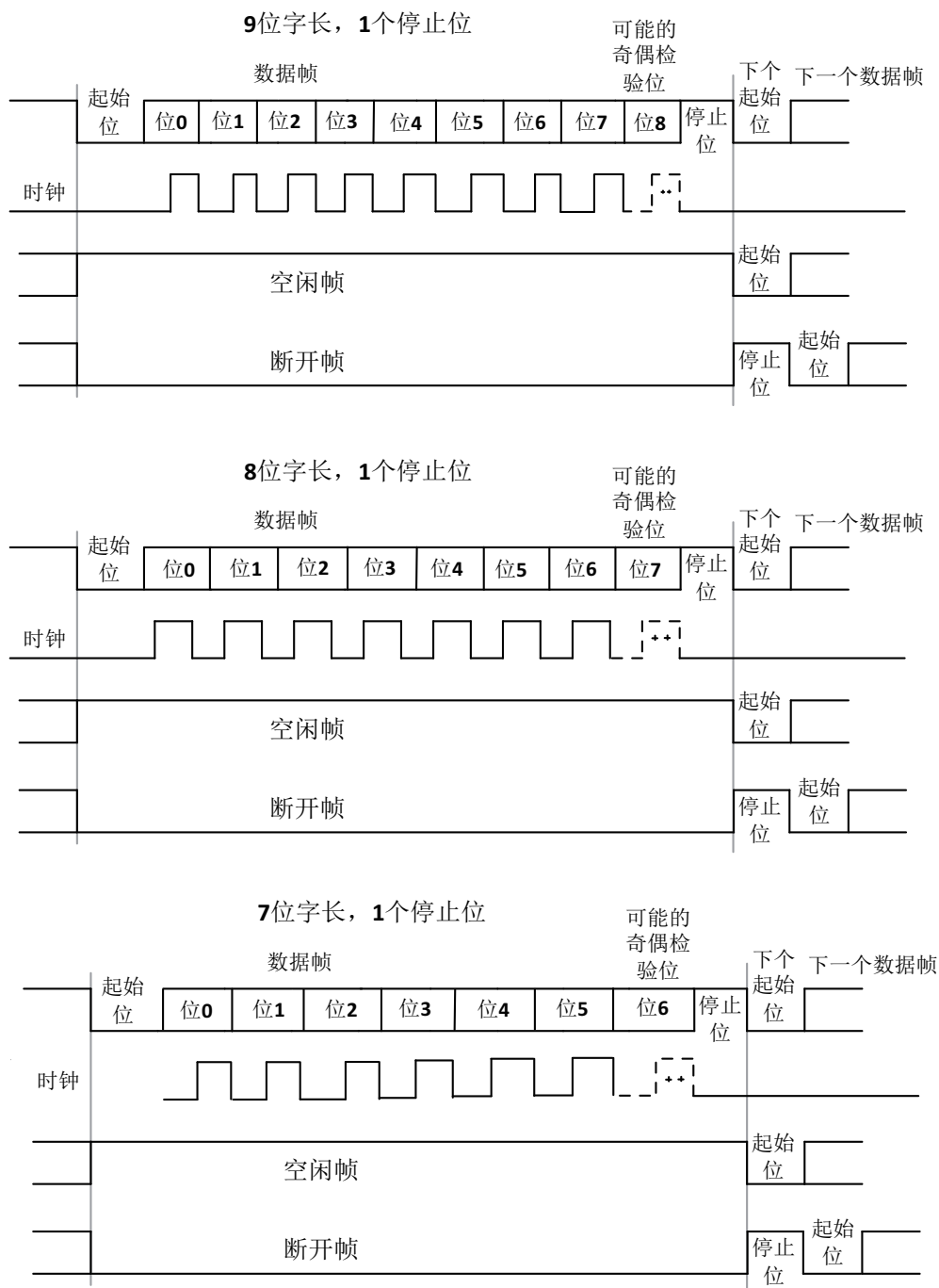
图 228. UART 时序
