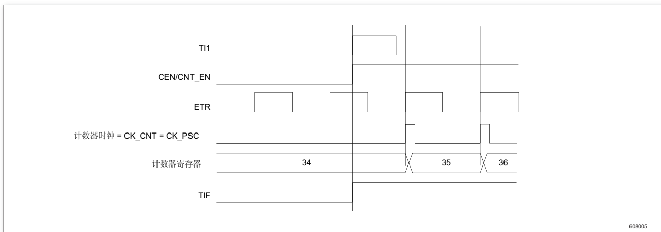
图 78. 外部时钟模式 2 + 触发模式下的控制电路
