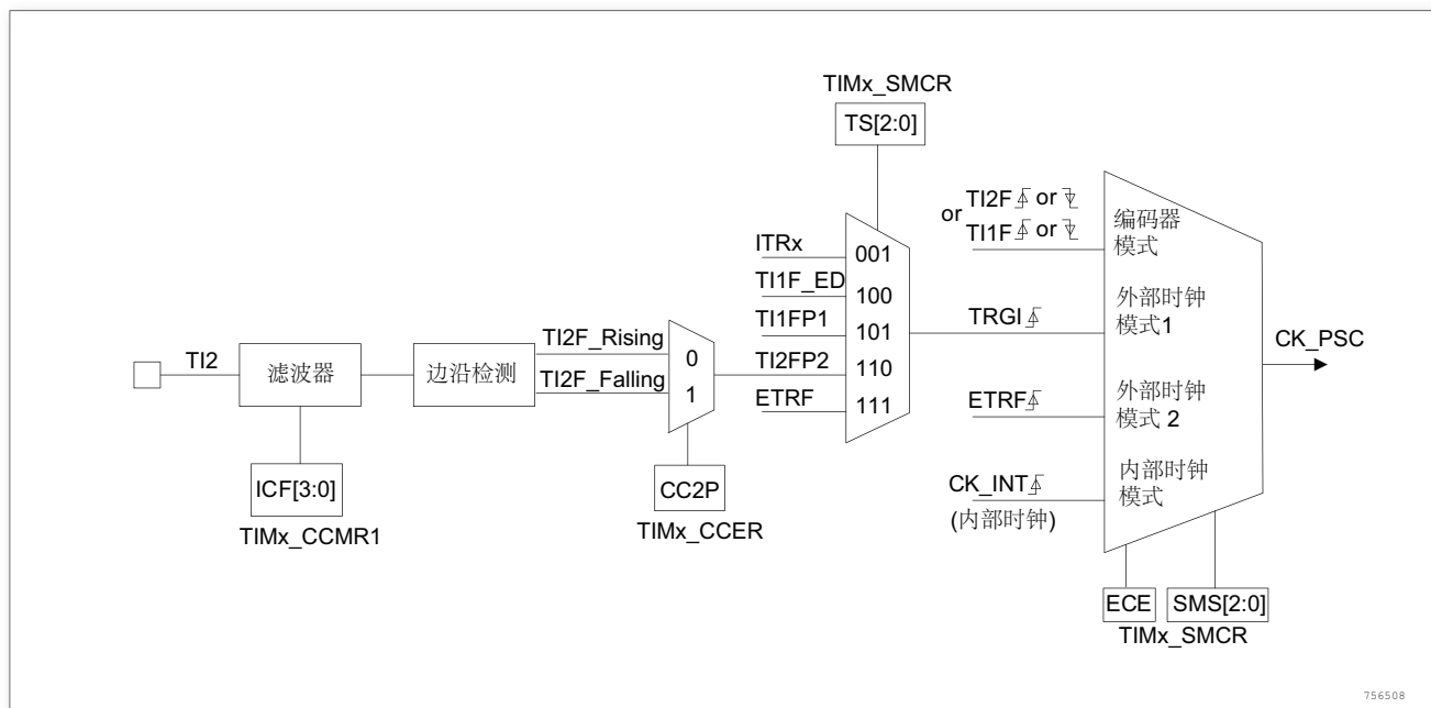
图 53. TI2 外部时钟连接例子
