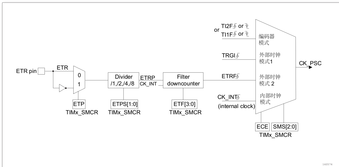
图 55. 外部触发输入框图
