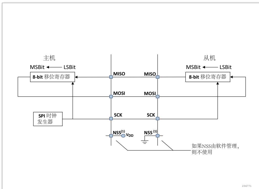
图 211. 单主和单从应用
