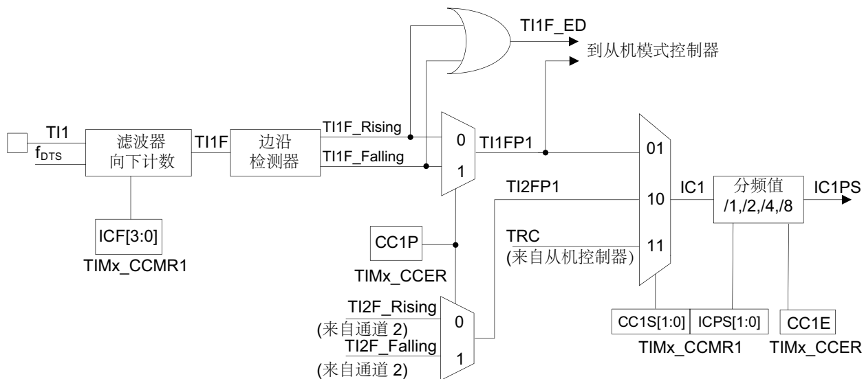
图 57. 捕获/比较通道 (如: 通道 1 输入部分)
