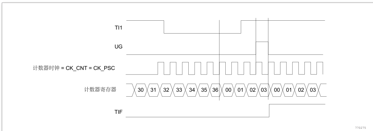
图 75. 复位模式下的控制电路
