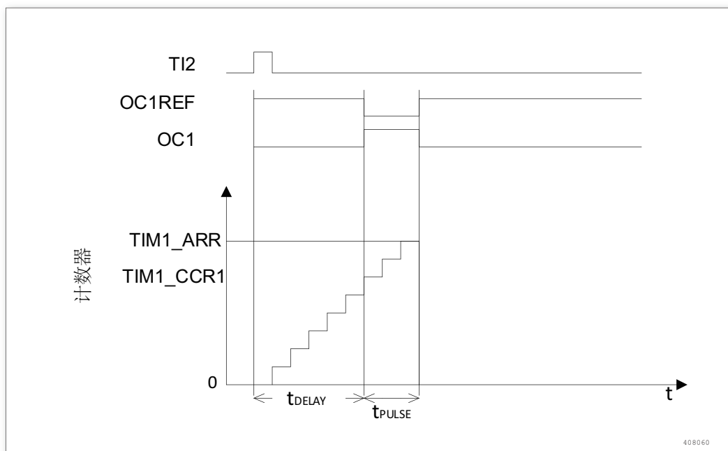
图 206. 单脉冲模式的例子
