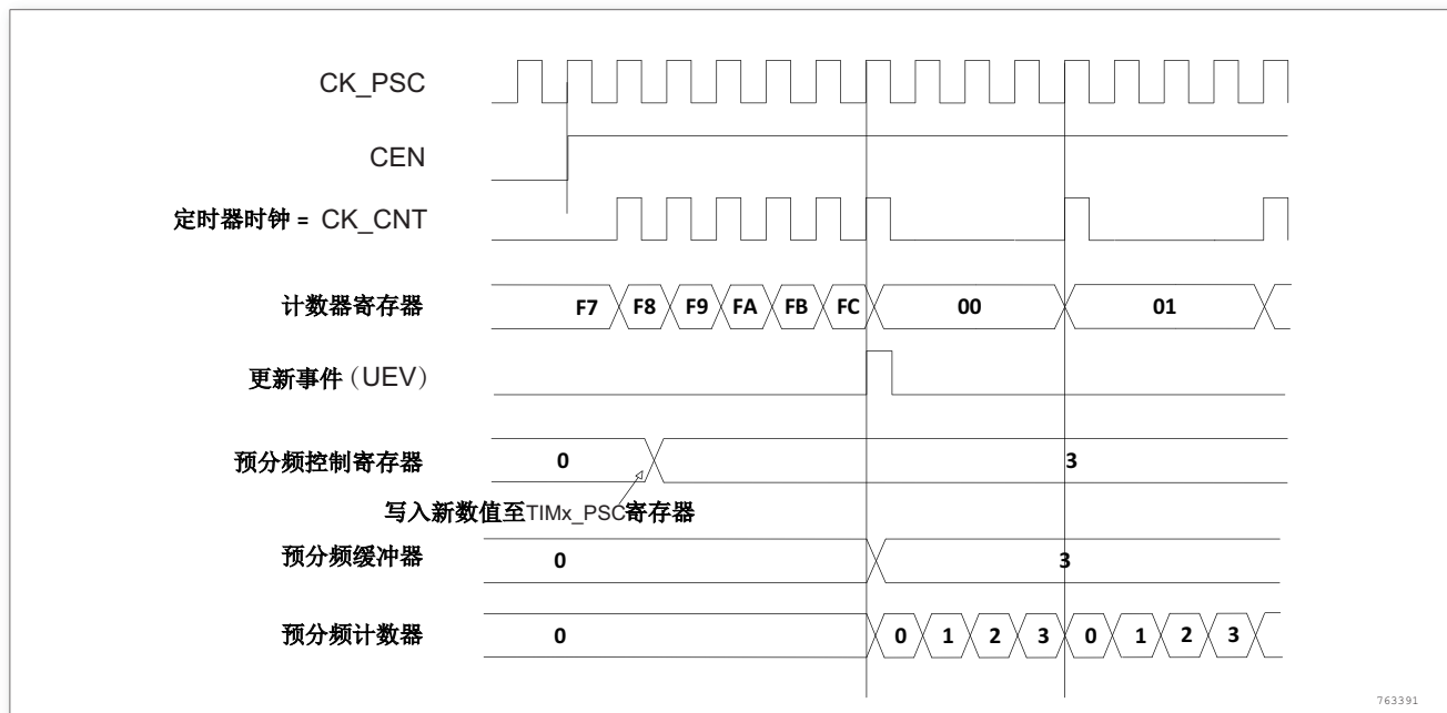
图 127. 当预分频器的参数从 1 变到 4 时，计数器的时序图
