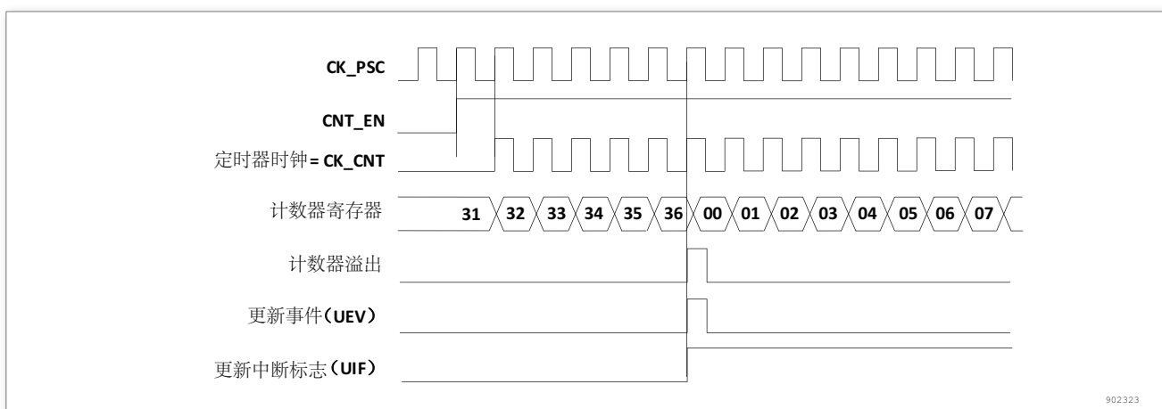
图 189. 计数器时序图，内部时钟分频因子为 1
