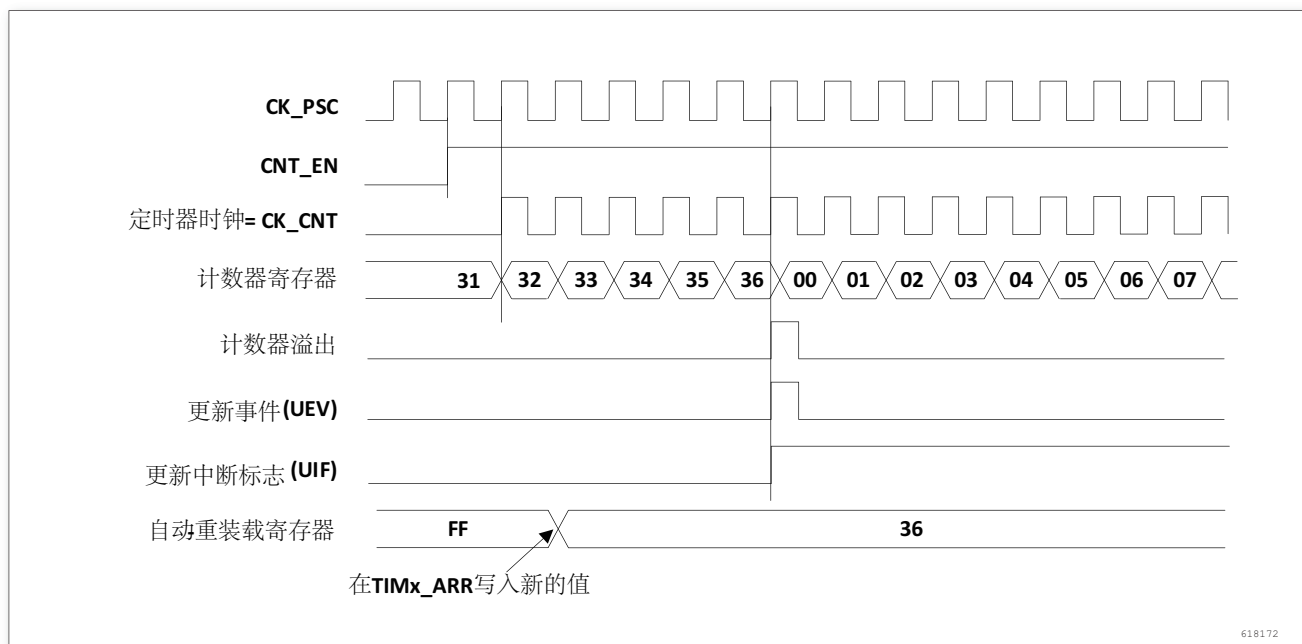
图 193. 计数器时序图, 当 ARPE = 0 时的更新事件 (TIMx_ARR 没有预装入)
