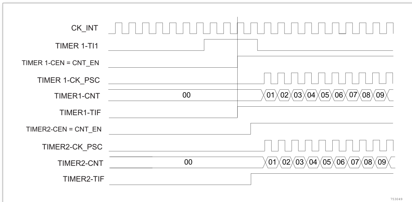
图 124. 使用定时器 1 的 TI1 输入触发定时器 1 和定时器 2
