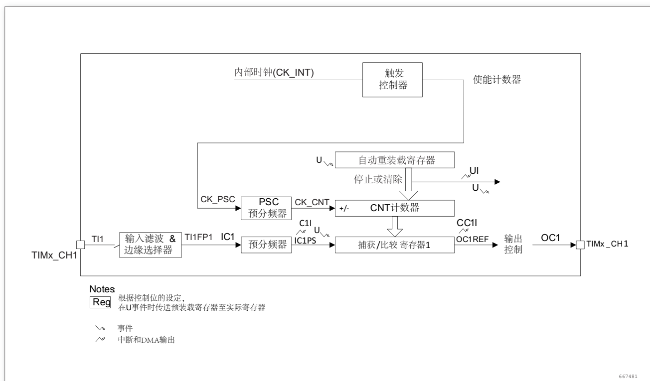
图 171. 基础定时器框图
