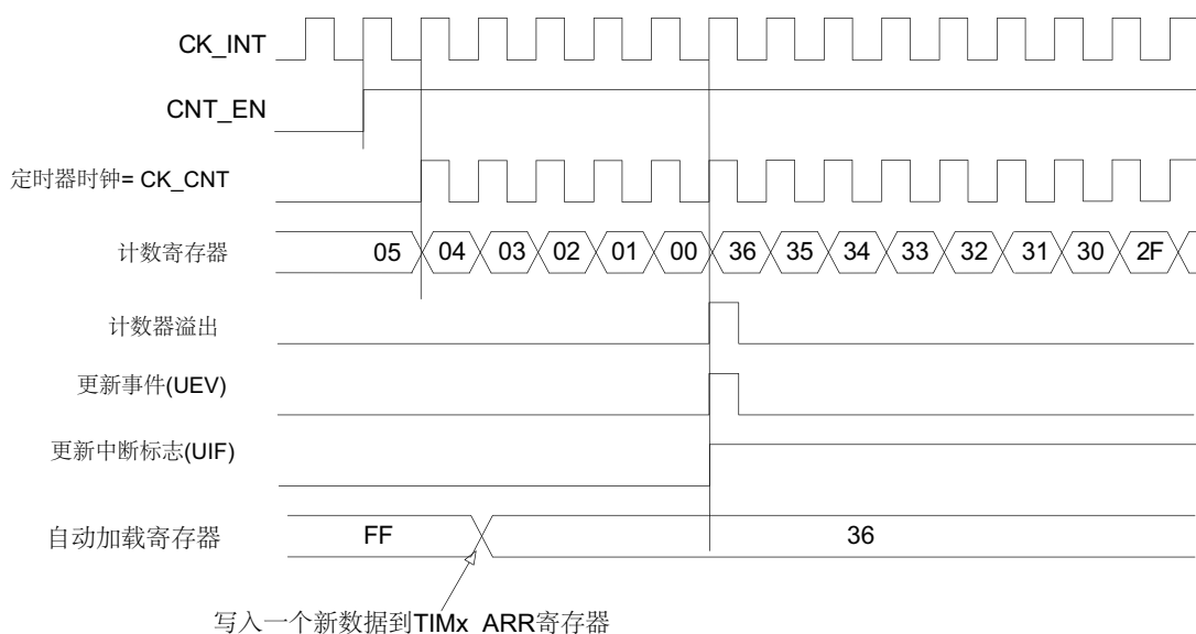
图 44. 计数器时序图，当没有使用重复计数器时的更新事件
