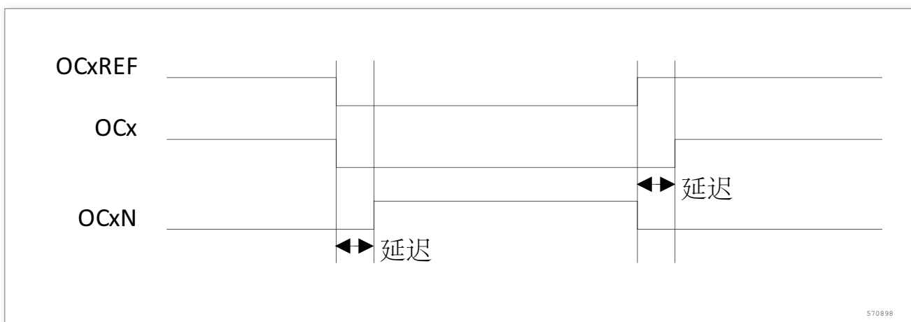
图 202. 带死区插入的互补输出
