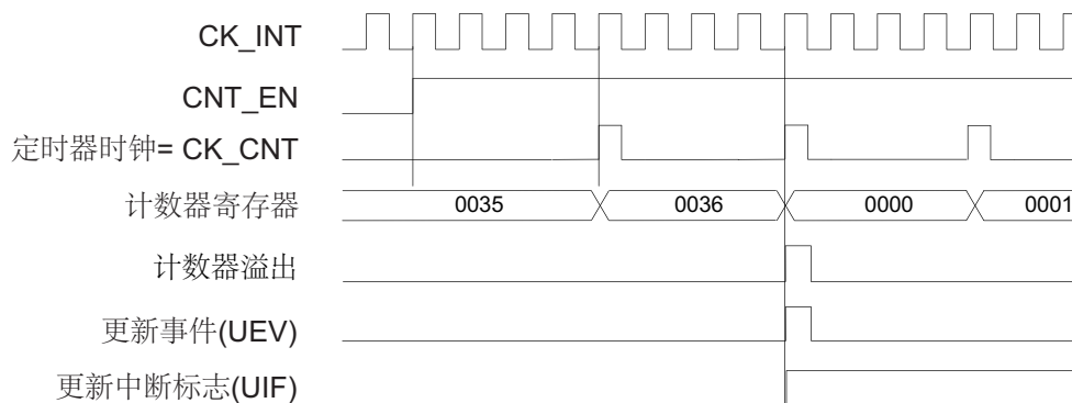
图 130. 计数器时序图，内部时钟分频因子为 4
