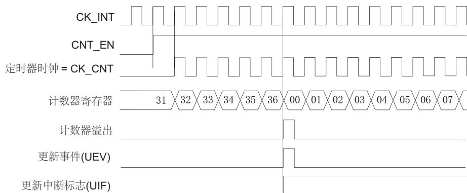
图 82. 计数器时序图，内部时钟分频因子为 1
