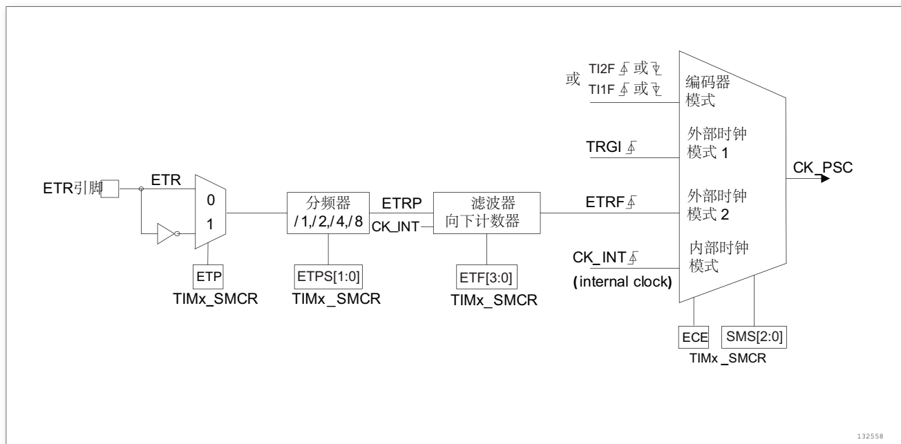
图 102. 外部触发输入框图
