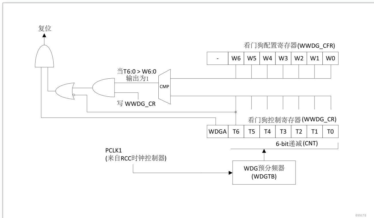
图 208. 看门狗框图
