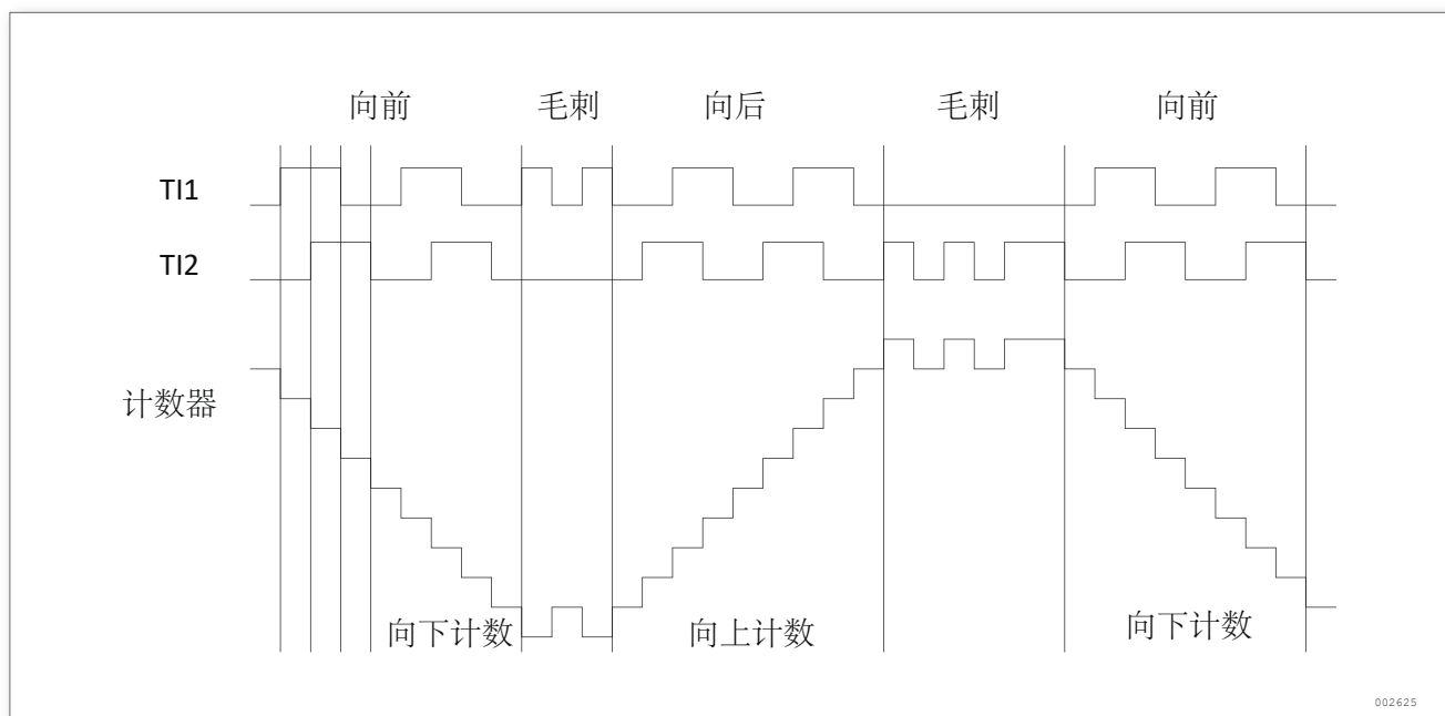
图 114. IC1FP1 反相的编码器接口模式实例
