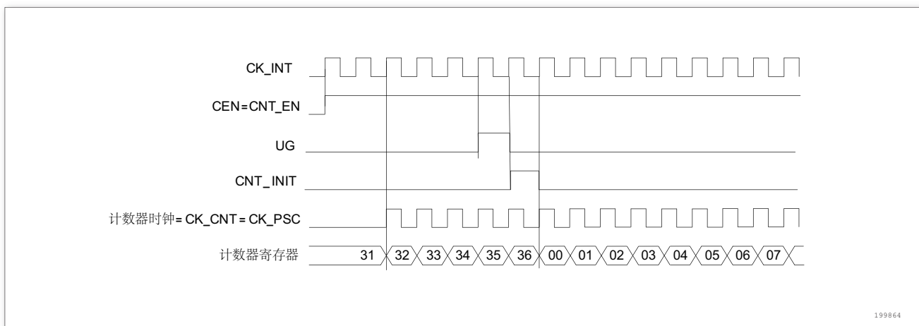
图 99. 一般模式下的控制电路, 内部时钟分频因子为 1
