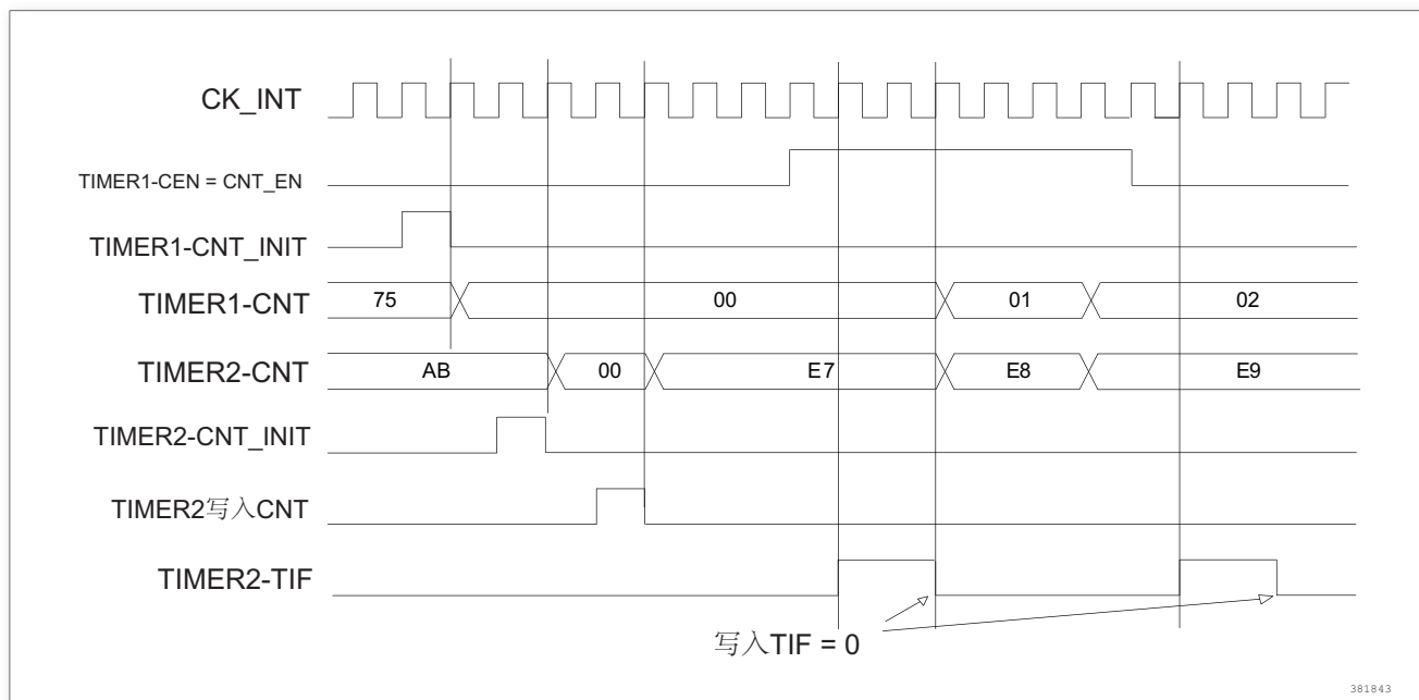
图 121. 通过使能定时器 1 可以控制定时器 2
