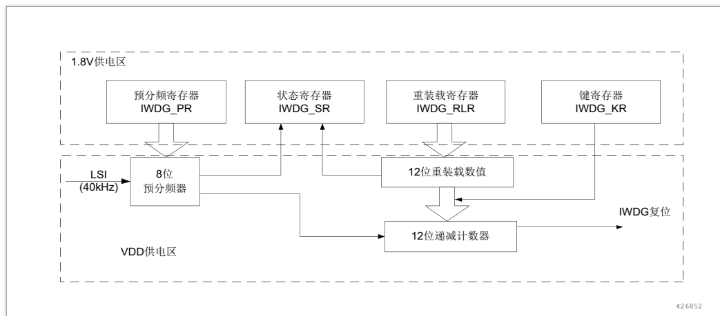
图 207. 独立看门狗框图
