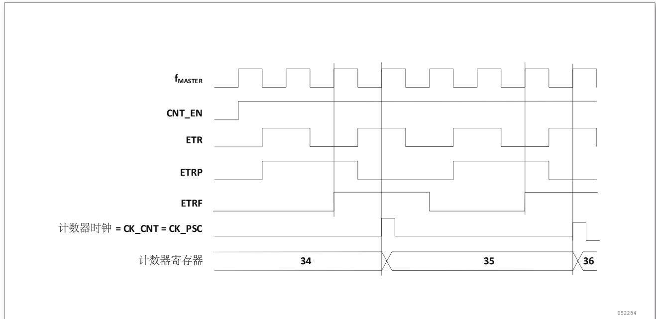
图 103. 外部时钟模式 2 下的控制电路
