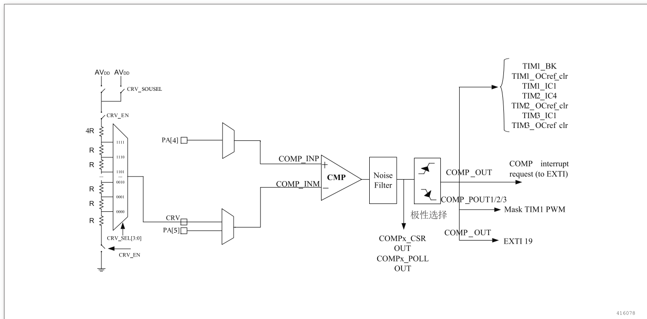
图 29. 比较器框图
