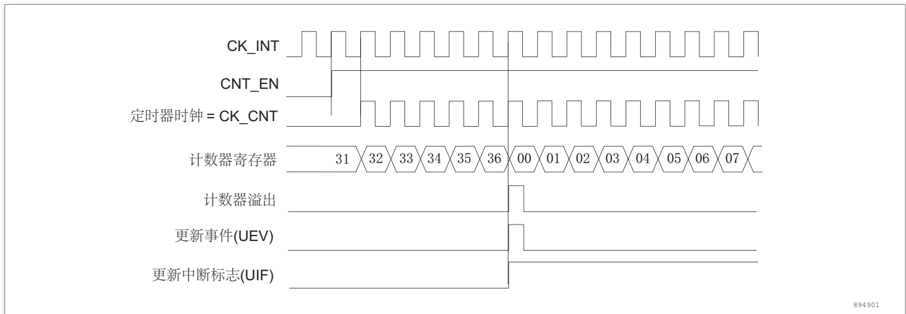
图 174. 计数器时序图，内部时钟分频因子为 1
