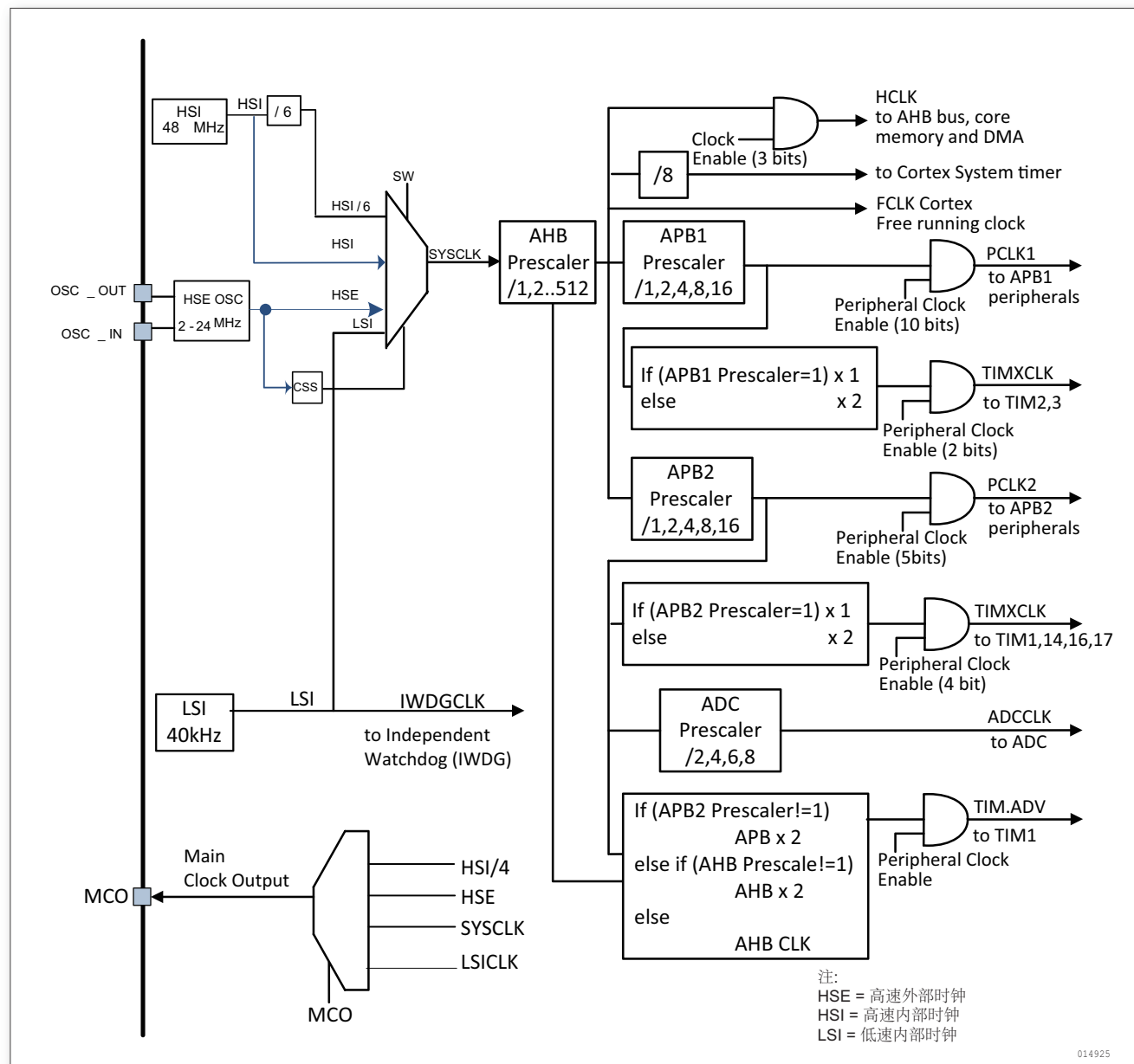
图 12. 时钟树
