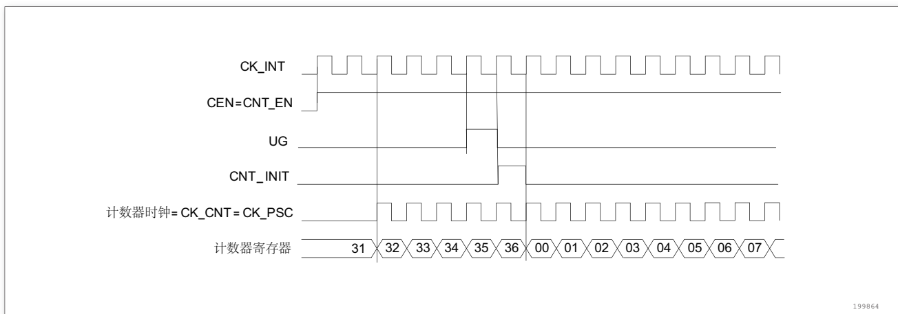
图 180. 一般模式下的控制电路，内部时钟分频因子为 1
