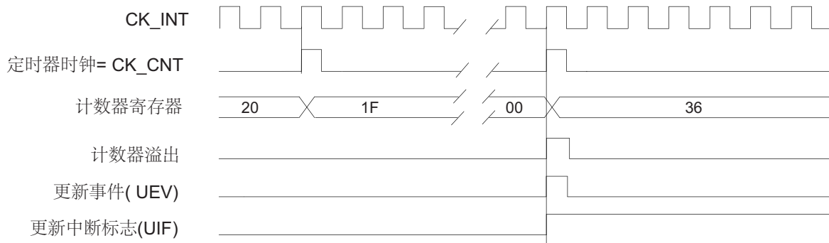
图 91. 计数器时序图，内部时钟分频因子为 N
