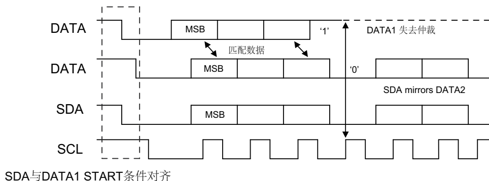
图 222. 多个主机仲裁
