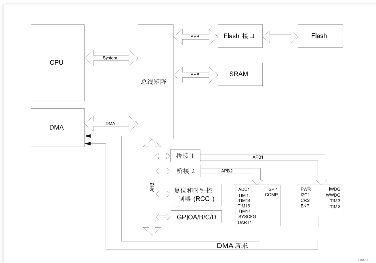
图 1. 系统架构
