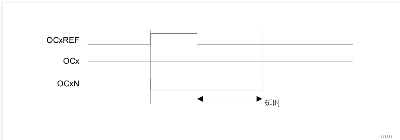
图 67. 死区波形延迟大于正脉冲
