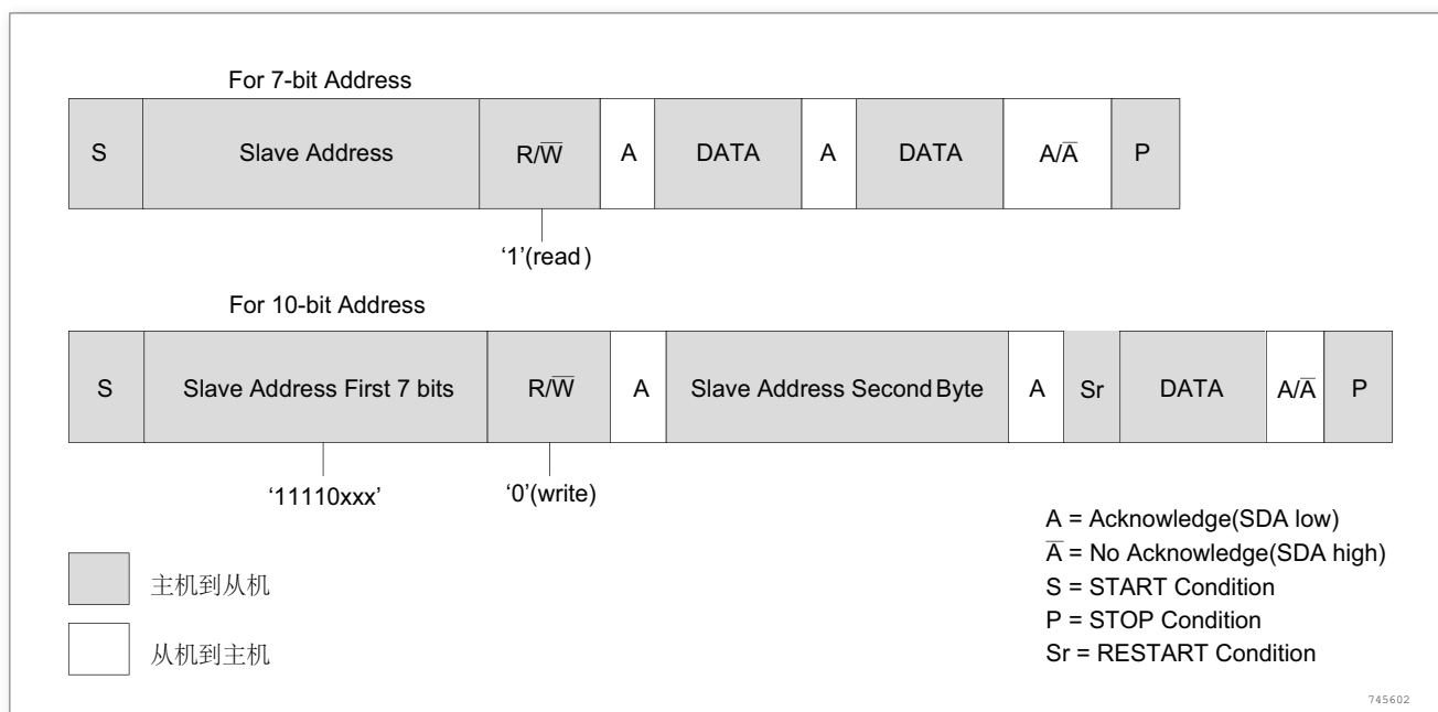
图 217. 主接收协议
