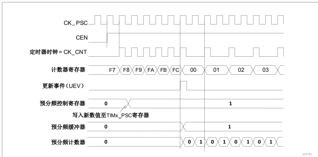
图 80. 当预分频器的参数从 1 变到 2 时, 计数器的时序图
