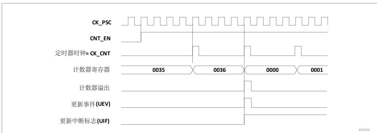
图 191. 计数器时序图, 内部时钟分频因子为 4
