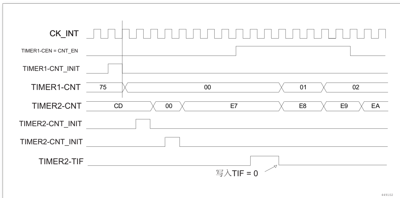
图 123. 利用定时器 1 的使能触发定时器 2
