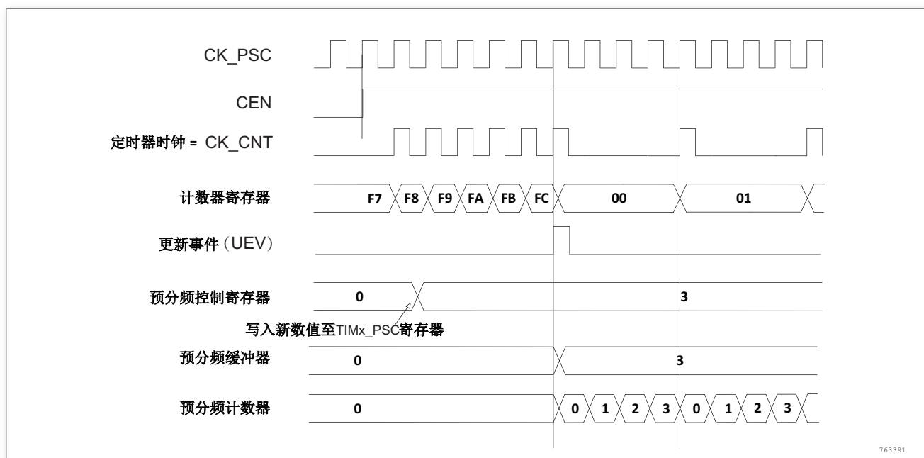
图 81. 当预分频器的参数从 1 变到 4 时，计数器的时序图
