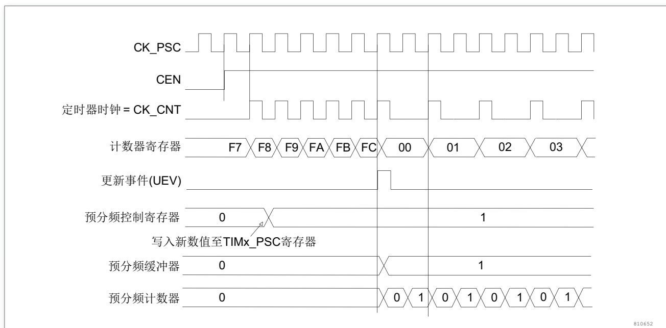
图 32. 当预分频器的参数从 1 变到 2 时，计数器的时序图
