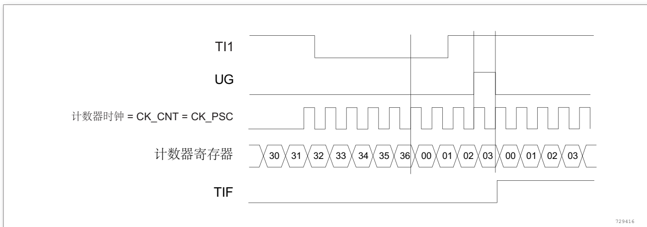
图 115. 复位模式下的控制电路
