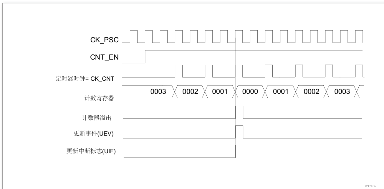
图 46. 计数器时序图，内部时钟分频因子为 2
