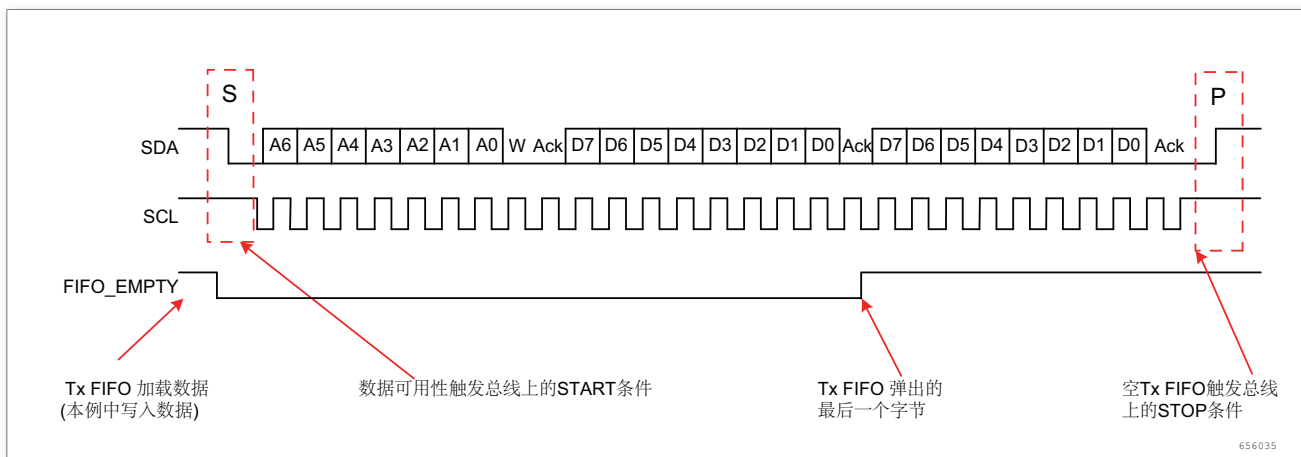
图 220. 主发送 - Tx FIFO 为空
