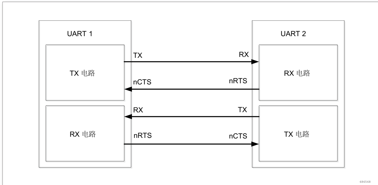
图 233. 两个 UART 间的硬件流控制
