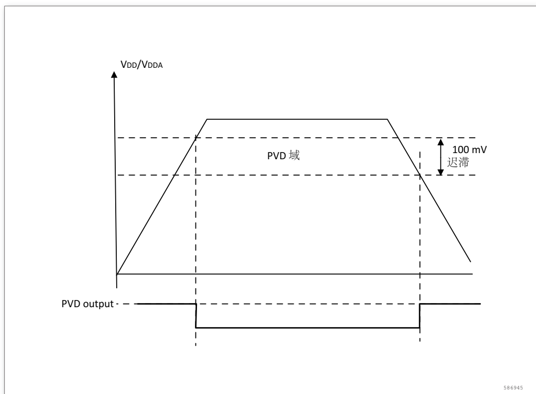
图 9. PVD 的阈值
