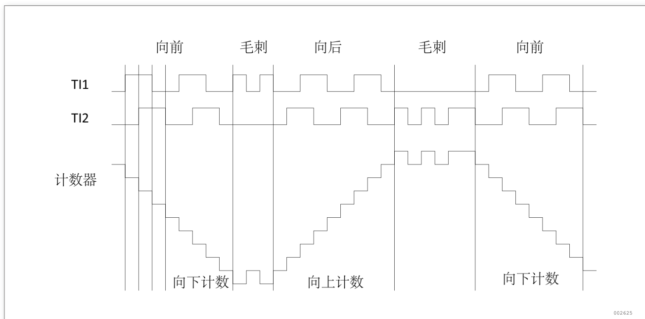
图 160. IC1FP1 反相的编码器接口模式实例
