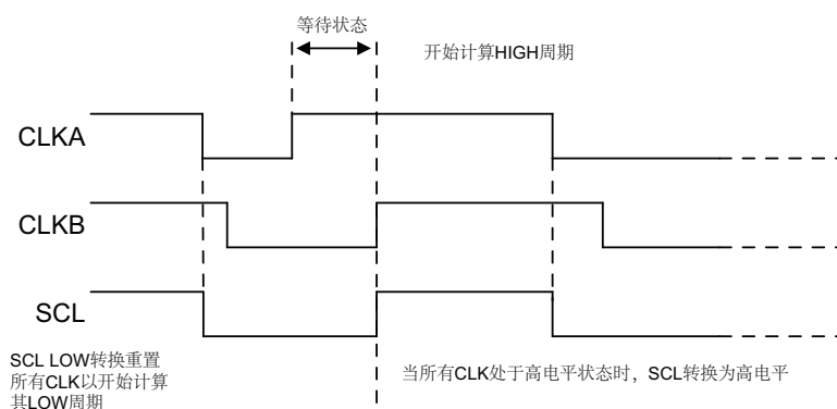
图 223. 多个主机时钟同步
