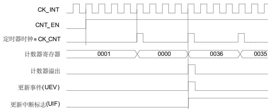
图 90. 计数器时序图，内部时钟分频因子为 4
