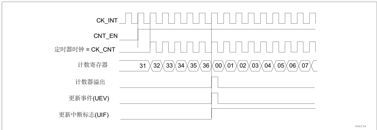
图 34. 计数器时序图，内部时钟分频因子为 1
