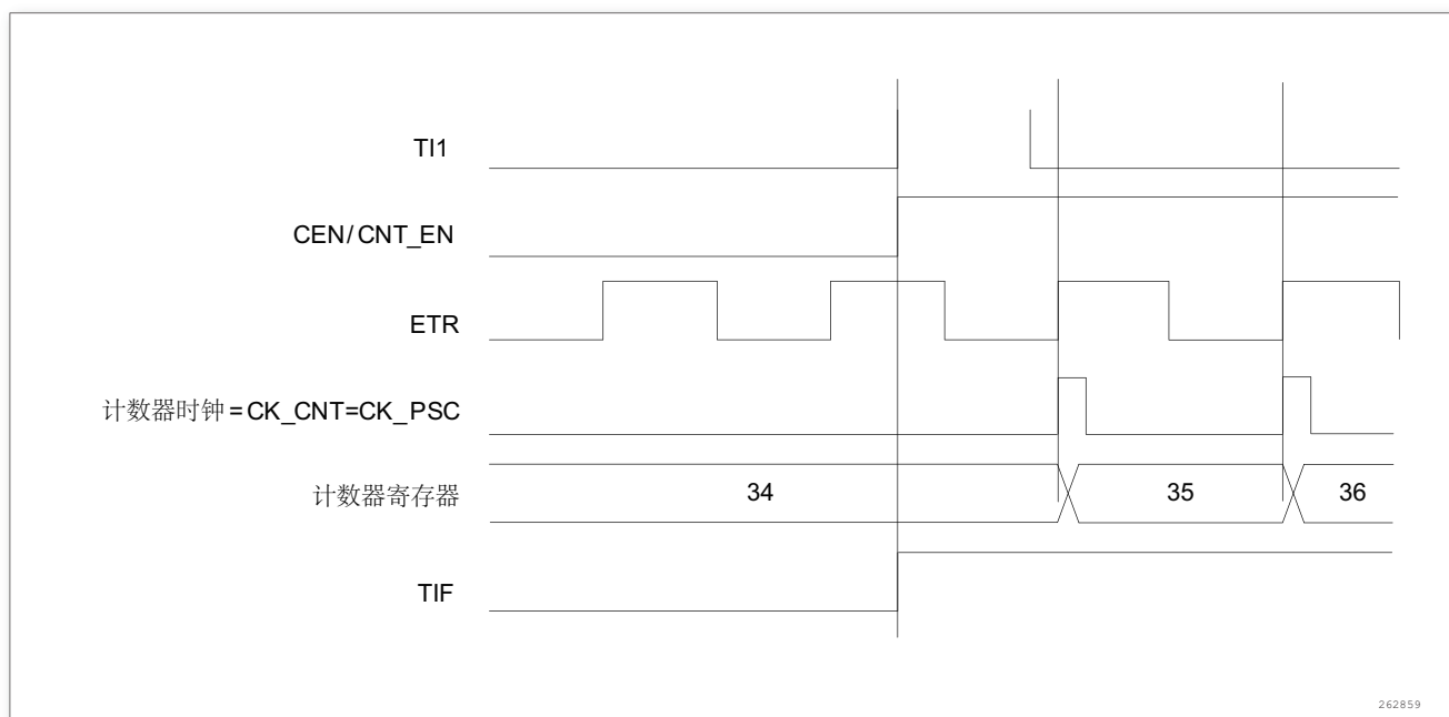
图 118. 外部时钟模式 2 + 触发模式下的控制电路
