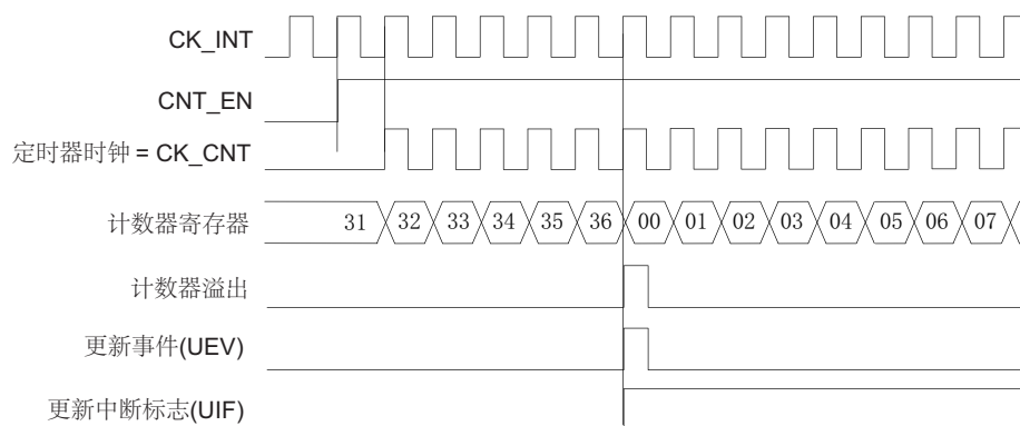
图 128. 计数器时序图，内部时钟分频因子为 1
