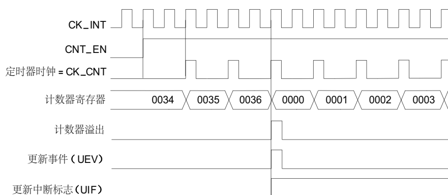
图 129. 计数器时序图，内部时钟分频因子为 2
