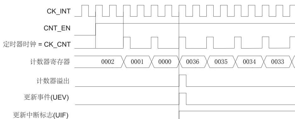
图 89. 计数器时序图，内部时钟分频因子为 2
