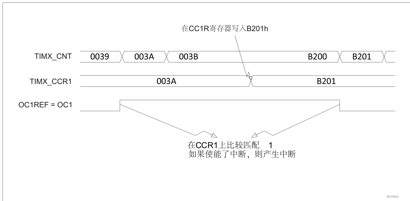
图 154. 输出比较模式，翻转 OC1
