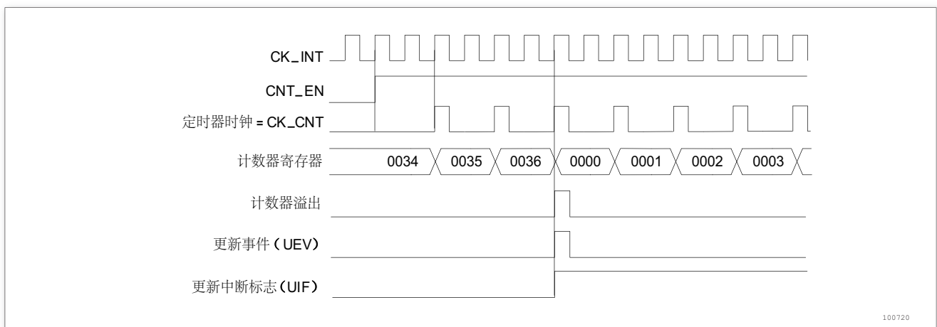
图 175. 计数器时序图，内部时钟分频因子为 2
