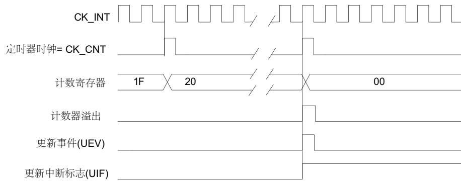
图 37. 计数器时序图，内部时钟分频因子为 N
