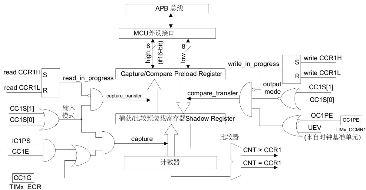
图 58. 捕获/比较通道 1 的主电路
