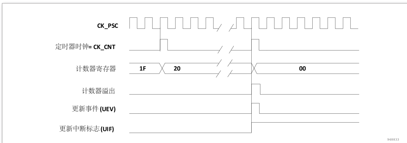
图 192. 计数器时序图, 内部时钟分频因子为 N
