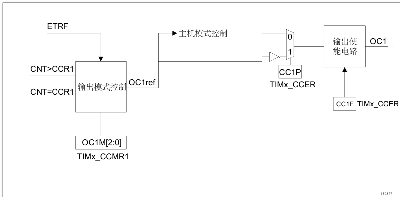
图 59. 捕获/比较通道的输出部分 (通道 1 至 3)
