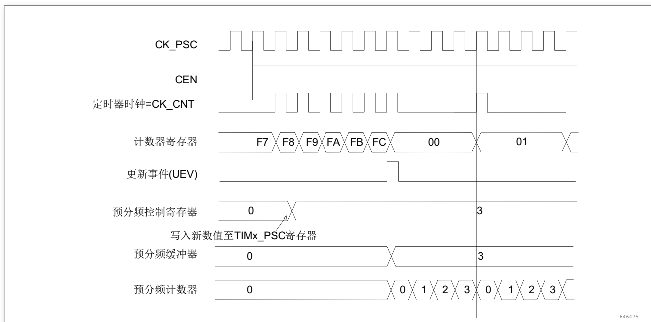
图 33. 当预分频器的参数从 1 变到 4 时, 计数器的时序图
