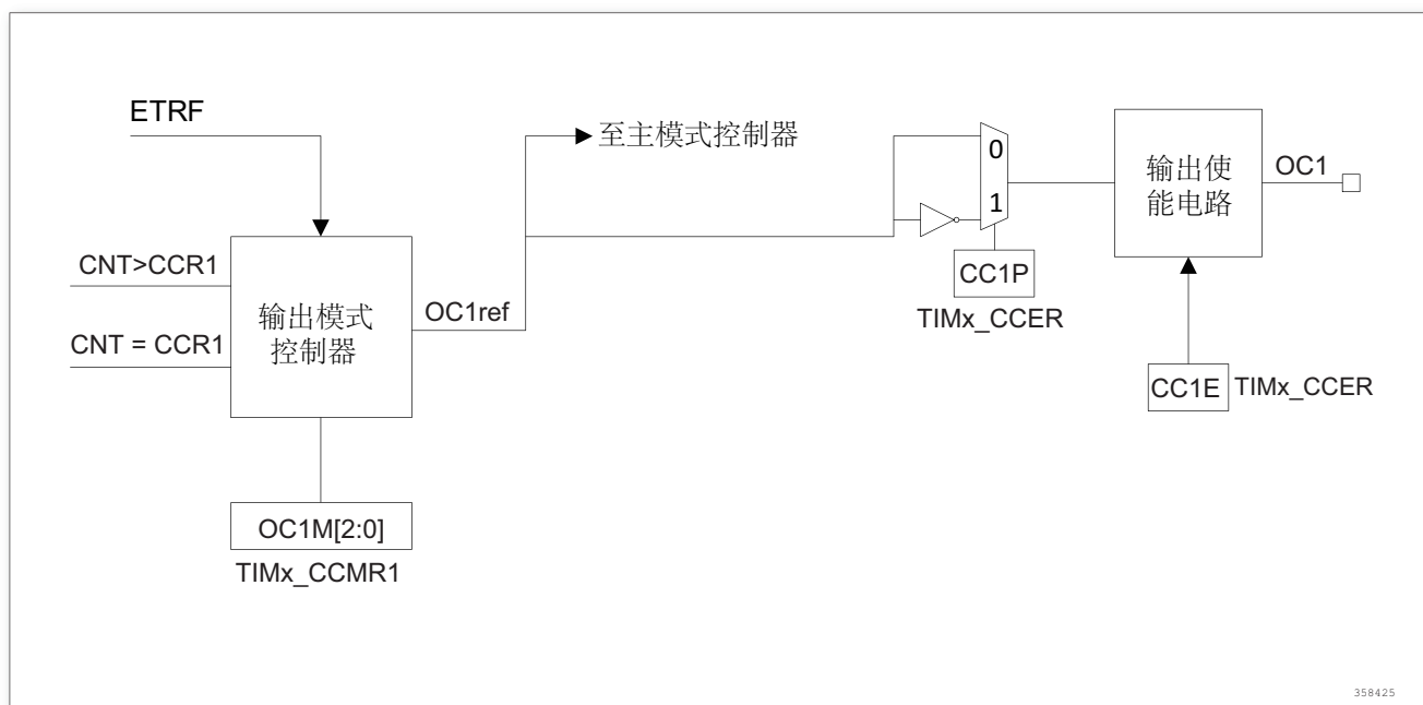
图 152. 捕获/比较通道的输出部分 (通道 1)
