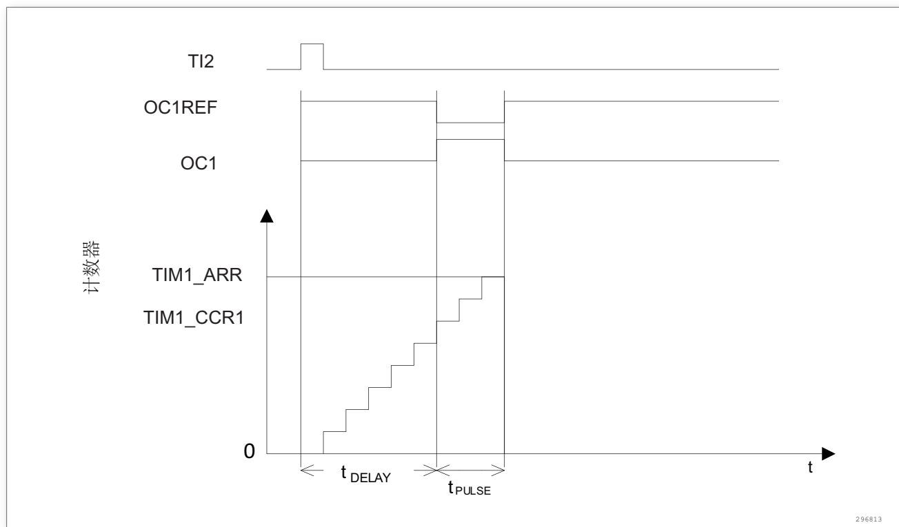
图 111. 单脉冲模式的例子
