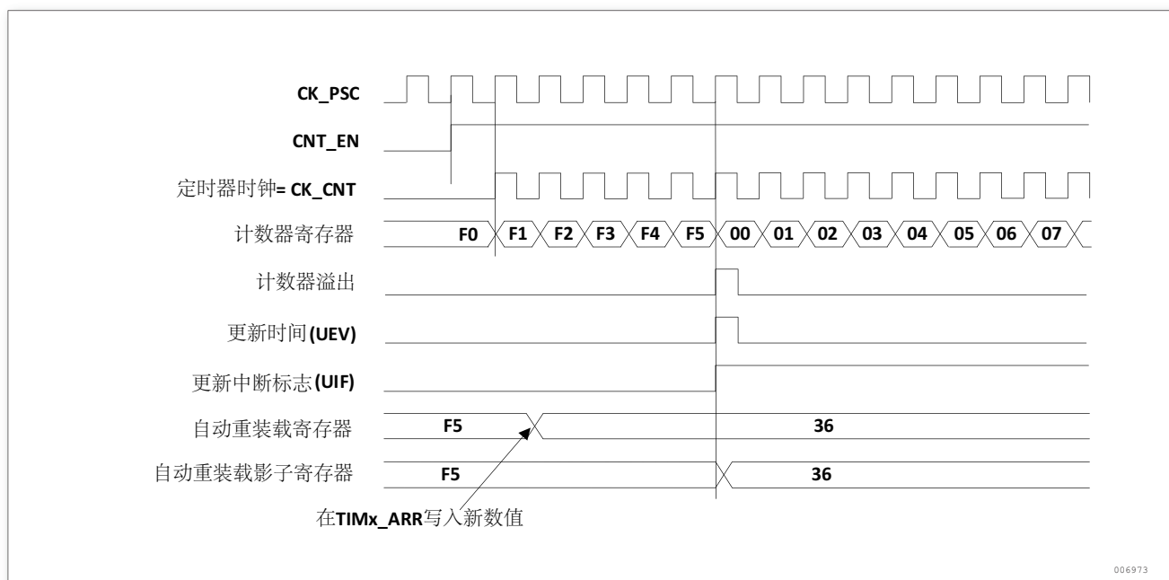
图 194. 计数器时序图，当 ARPE = 1 时的更新事件 (TIMx_ARR 预装载)
