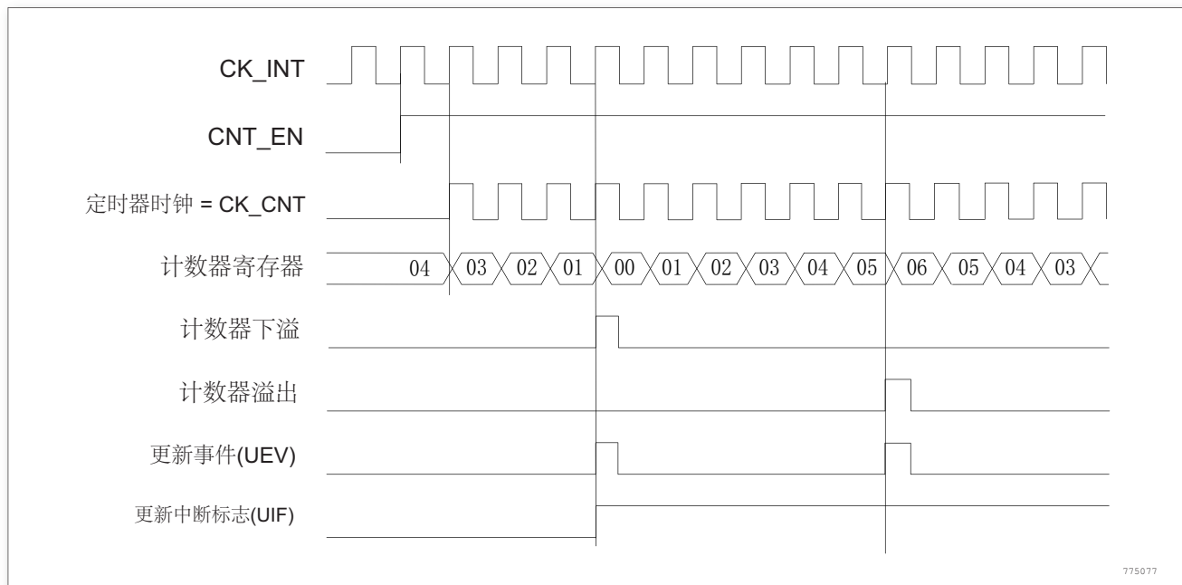
图 139. 计数器时序图，内部时钟分频因子为 1，TIMx_ARR = 0x6
