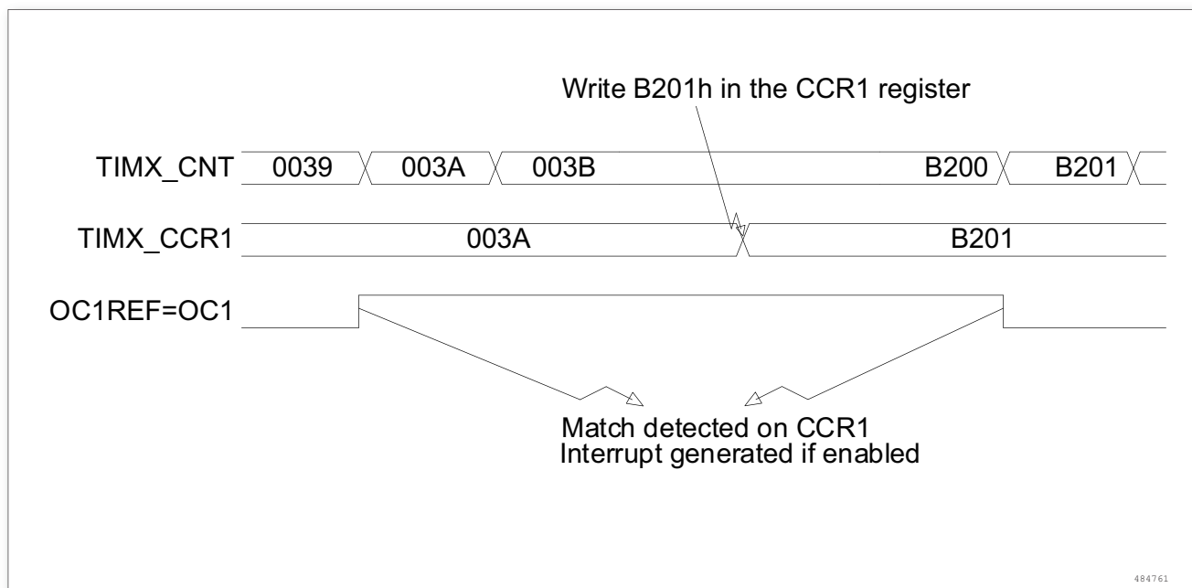
图 62. 输出比较模式，翻转 OC1
