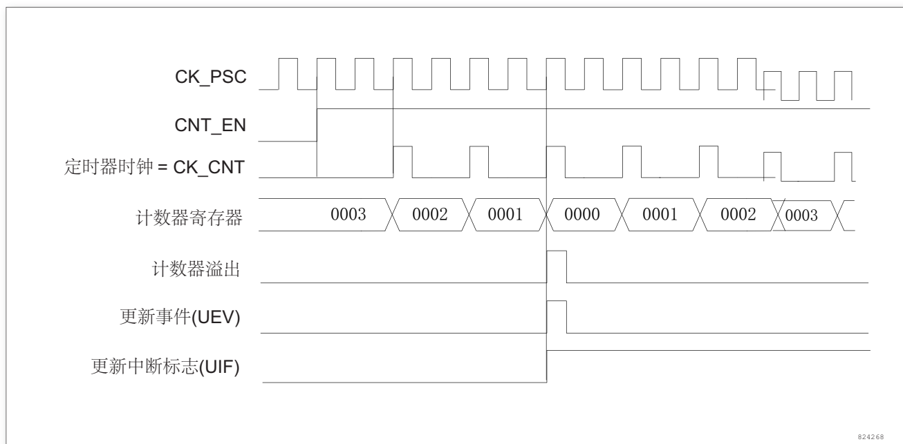
图 140. 计数器时序图，内部时钟分频因子为 2
