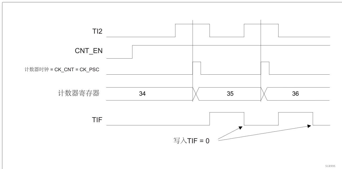
图 147. 外部时钟模式 1 下的控制电路
