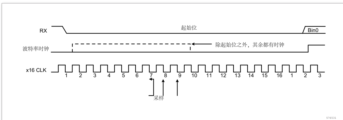
图 232. RX 引脚采样方案
