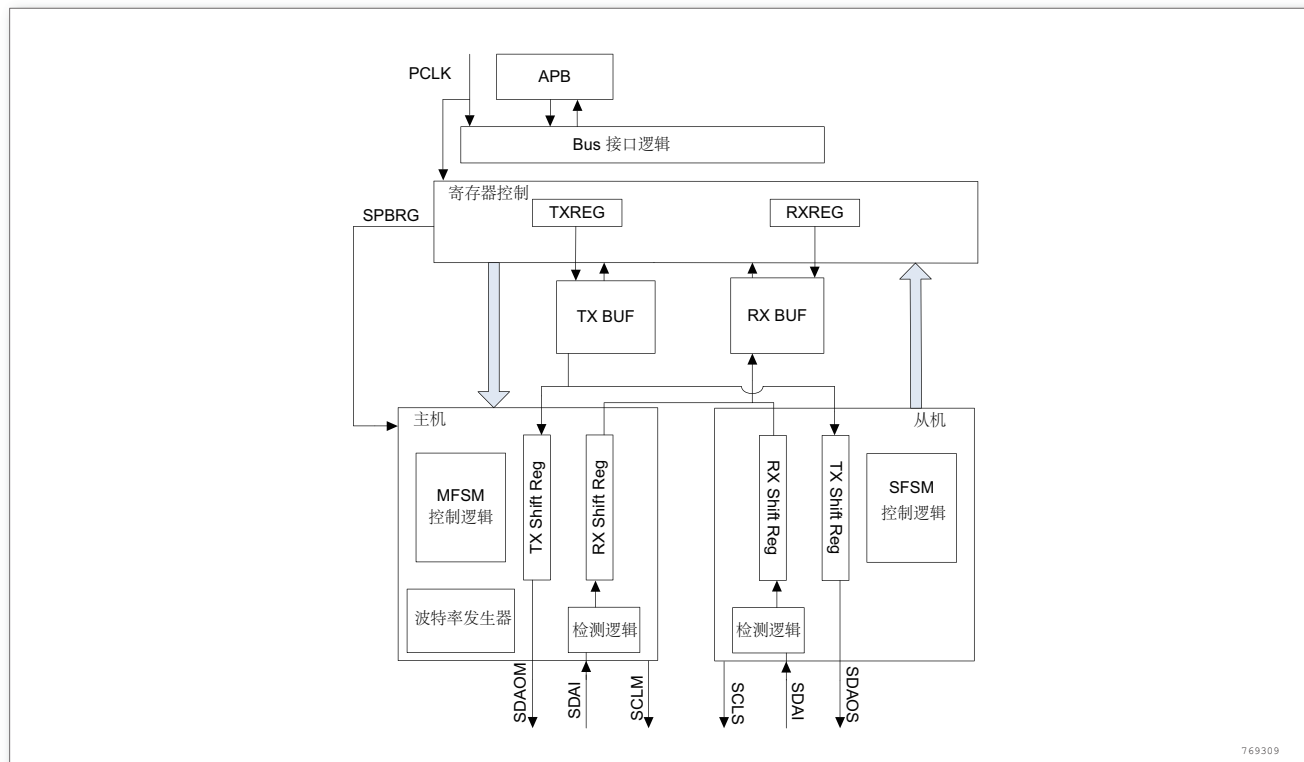
图 224. I 2 C 功能框图
