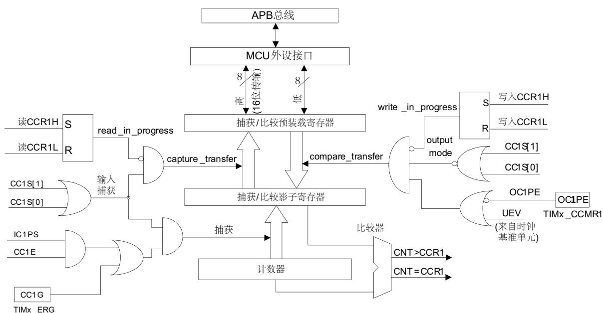
图 105. 捕获/比较通道 1 的主电路
