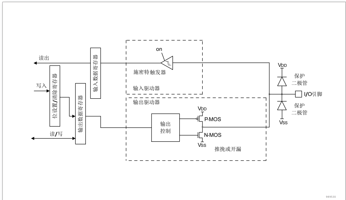
图 17. 输出配置
