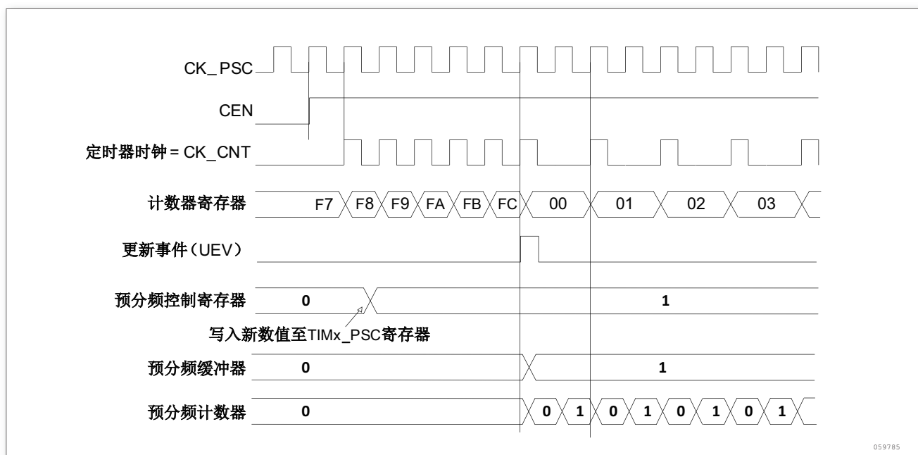
图 126. 当预分频器的参数从 1 变到 2 时, 计数器的时序图
