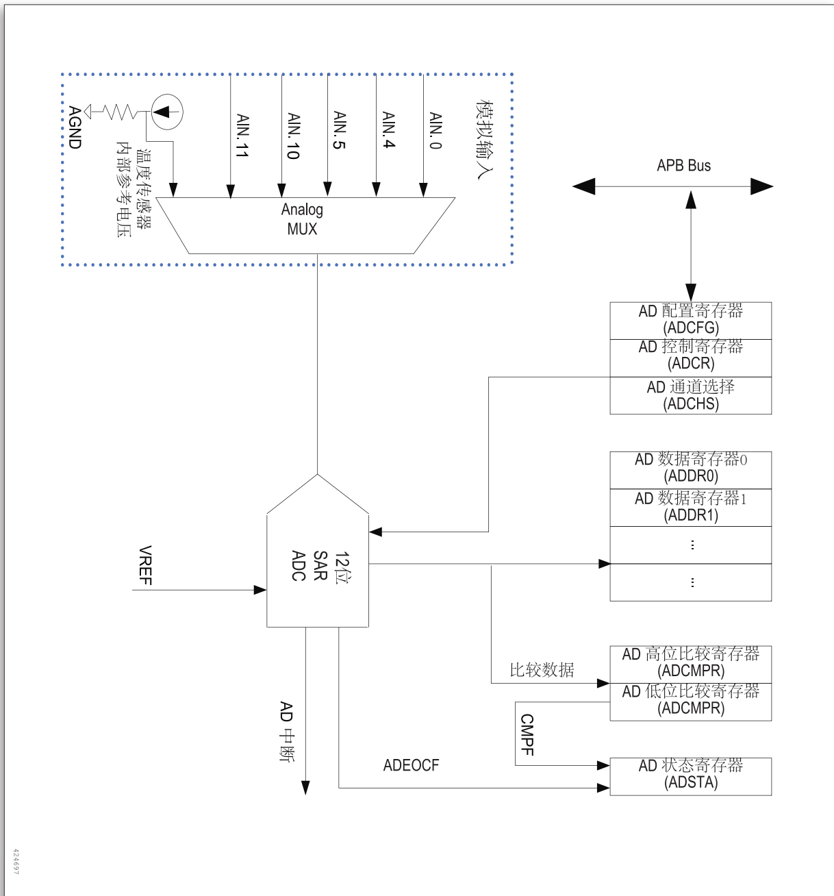
图 24. ADC 框图
