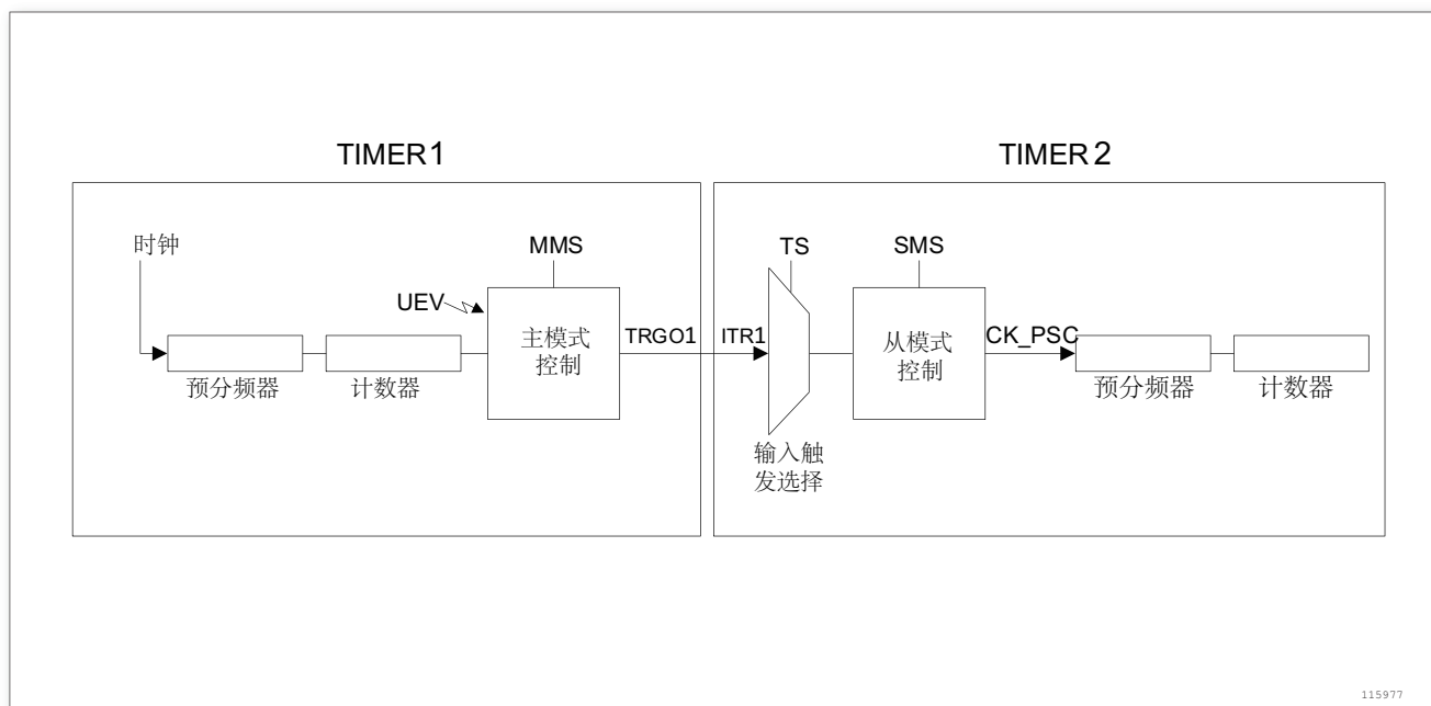
图 165. 主/从定时器的例子
