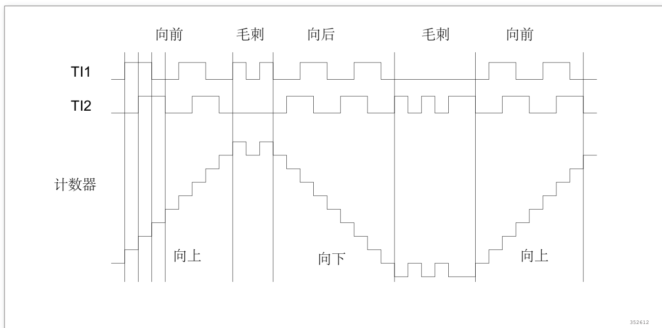
图 72. 编码器模式下的计数器操作实例
