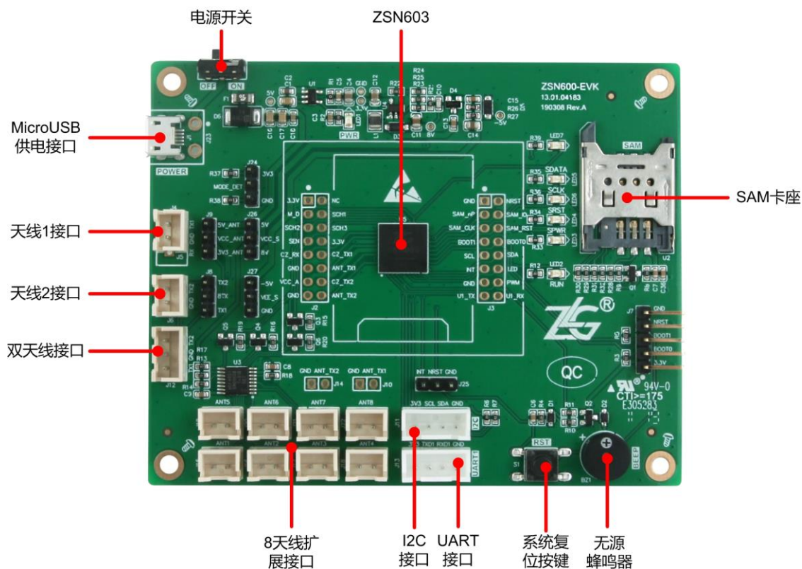
图 1.3 ZSN603-EVK 开发板资源分布
