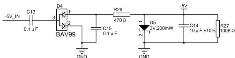
图 1.6 负压电路
