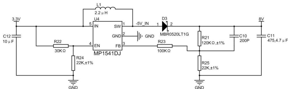
图 1.5 升压电路
