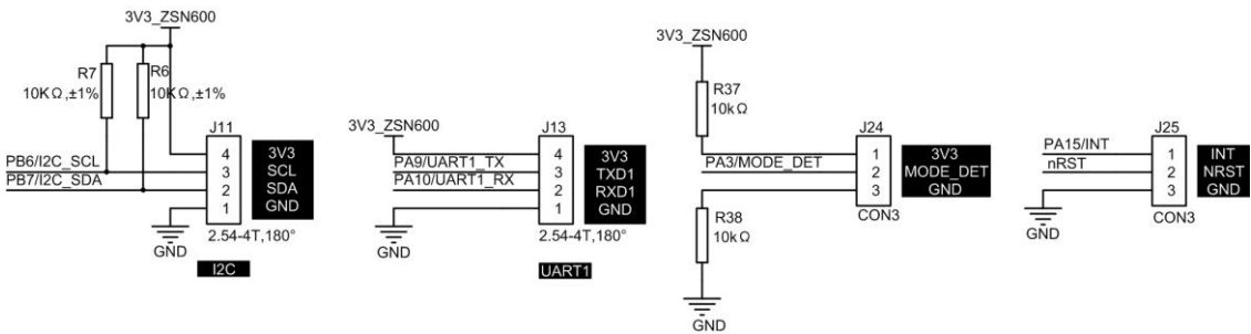
图 1.13 通信接口
