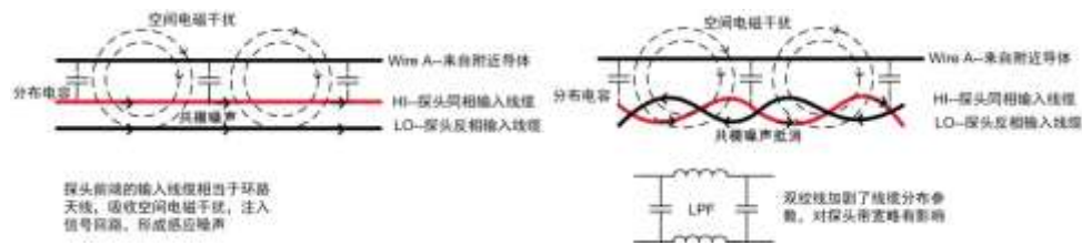
图 4.5 输入线缆双绞利与弊
