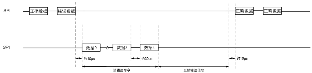
图 3.19 SPI 错误反馈机制时序图
