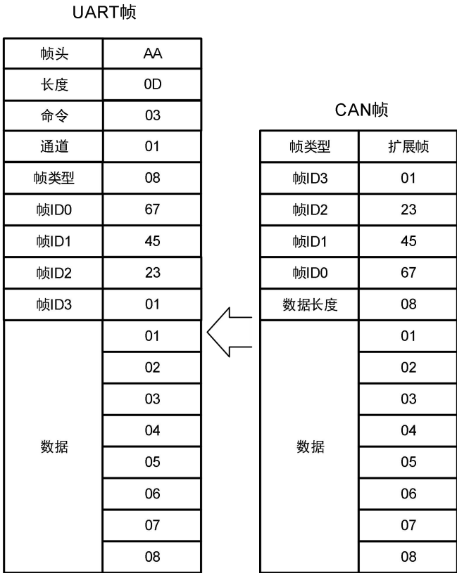
图 3.8 CAN 帧转 UART 帧示例（自定义协议转换）
