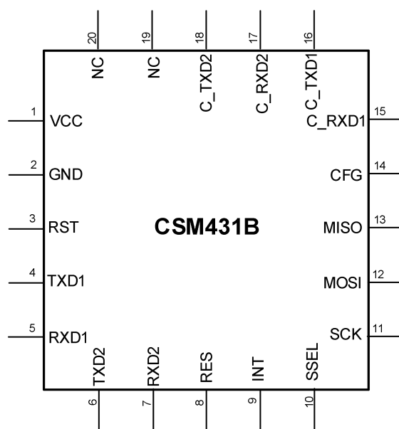
图 2.2 CSM431B 引脚排列
