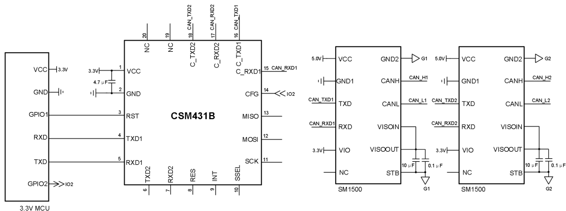
图 2.6 UART1 转 CANFD1 和 CANFD2 硬件电路
