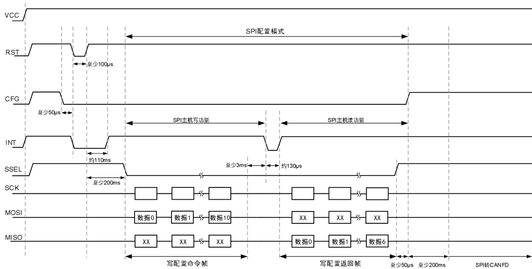
图 4.1 通过 SPI 写配置命令的时序图
