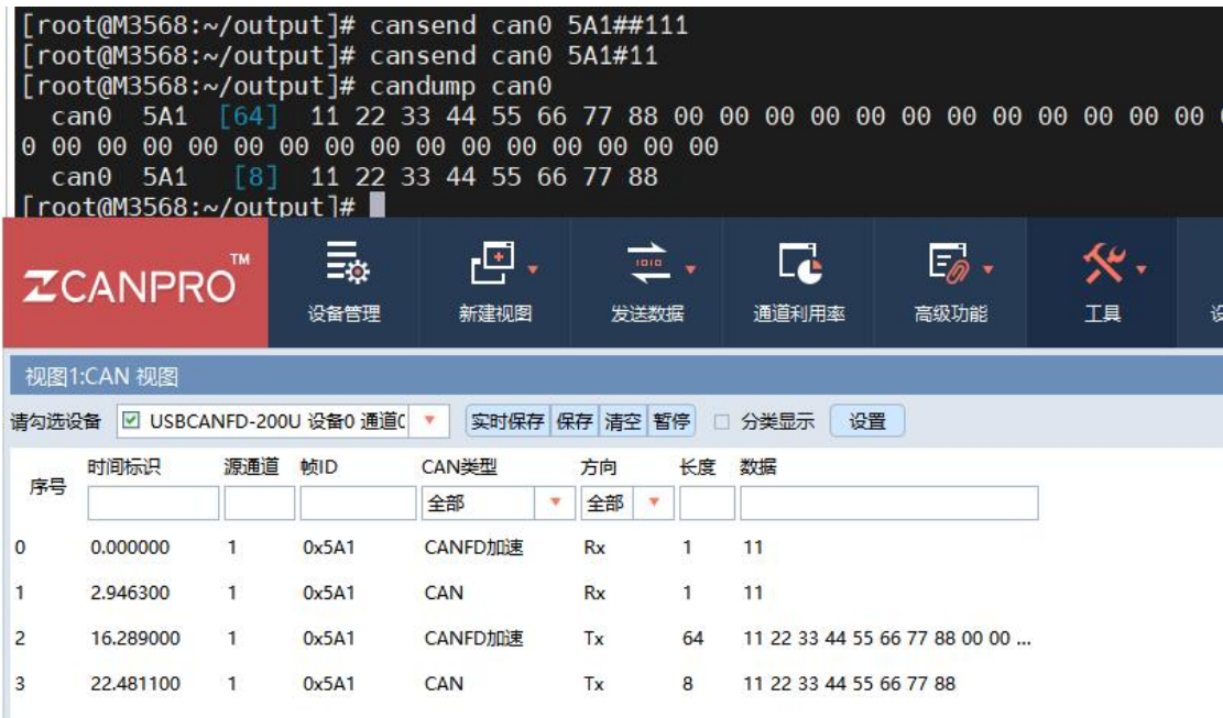
图 6.3 使用 UART1 和 UART2 转 CANFD1 和 CANFD2 驱动 在 UART1 转 CANFD1 数据流通道进行数据收发
