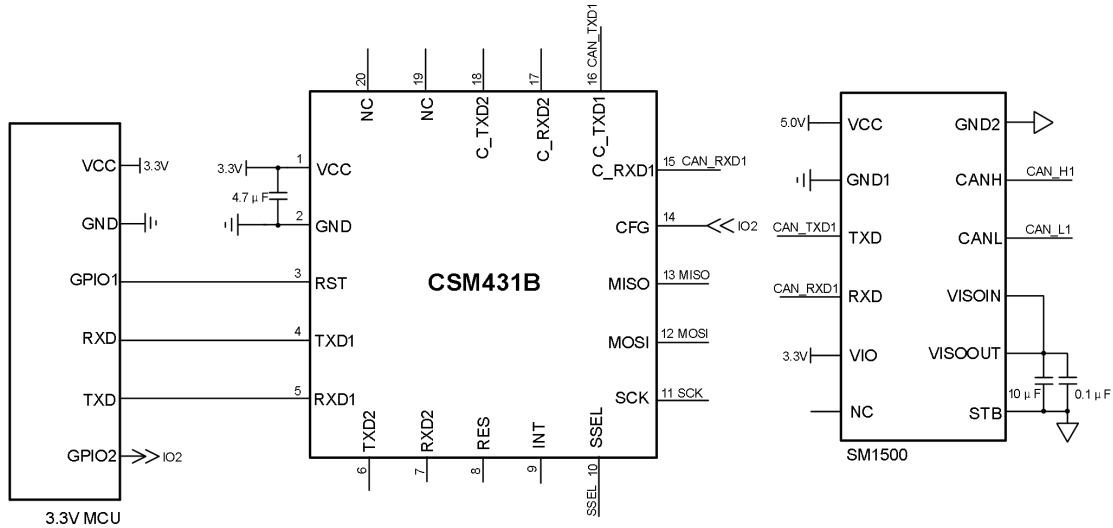
图 2.5 UART1 转 CANFD1 参考电路
