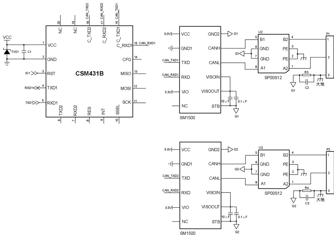
图 2.8 外围保护电路 1
