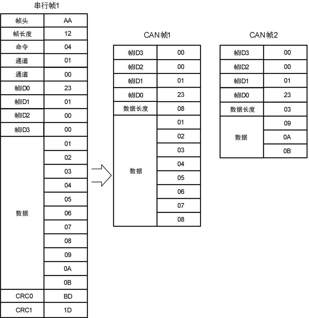
图 3.13 串行帧转 CAN/CANFD 帧示例（自定义带校验协议转换）
