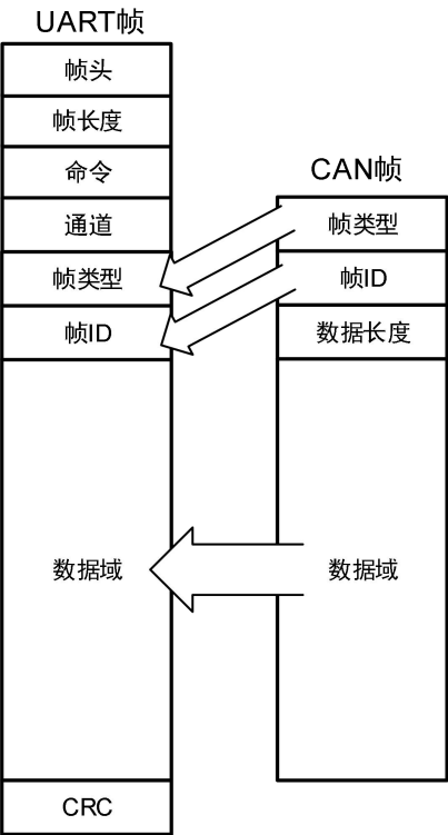
图 3.14 CAN/CANFD 帧转 UART 帧（自定义带校验协议转换）
