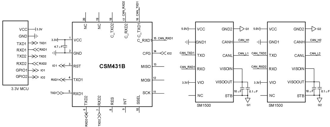
图 2.7 UART1 和 UART2 转 CANFD1 和 CANFD2 参考电路
