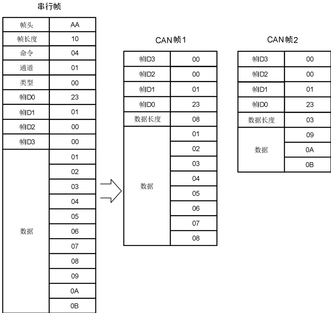
图 3.6 串行帧转 CAN/CANFD 帧示例（自定义协议转换）
