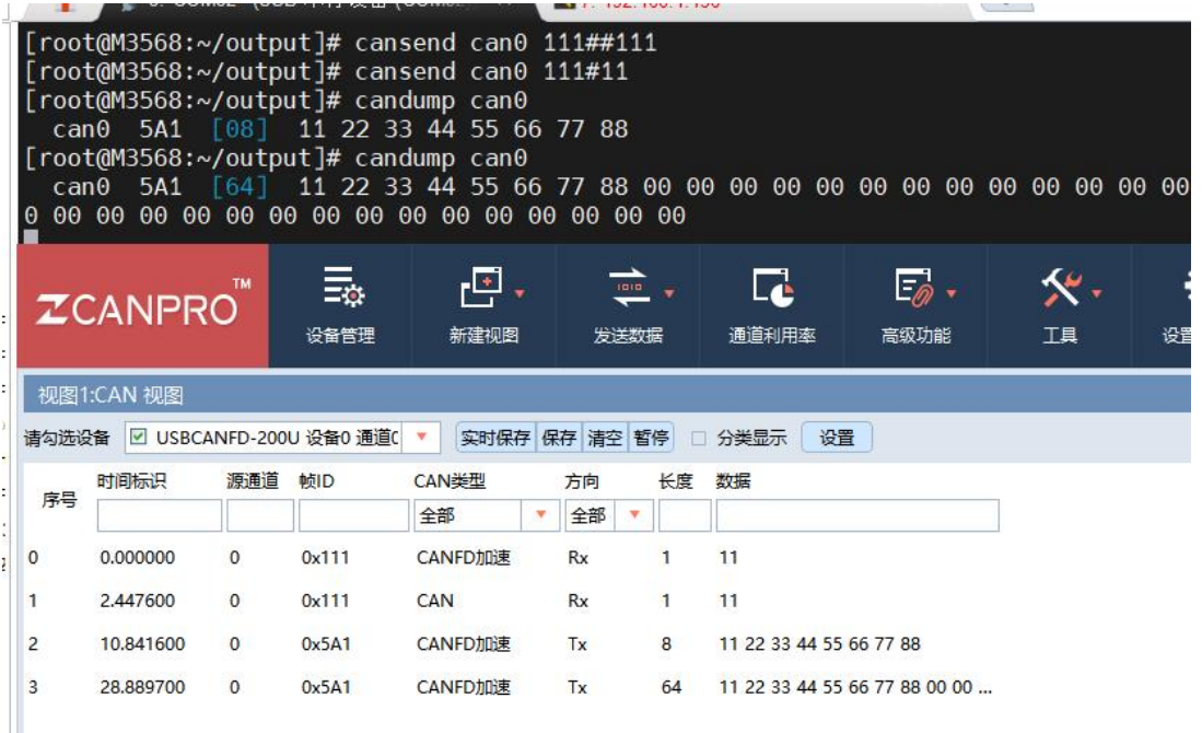
图 6.1 使用 UART1 转 CANFD1 和 CANFD2 驱动 在 UART1 转 CANFD1 数据流通道进行数据收发
