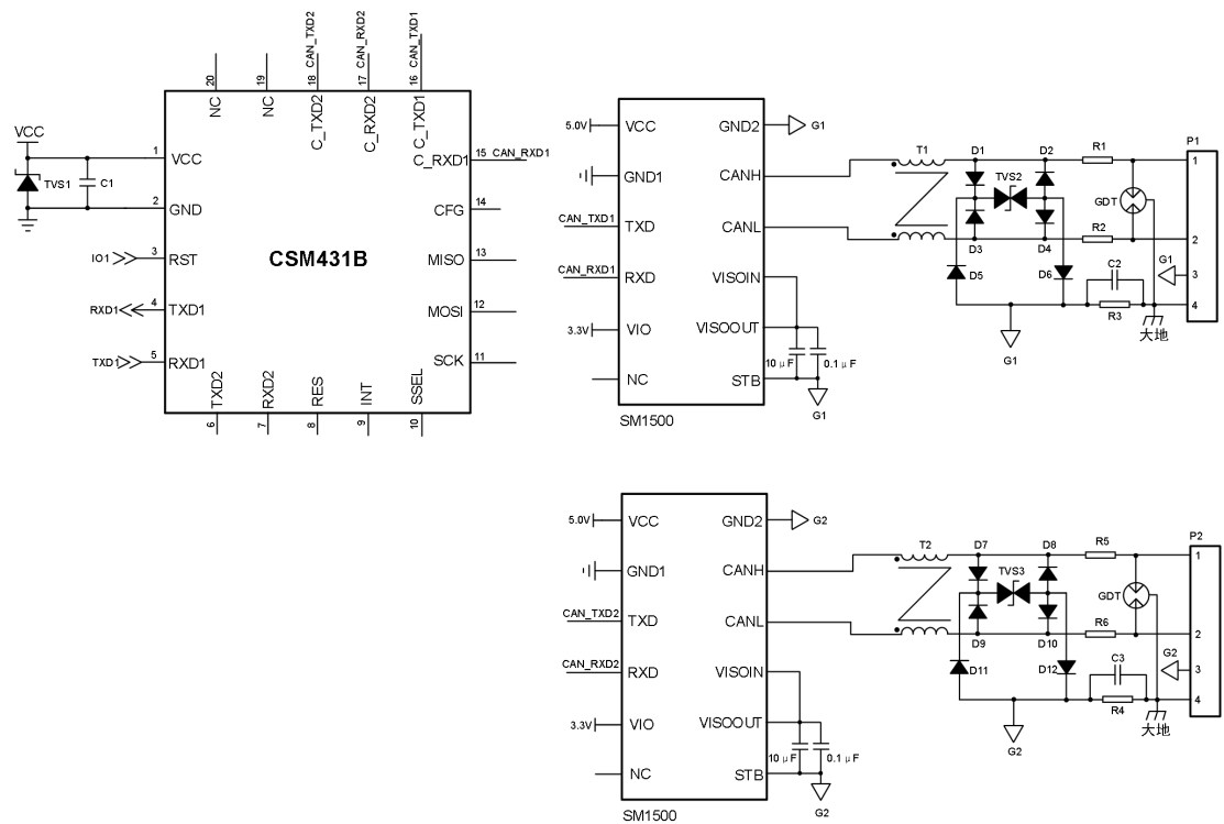
图 2.9 外围保护电路 2
