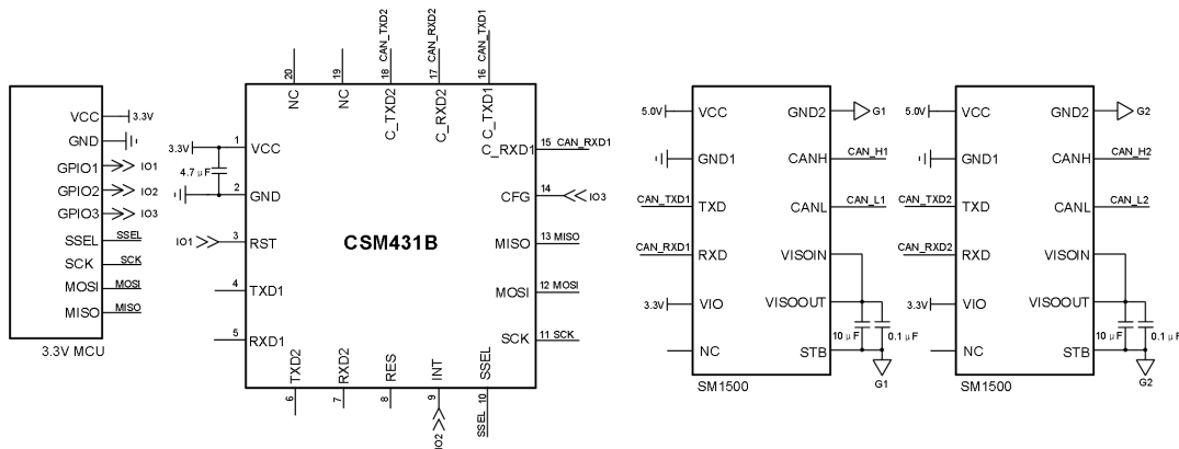
图 2.4 SPI 转 CANFD1 和 CANFD2 参考电路
