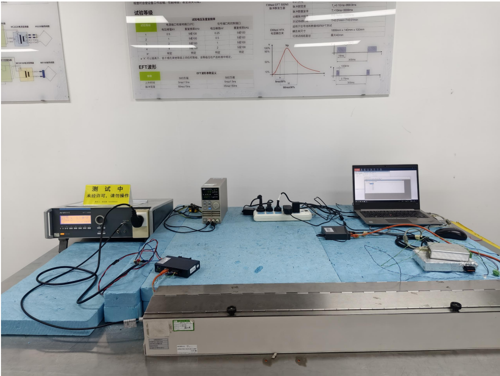
图 6 电快速瞬变脉冲群抗扰度试验现场配置图
