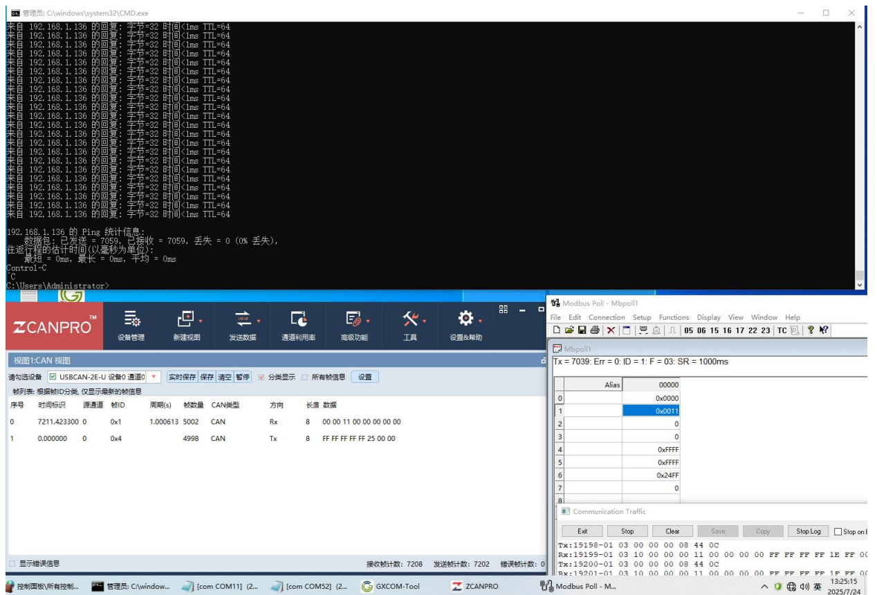
图 11 样机在低温试验第一次启动检查功能正常 (RTU 模式, 供电电压 9VDC)
