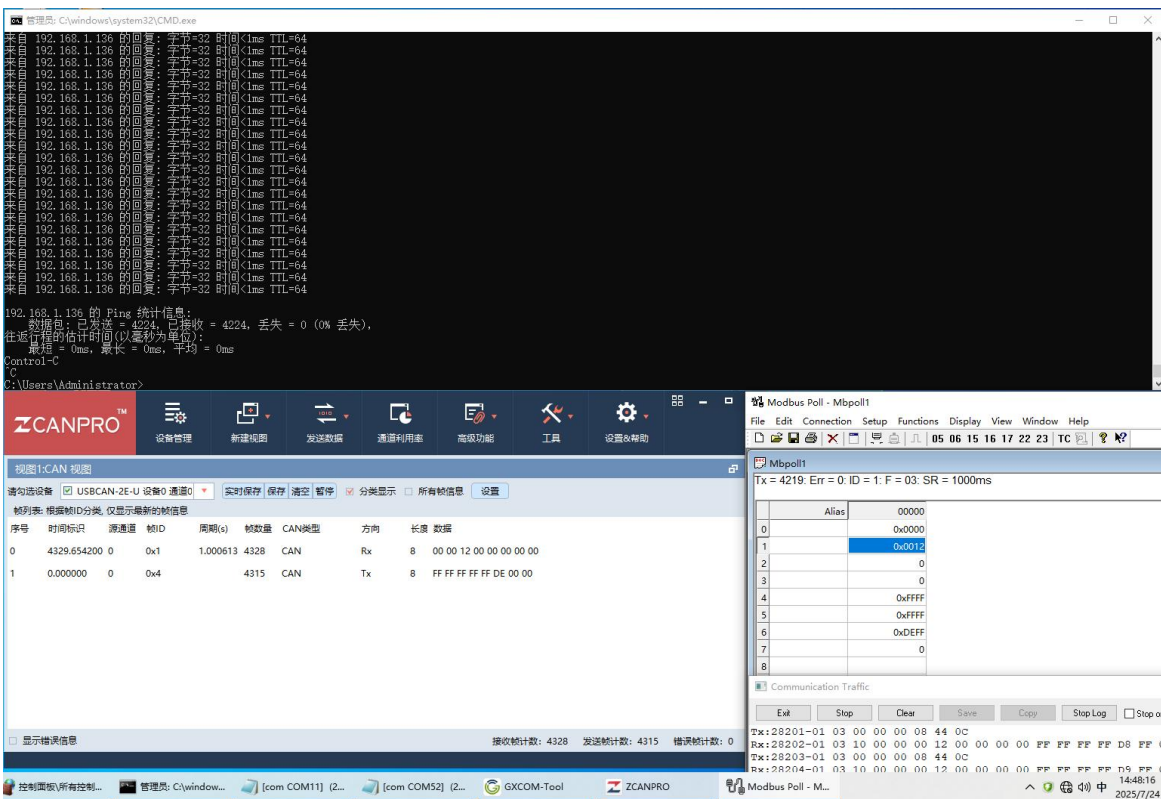
图 13 样机在低温试验第三次启动检查功能正常 (RTU 模式, 供电电压 36VDC)
