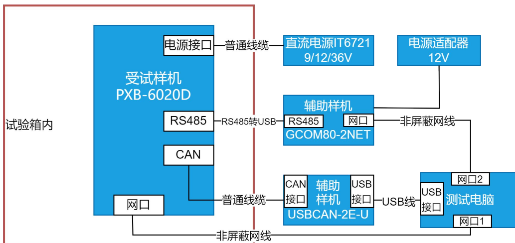
图 2 试验配置框图
