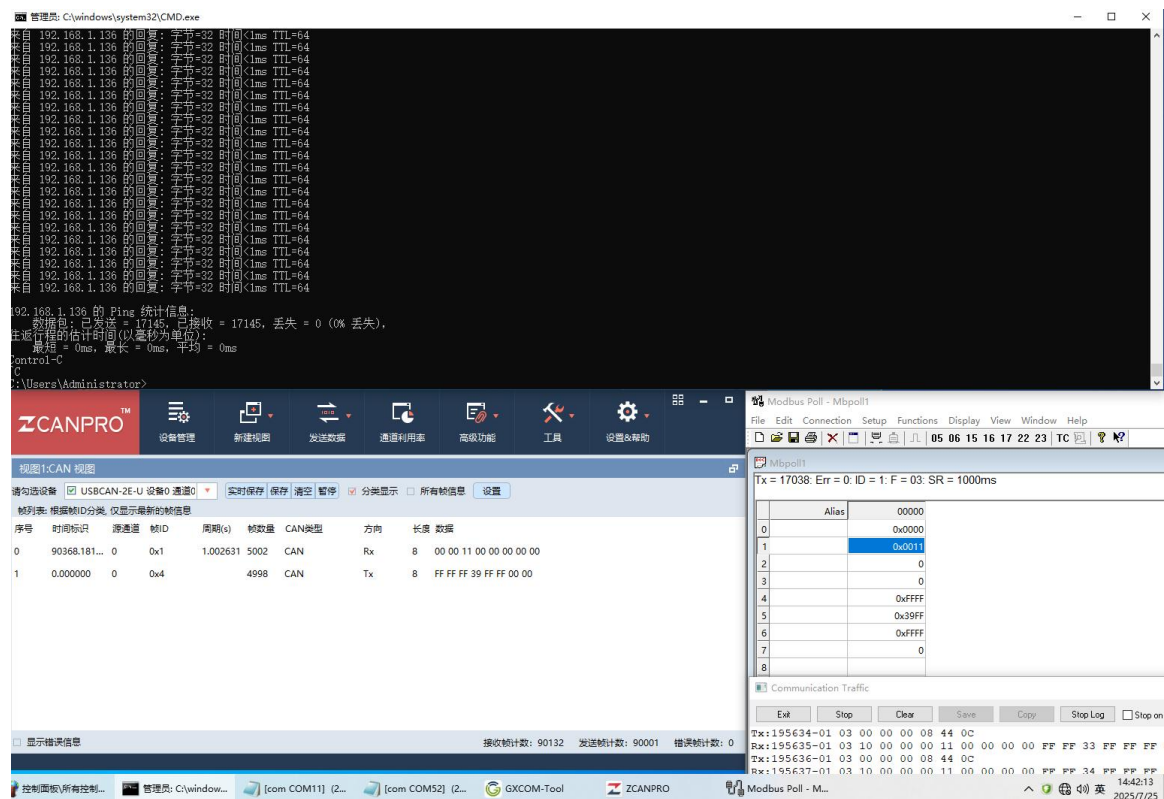
图 8 样机在高温试验第二次启动检查功能正常 (RTU 模式, 供电电压 12VDC)
