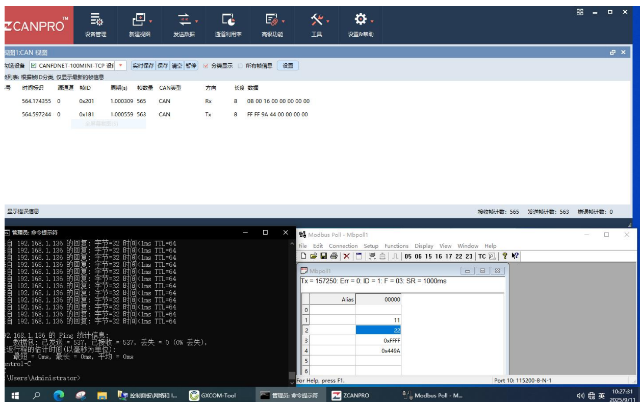
图 12 样机在恒定湿热试验时第三次启动运行检查功能正常（36VDC 供电）
