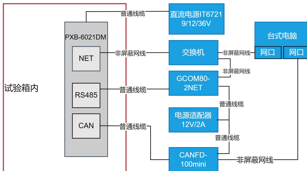
图 2 试验配置框图
