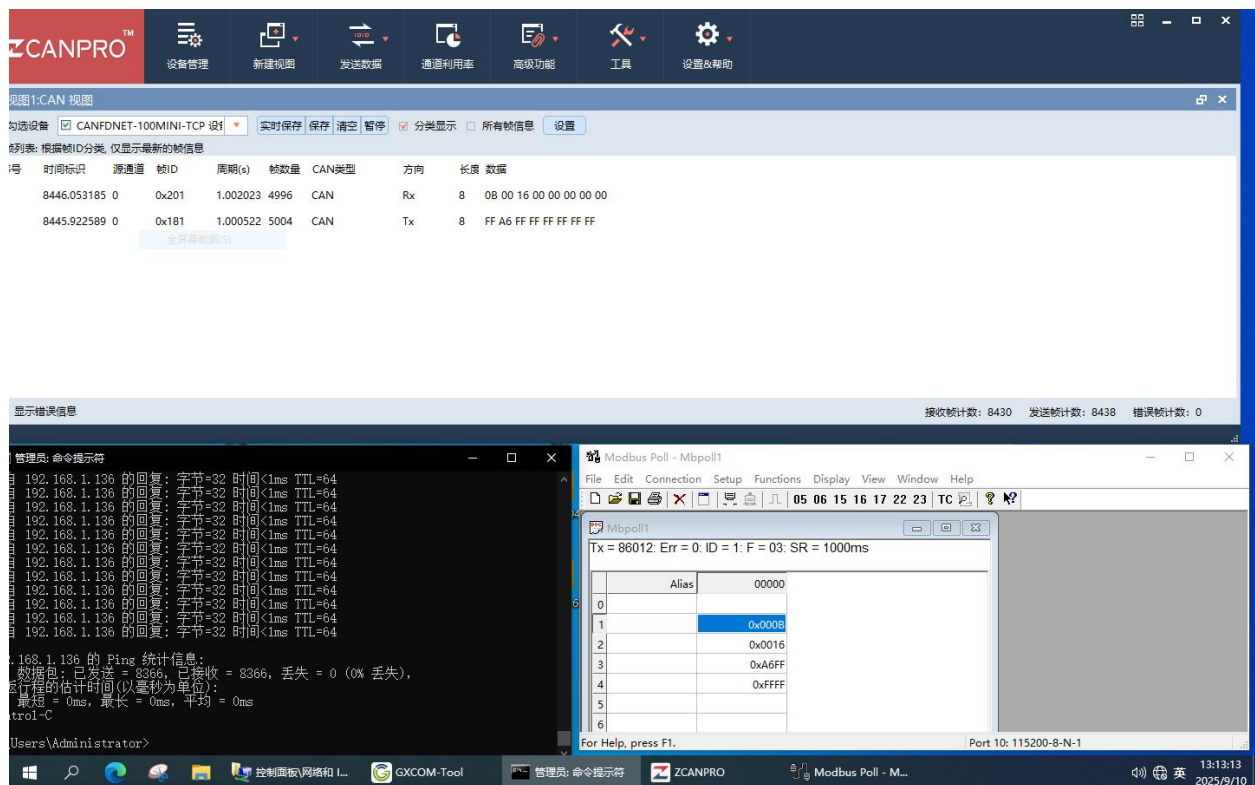
图 10 样机在低温试验时第一次启动运行检查功能正常（9VDC 供电）
