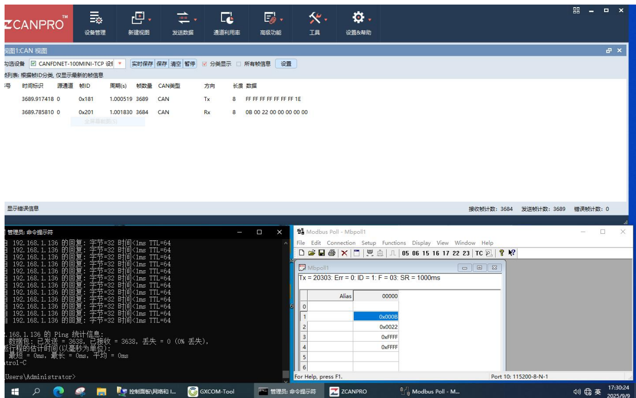
图 8 样机在高温试验时第三次启动运行检查功能正常（36VDC 供电）
