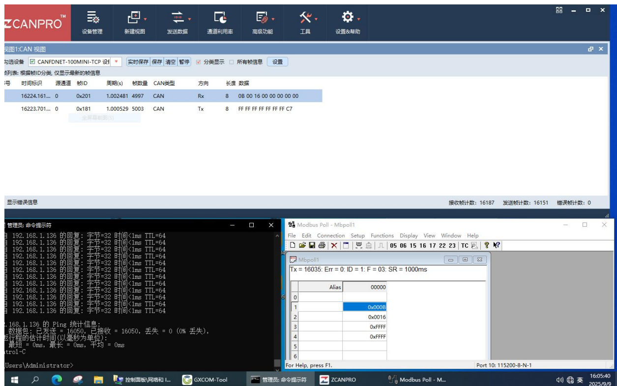
图 6 样机在高温试验时第一次启动运行检查功能正常（12VDC 供电）
