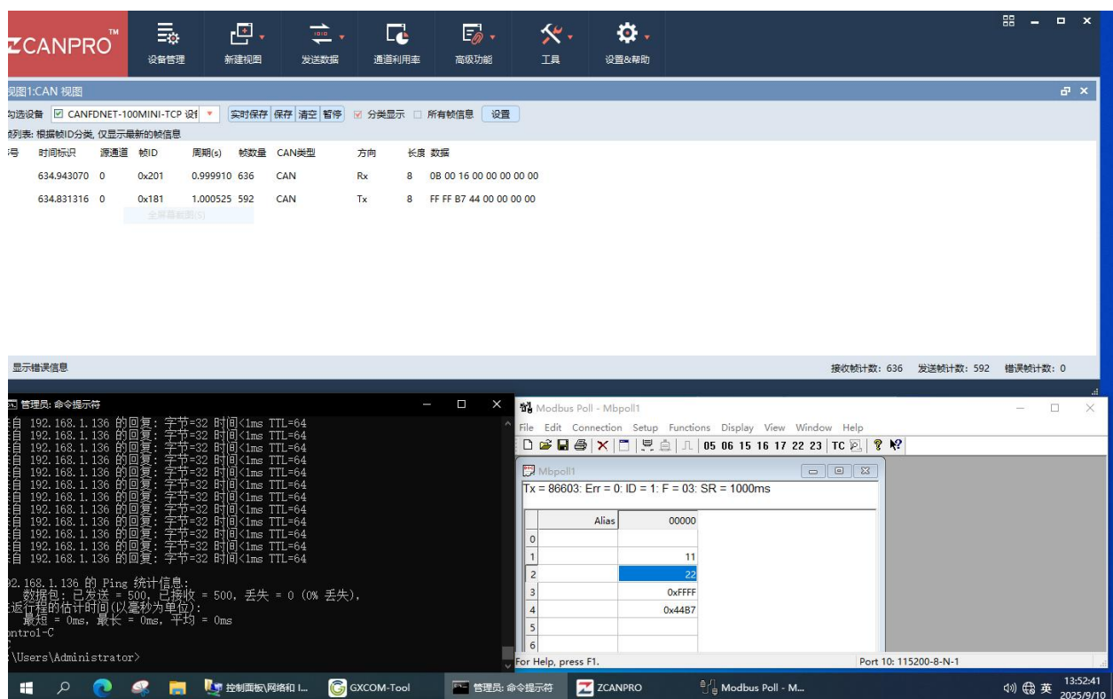
图 11 样机在低温试验时第二次启动运行检查功能正常（36VDC 供电）
