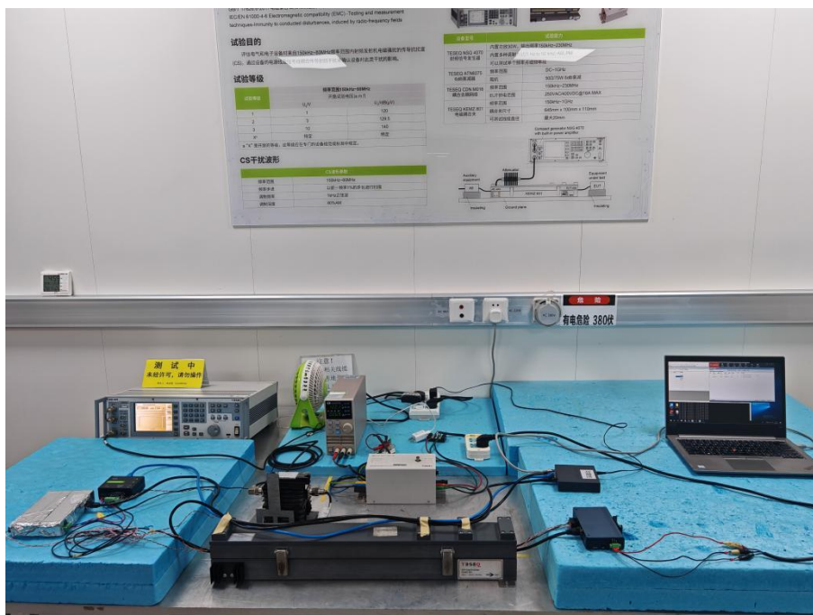
图 11 CS 试验现场配置图
