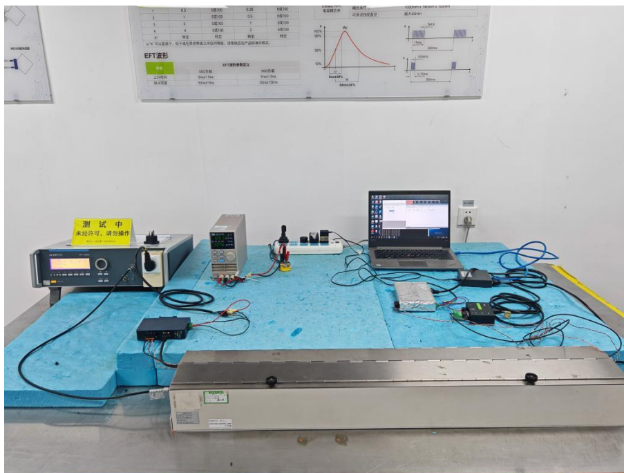
图 10 EFT 试验现场配置图
