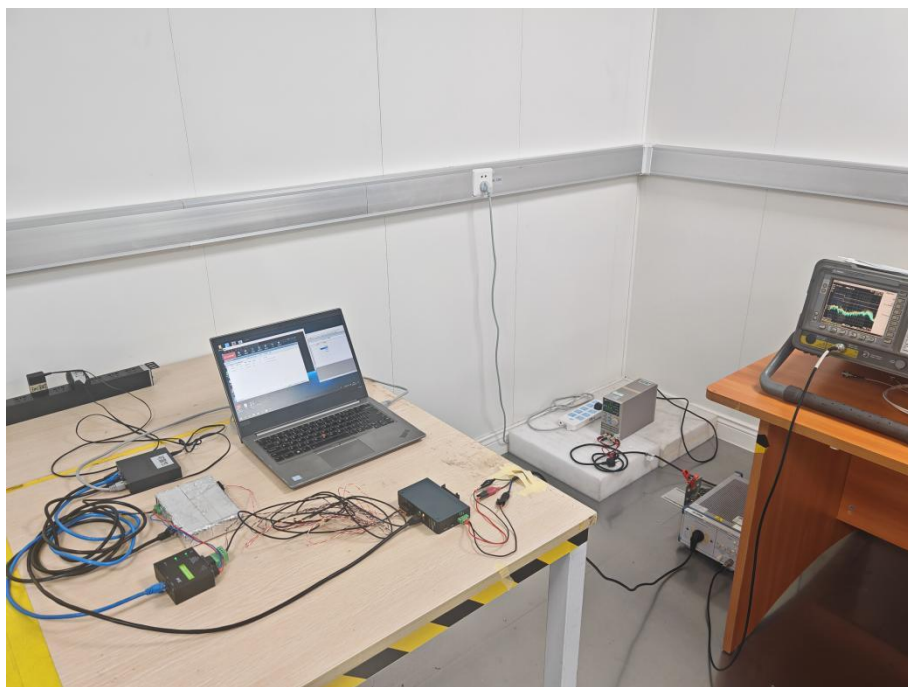
图 13 CE 试验现场配置图
