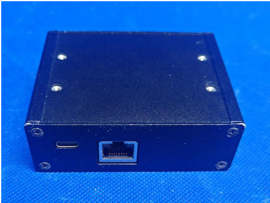
图 8 辅助样机 CANFDNET-100mini 后视图
