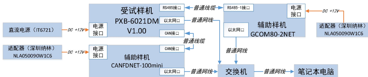
图 1 试验配置网络连接示意图
