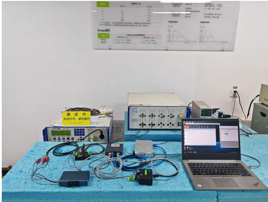
图 12 浪涌试验现场配置图
