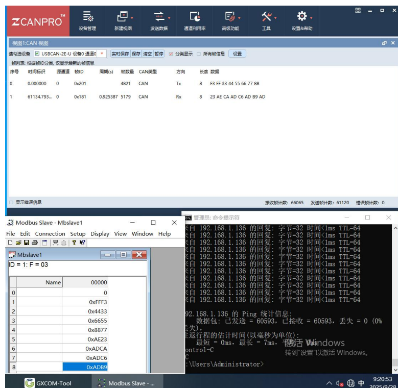
图 9 样机在温度变化试验时功能正常（12VDC 供电）
