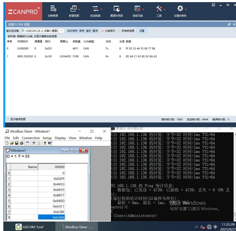
图 6 样机在高温试验时第一次启动运行检查功能正常（36VDC 供电）
