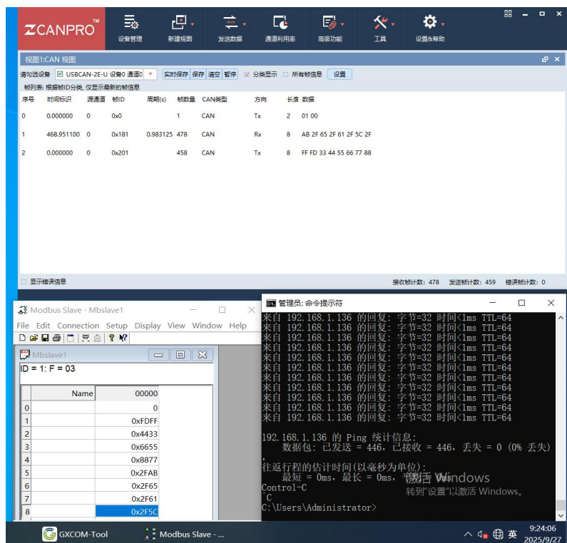
图 11 样机在恒定湿热试验时第二次启动运行检查功能正常（9VDC 供电）
