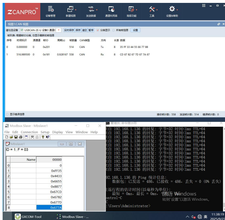
图 7 样机在高温试验时第二次启动运行检查功能正常（9VDC 供电）
