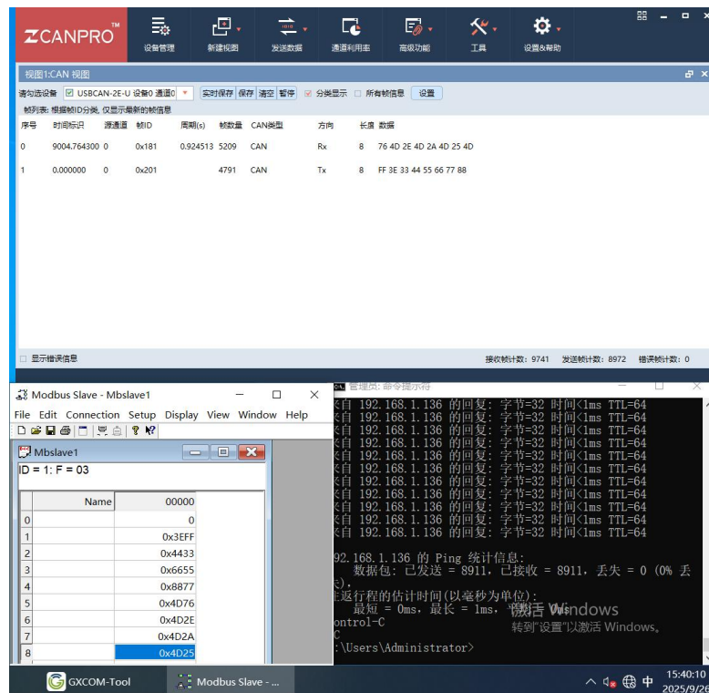
图 12 样机在低温试验时第三次启动运行检查功能正常（12VDC 供电）
