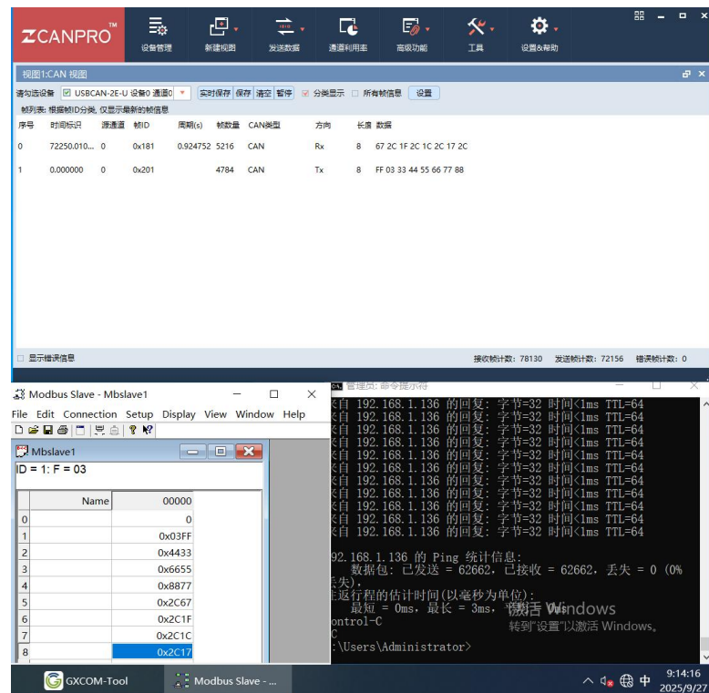
图 10 样机在恒定湿热试验时第一次启动运行检查功能正常（12VDC 供电）
