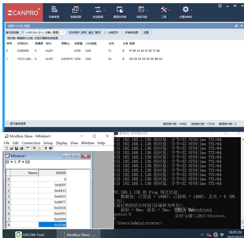
图 8 样机在高温试验时第三次启动运行检查功能正常（36VDC 供电）
