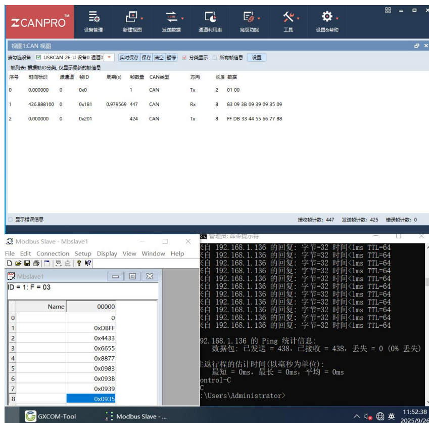
图 11 样机在低温试验时第二次启动运行检查功能正常(36VDC 供电)
