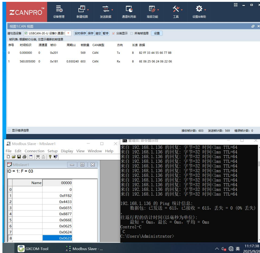
图 10 样机在低温试验时第一次启动运行检查功能正常(9VDC 供电)
