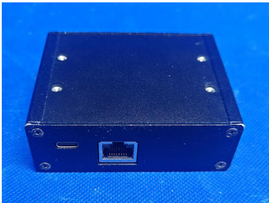
图 6 辅助样机 CANFDNET-100mini 后视图
