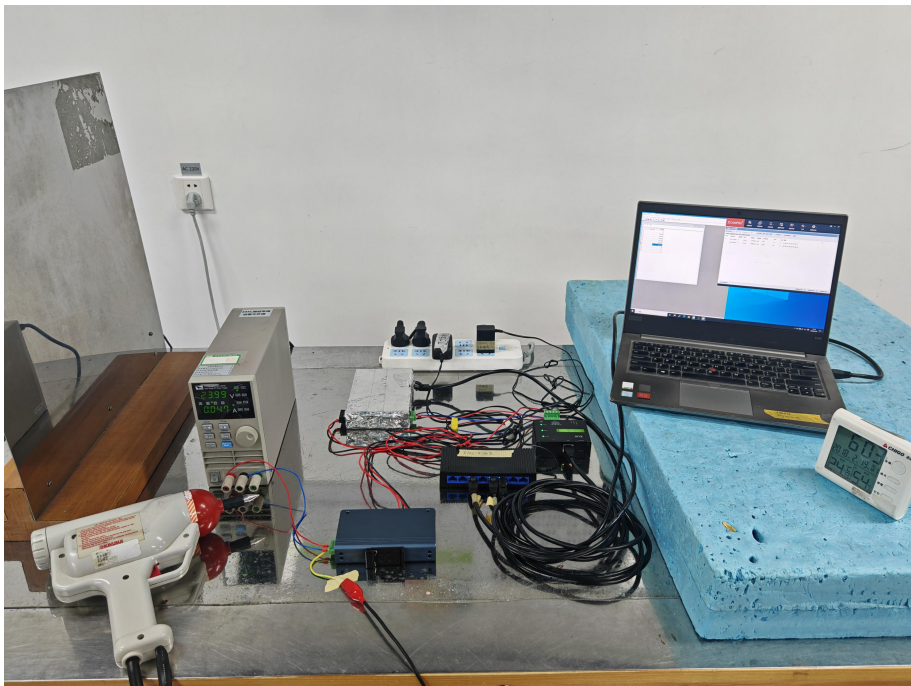
图 7 ESD 试验现场配置图
