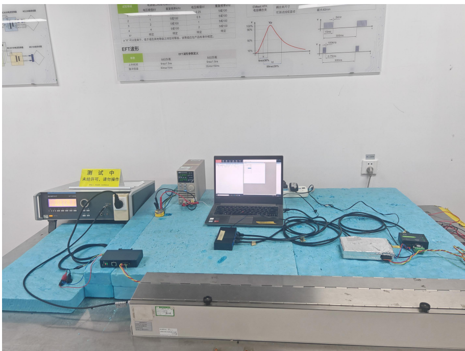
图 8 EFT 试验现场配置图
