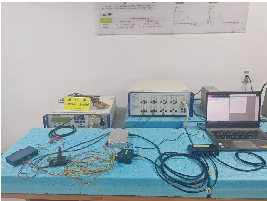
图 10 浪涌试验现场配置图
