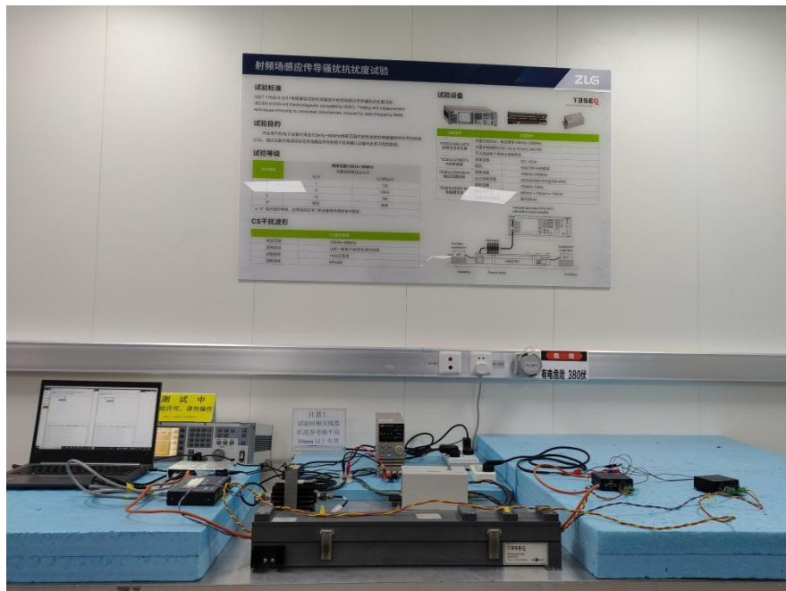
图 12 CS 试验配置
