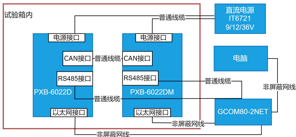
图 2 试验配置框图
