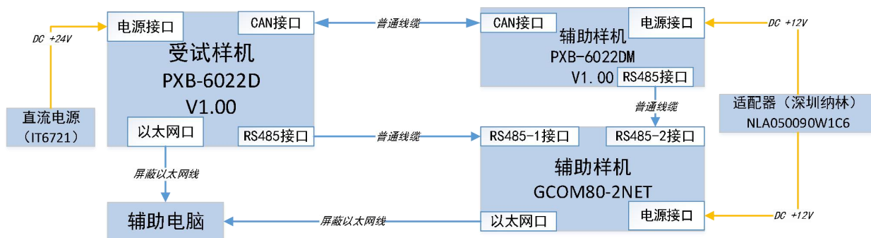
图 1 试验配置网络连接示意图
