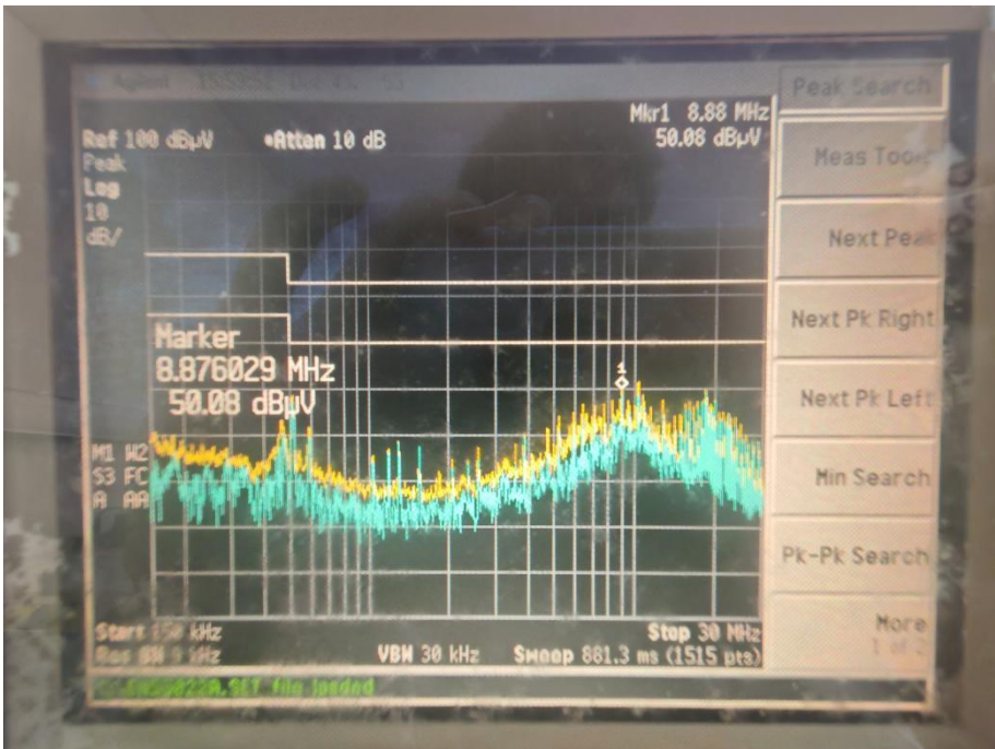
EUT-L/N 线 （Peak 曲线图）
