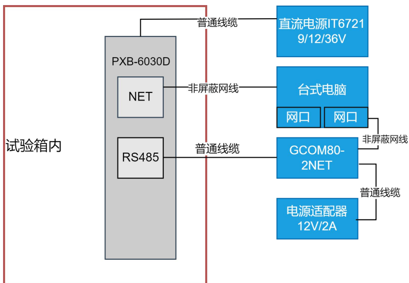
图 2 试验配置框图
