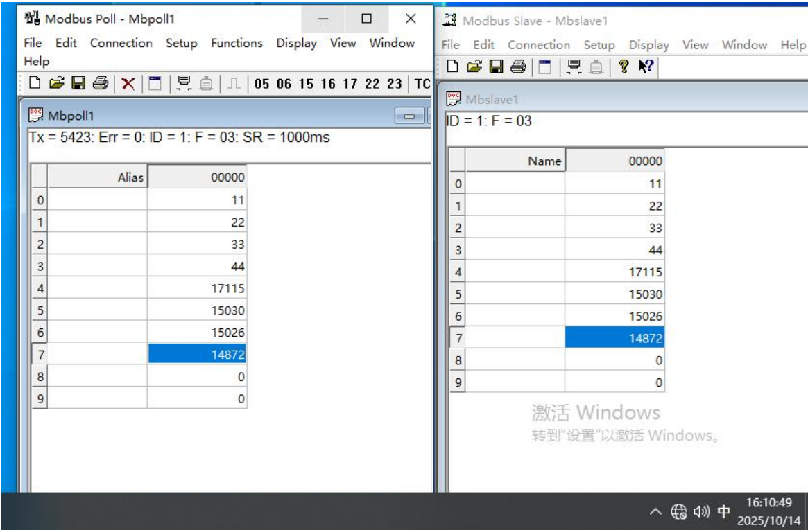
图 8 样机在高温试验时第三次启动运行检查功能正常（36VDC 供电）
