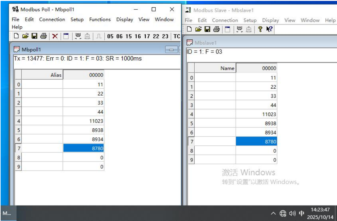
图 6 样机在高温试验时第一次启动运行检查功能正常（12VDC 供电）
