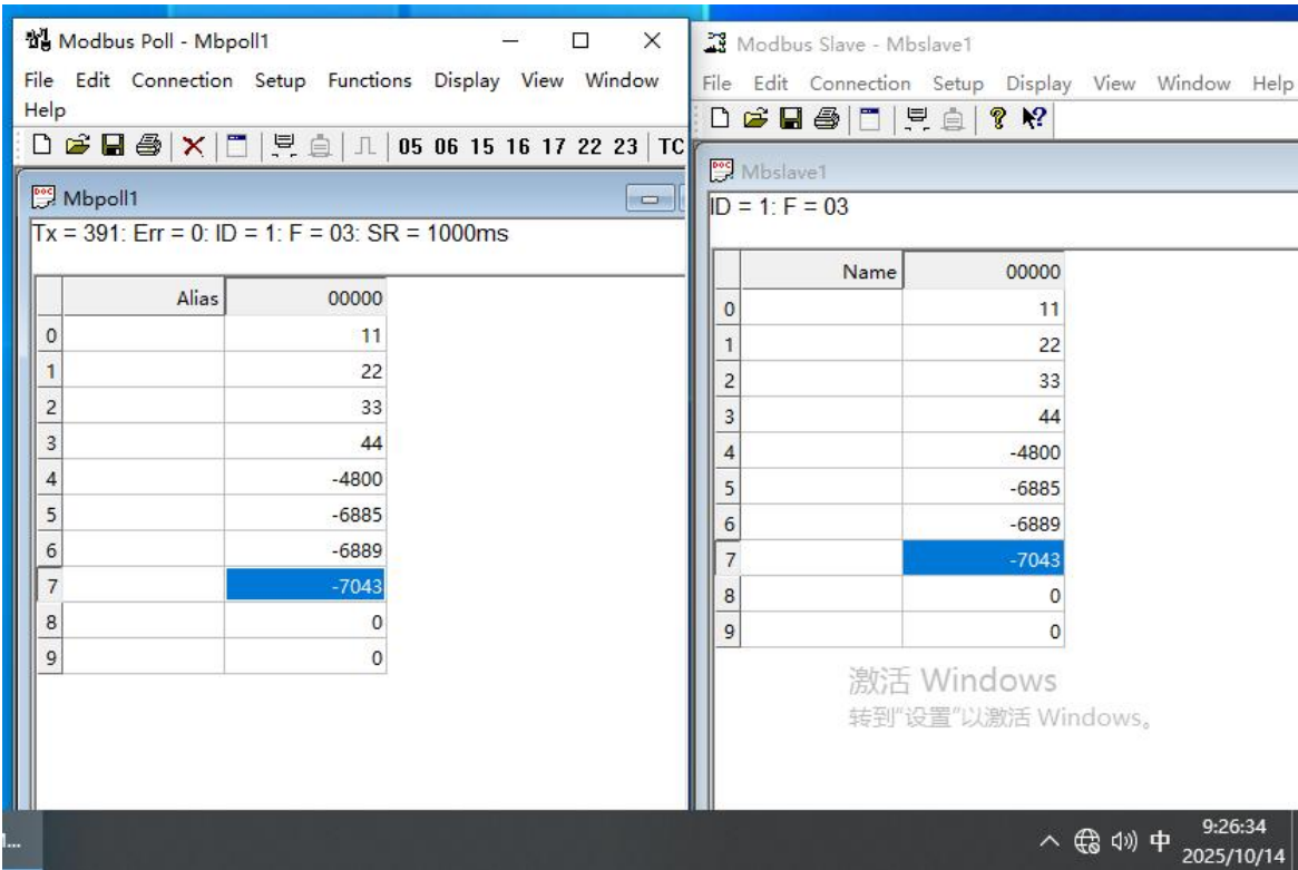
图 11 样机在恒定湿热试验时第二次启动运行检查功能正常（9VDC 供电）
