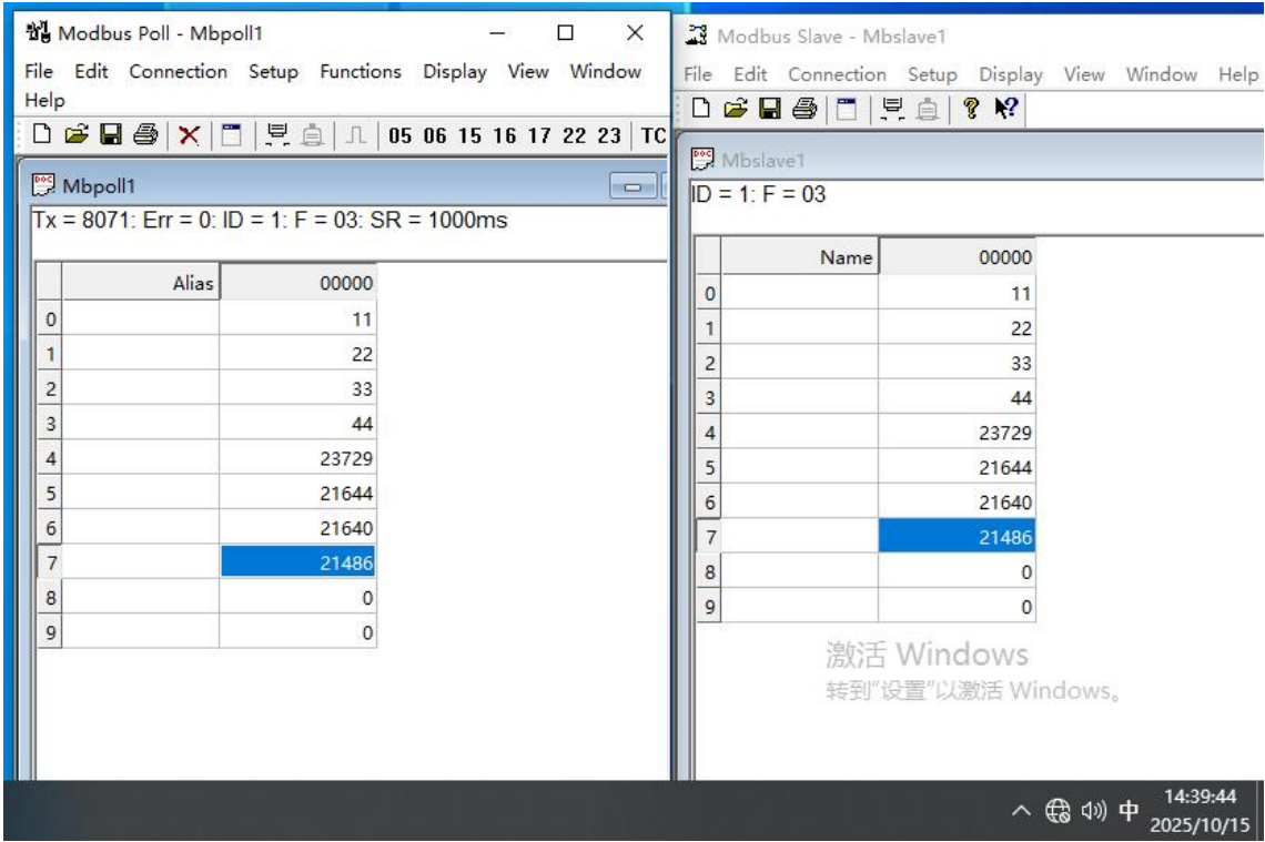
图 11 样机在低温试验时第二次启动运行检查功能正常（12VDC 供电）
