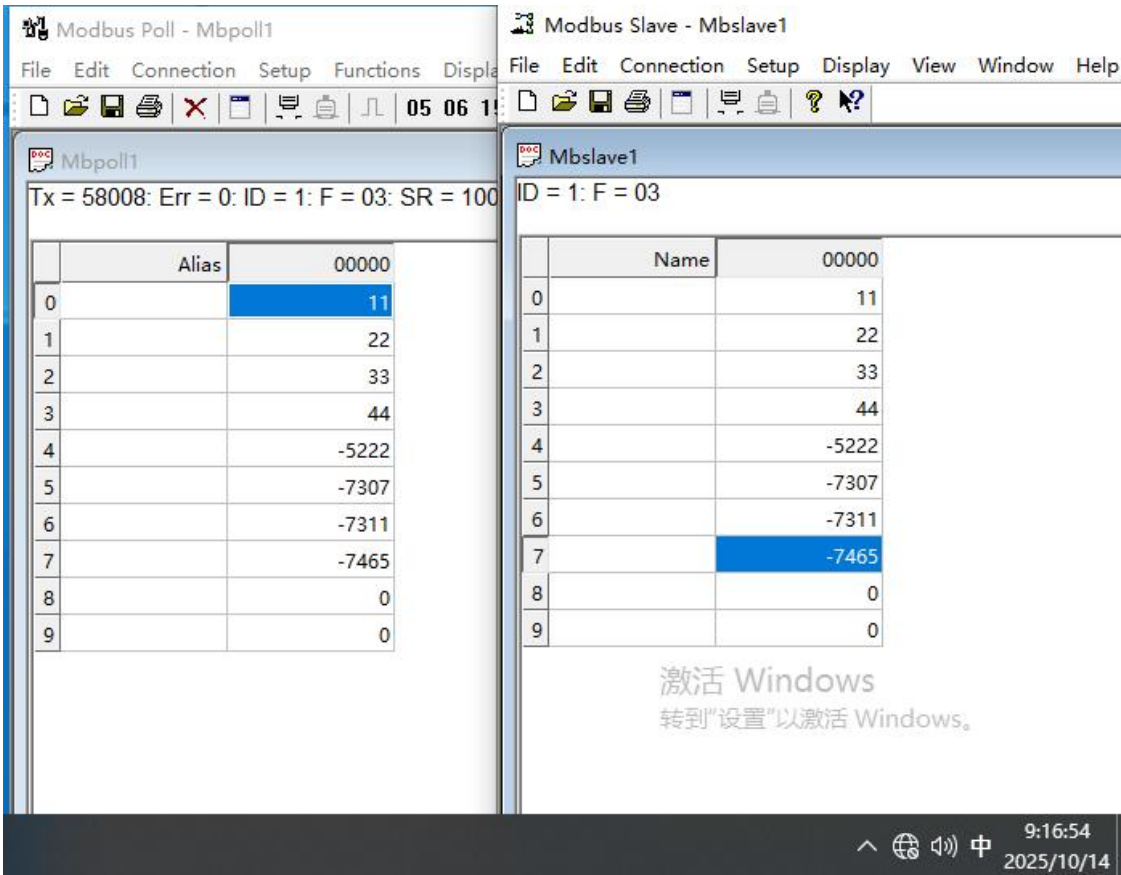
图 10 样机在恒定湿热试验时第一次启动运行检查功能正常（12VDC 供电）
