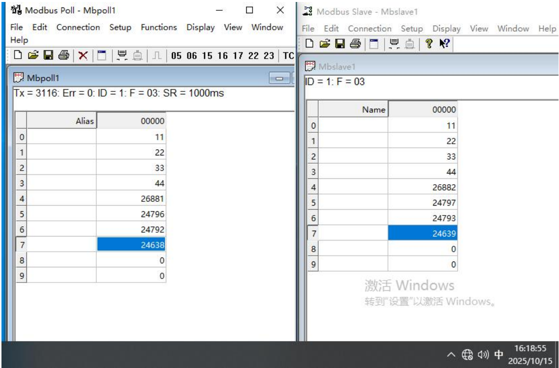
图 12 样机在低温试验时第三次启动运行检查功能正常（36VDC 供电）
