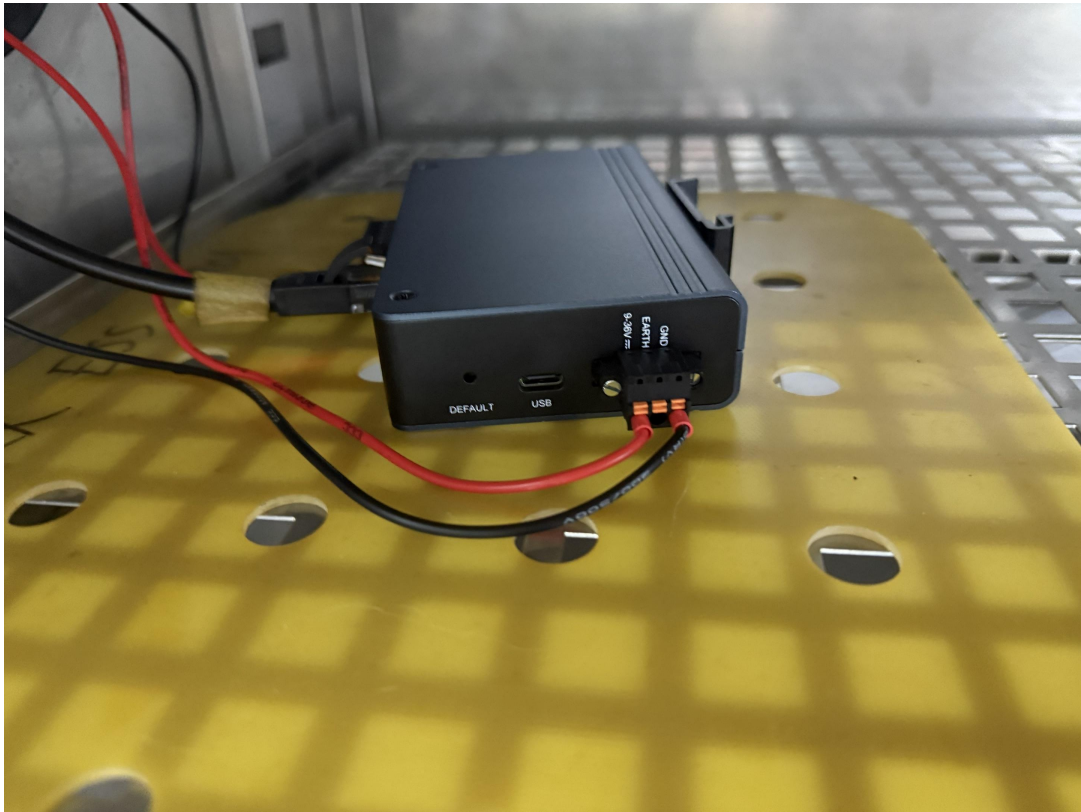
图 3 实际测试环境图
