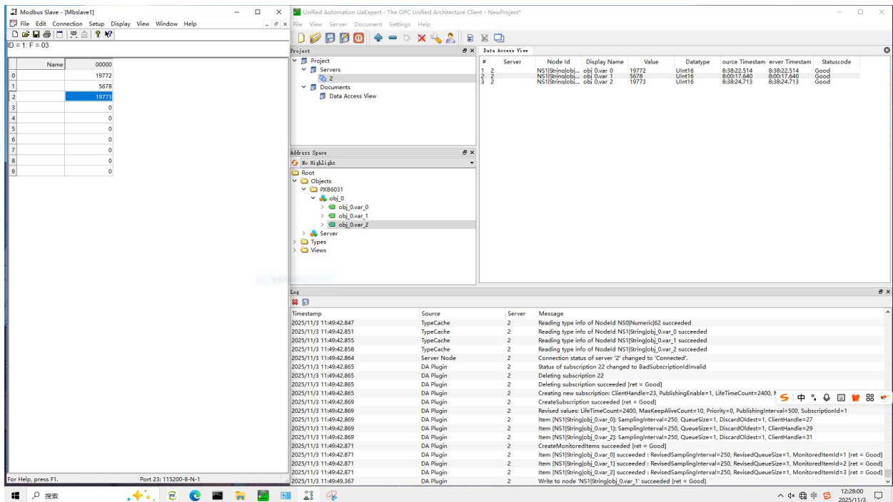
图 10 样机在低温试验时第一次启动运行检查功能正常（9VDC 供电）
