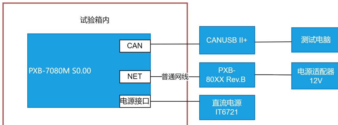
图 2 试验配置框图
