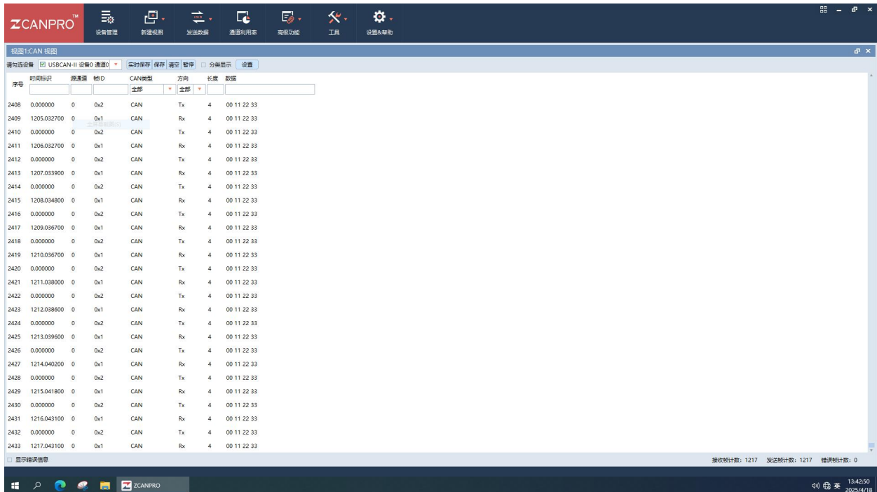
图 14 样机在低温试验时第三次启动运行检查功能正常（36VDC 供电）
