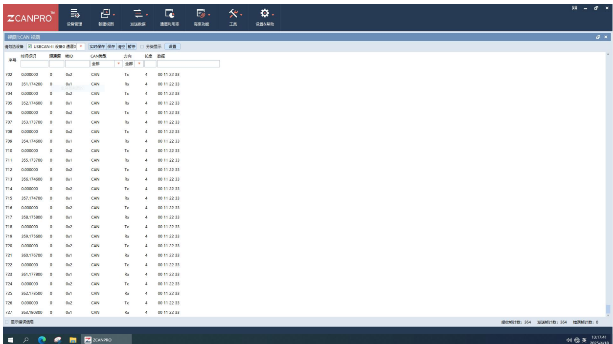
图 13 样机在低温试验时第二次启动运行检查功能正常（24VDC 供电）
