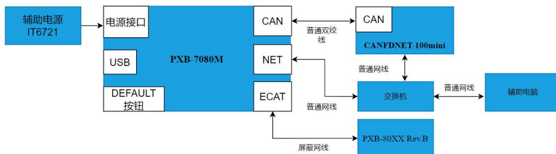
图 1 试验配置示意图
