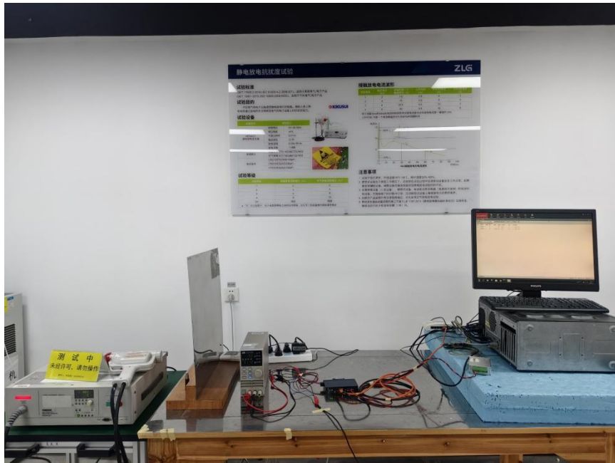
图 9 ESD 试验配置
