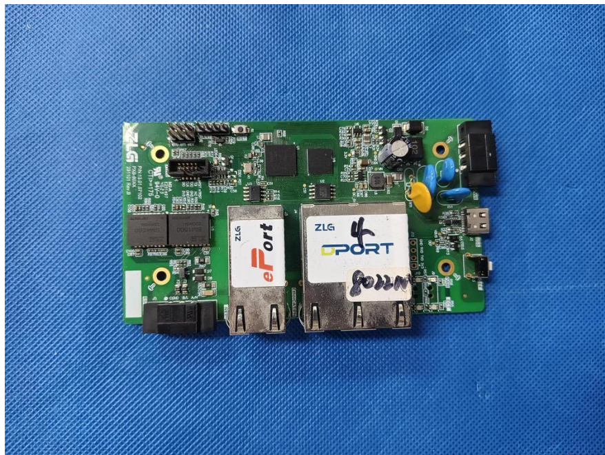
图 6 PXB-80XX Rev.B 正视图
