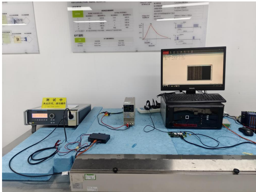
图 10 EFT/B 试验配置
