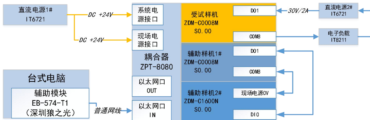
图 1 试验配置示意图
