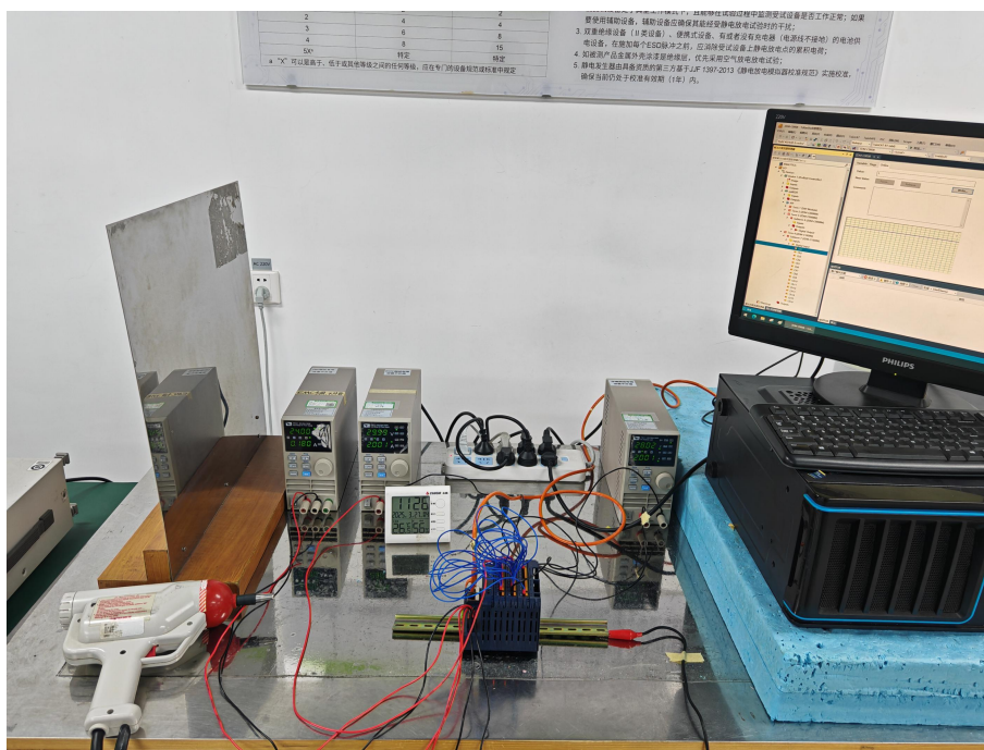
图 2 ESD 试验现场配置图
