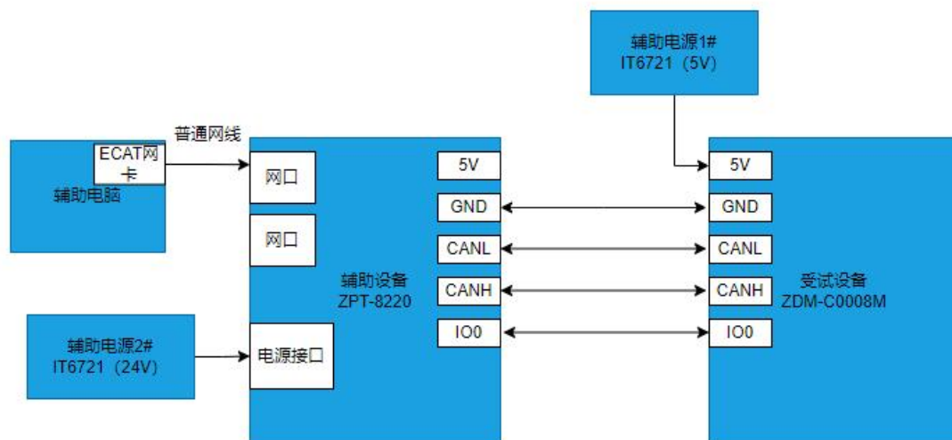
图1 试验配置图
