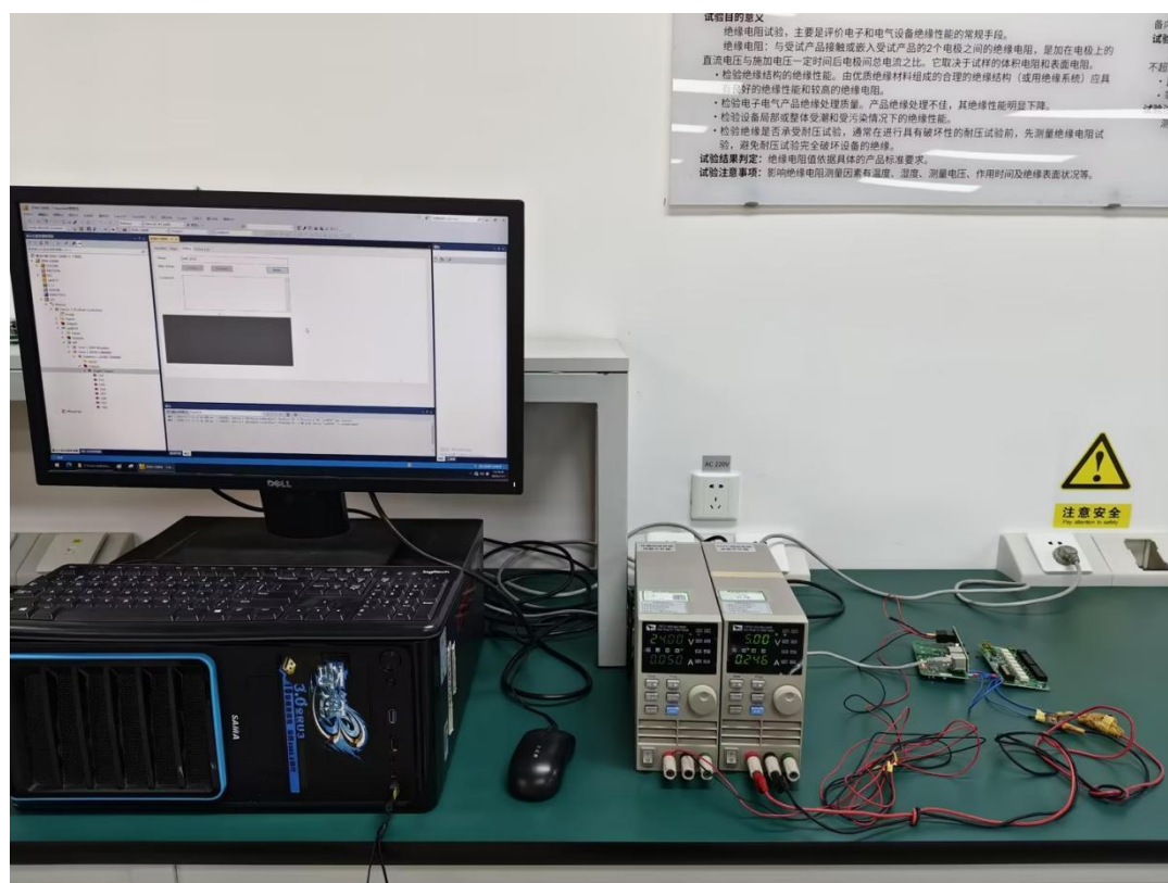
图1 试验配置图
