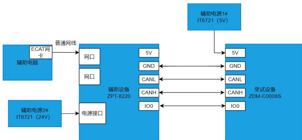
图1 试验配置图
