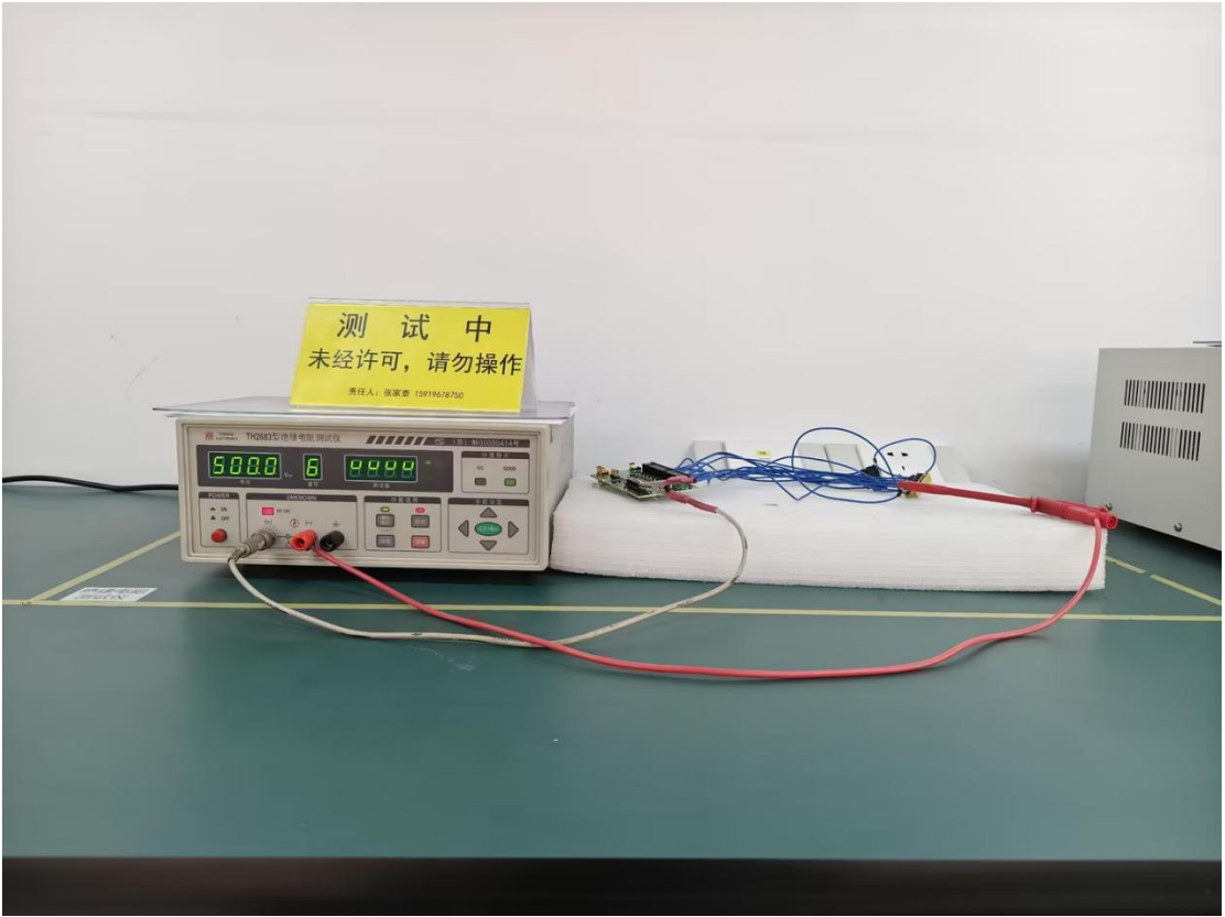
图 2 绝缘电阻试验
