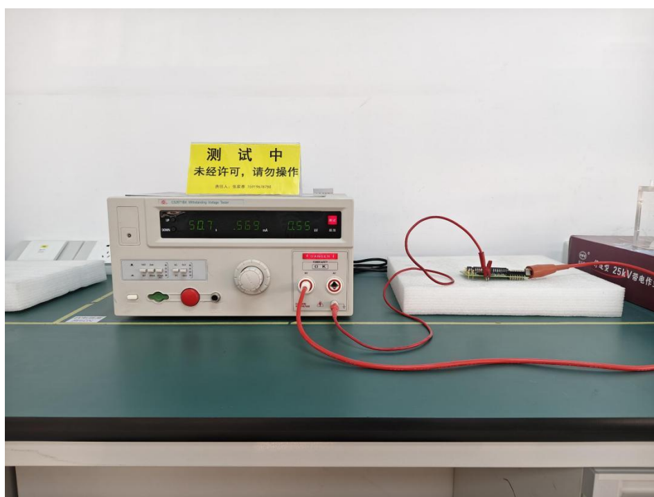
图 8 抗电强度试验
