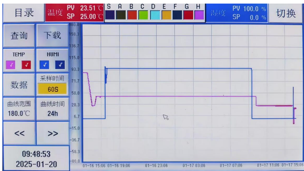
图 7 湿热处理曲线图
