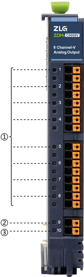
图 2.2 LED 指示灯标注
