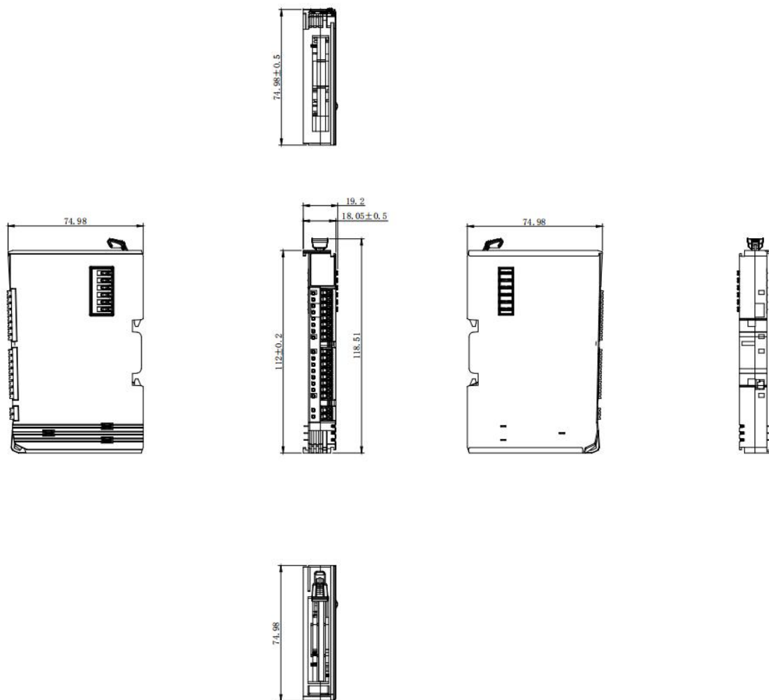
图 4.1 ZDM-C0008V 产品尺寸
