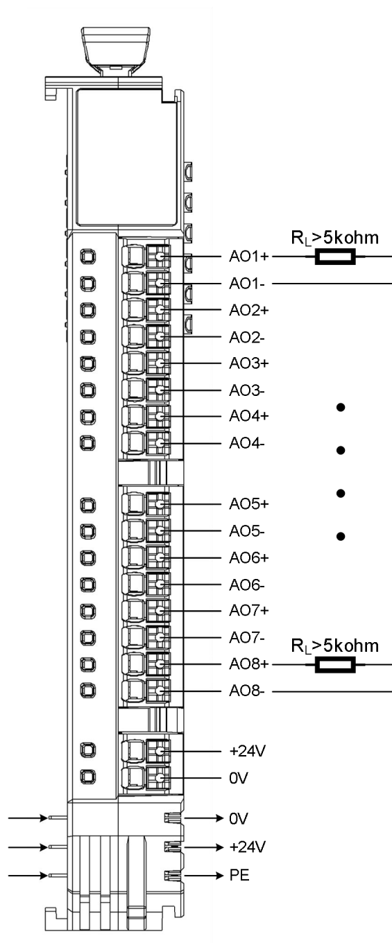
图 3.1 ZDM-C0008V 模块接线图
