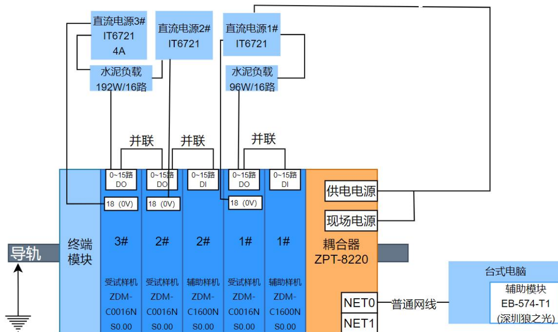
图 1 试验配置示意图
