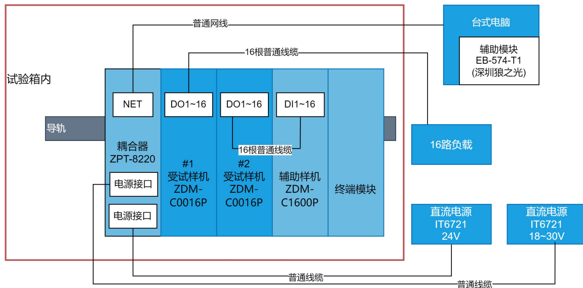
图 2 试验配置框图
