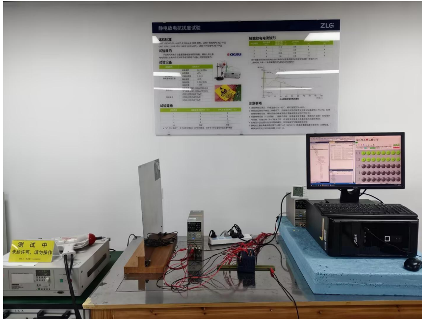
图 2 ESD 试验现场配置图
