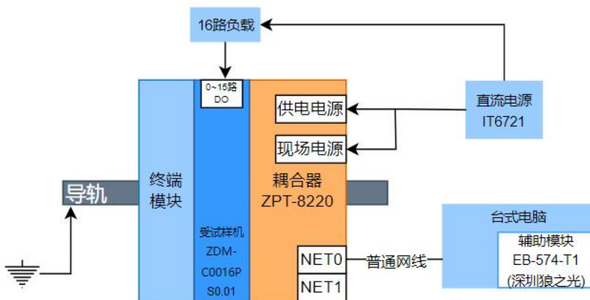
图 1 试验配置示意图
