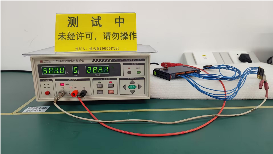
图 2 绝缘电阻试验
