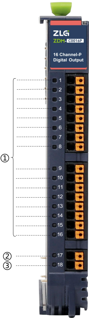
图 2.2 指示灯面板
