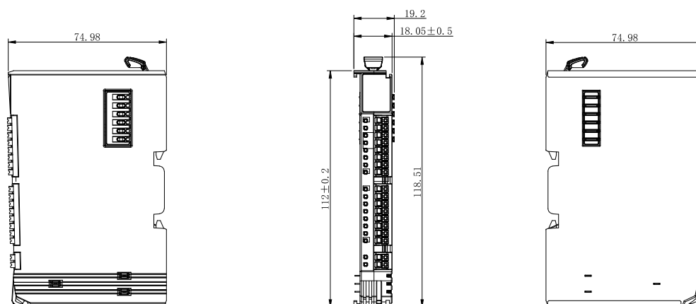
图 4.1 ZDM-C0016P 产品尺寸
